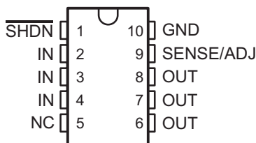
U 封装 (顶视图)
