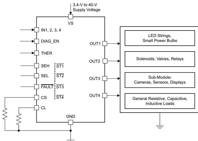
典型应用电路原理图
