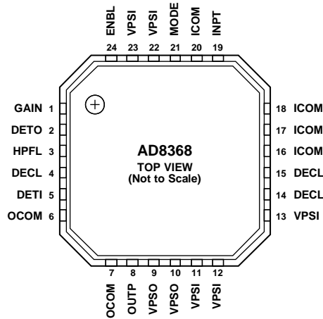
图2. 引脚配置
