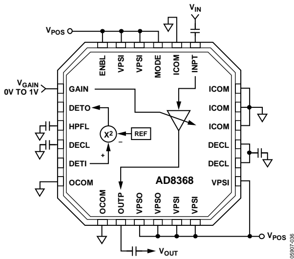
图33. VGA模式下，使增益随着 V_{GAIN} 的增加而增加的典型连接图(MODE高电平)
