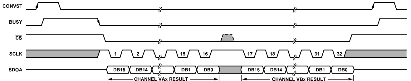
图58. 串行接口1线模式
