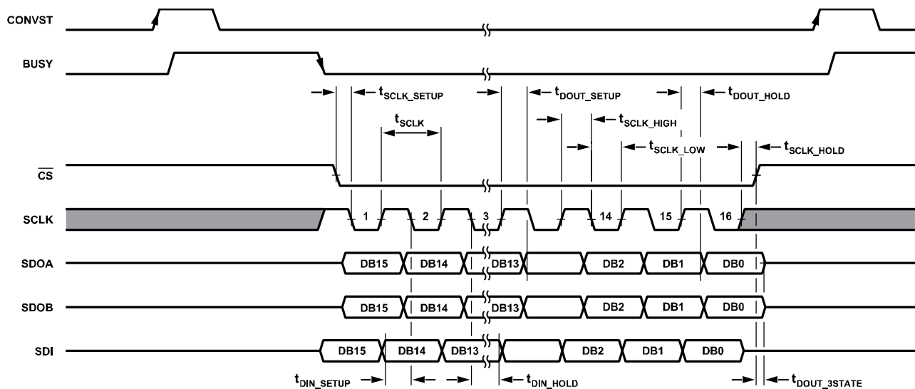
图6. 串行时序图
