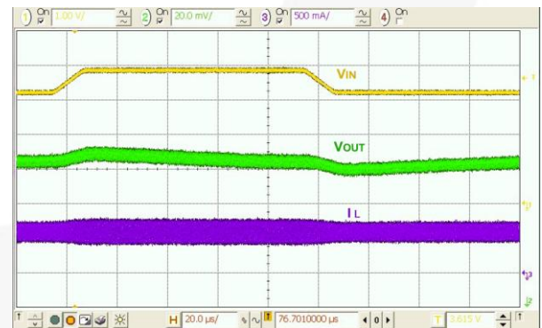
图 21. 线路瞬变, 3.3-3.9-3.3 V_{IN} , 10 \mu\text{s} 边沿, 600 mA 负载
