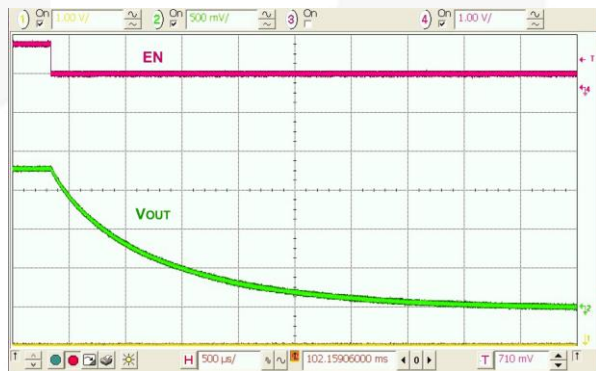
图 27. 关断, 无负载, 输出放电已启用
