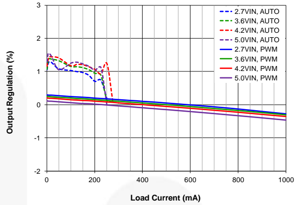
图 11. \Delta V_{OUT} (%) 与负载电流和输入电压的关系, V_{OUT} = 1.23\text{ V} , 标准化为 3.6\text{ V}_{IN} , 500\text{ mA} 负载, FPWM, 点线表示自动模式
