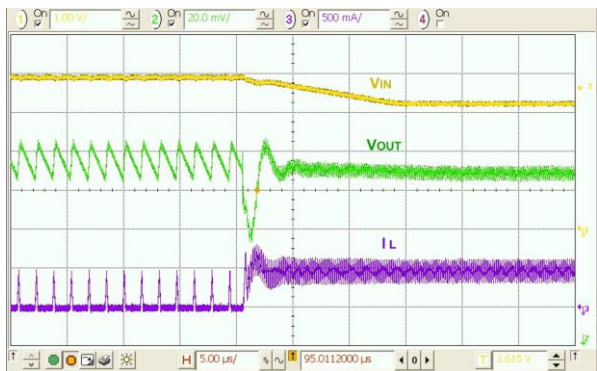
图 22. 组合线路/负载瞬态, 3.9-3.3 V_{IN} , 10 \mu\text{s} 边沿, 36-400 mA 负载, 100 ns 边沿
