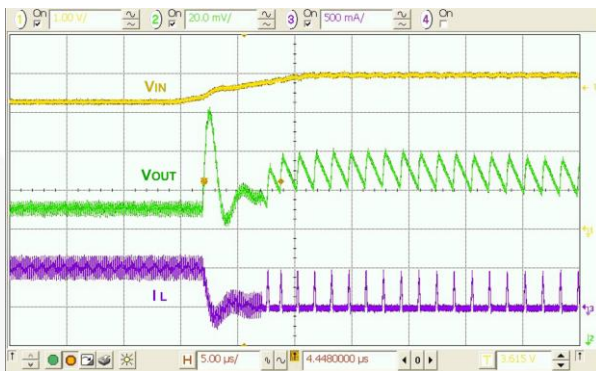
图 23. 组合线路/负载瞬态, 3.3-3.9 V_{IN} , 10 \mu\text{s} 边沿, 400-36 mA 负载, 100 ns 边沿
