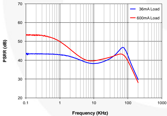
图 32. PSRR, 50 Ω 和 3 Ω 负载
