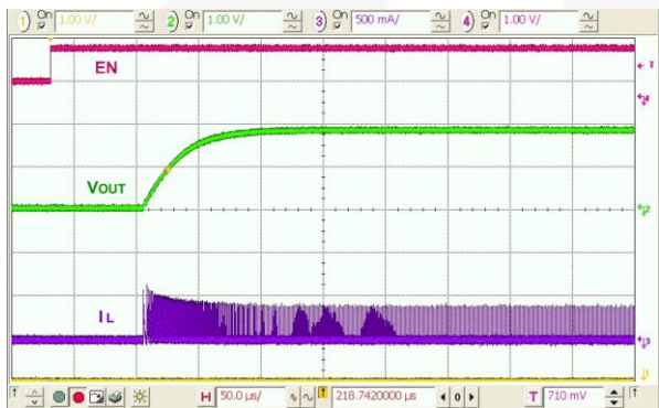
图 24. 启动, 50 \Omega 负载
