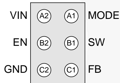
图 3. 焊球仰视图
