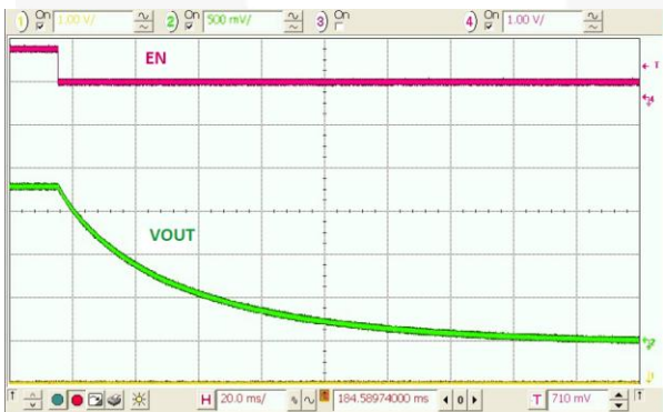
图 26. 关断, 10 k \Omega 负载, 无输出放电
