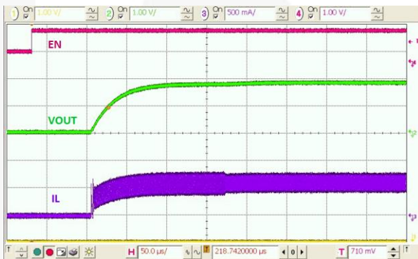
图 25. 启动, 3 \Omega 负载
