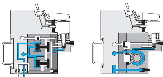
4/2 monostable module
