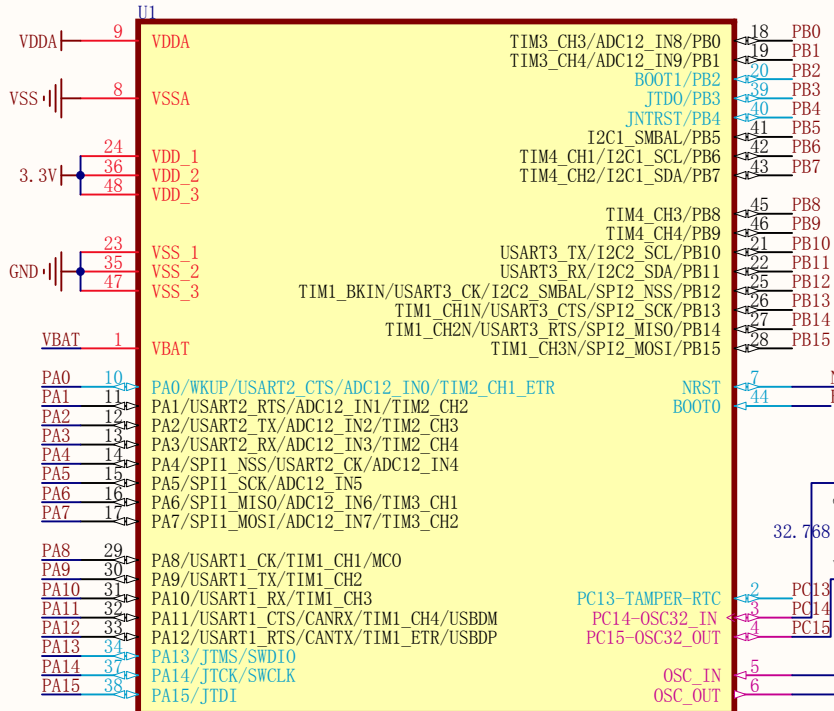
STM32F103C8T6最小系统板
