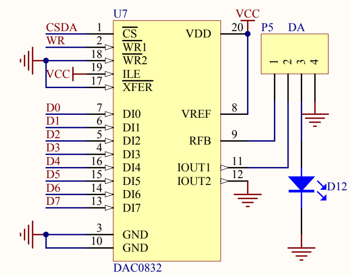
DAC0832电路
