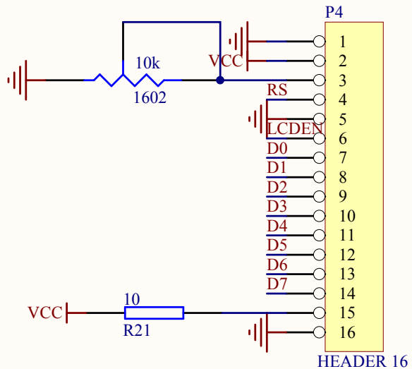
1602电路
