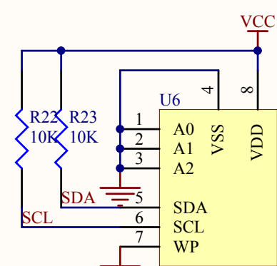
24C02电路
