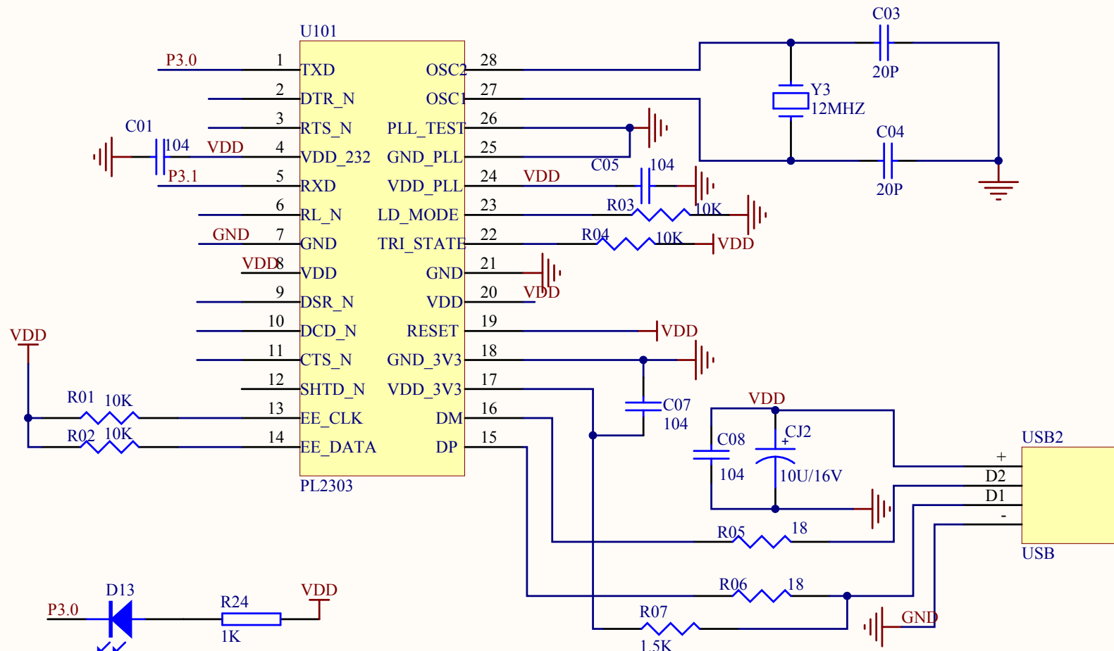
PL2303电路
