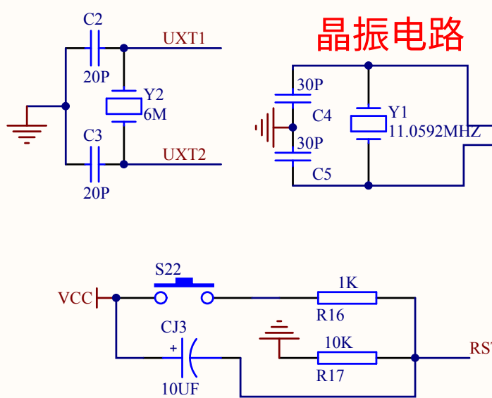
单片机复位电路
