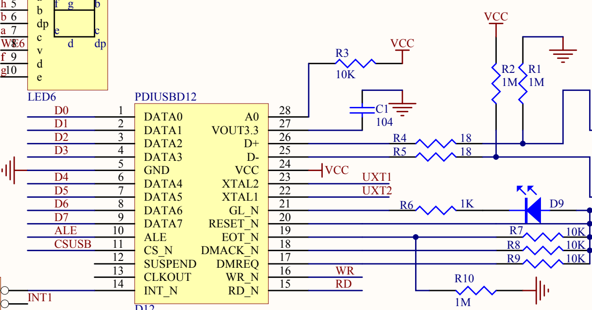
PDIUSBD12电路
