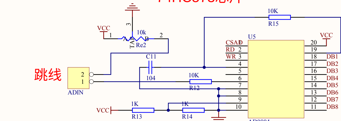
AD0804电路
