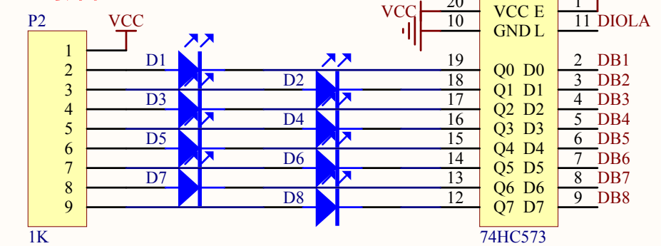
74HC573芯片
