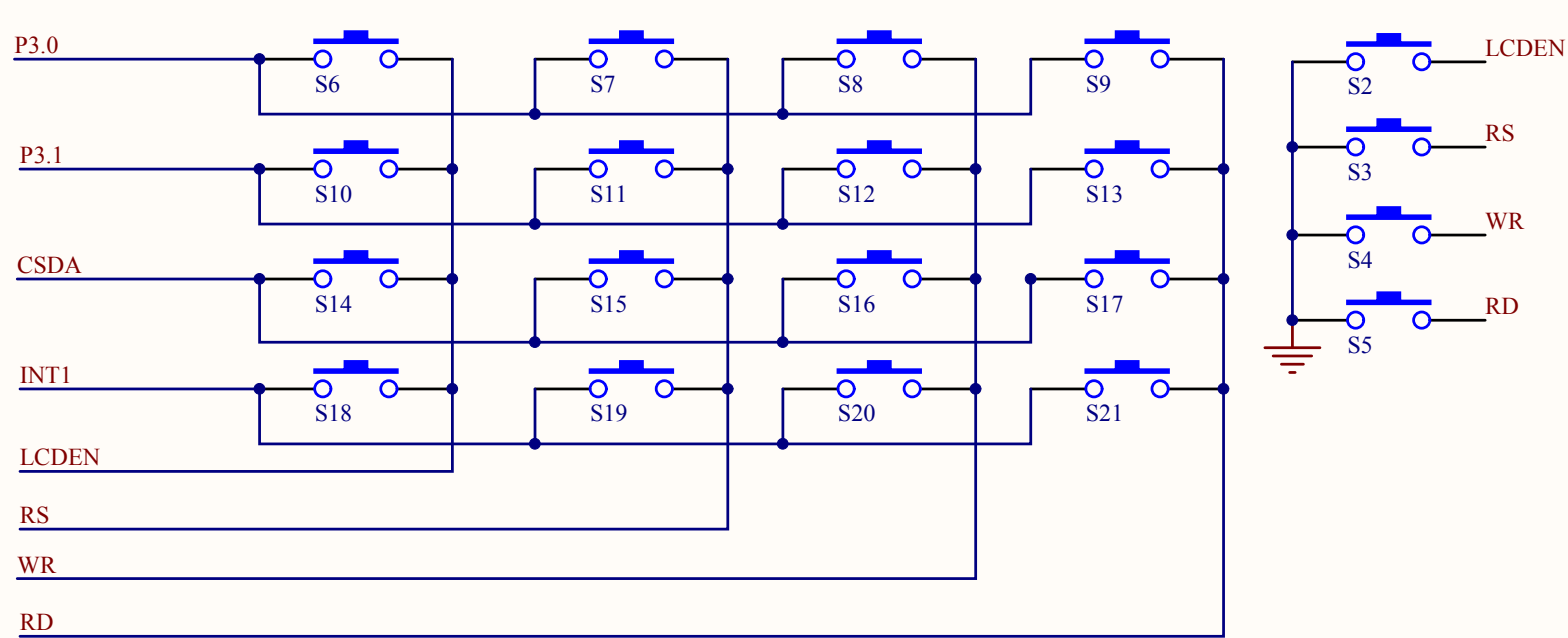
矩阵键盘电路
