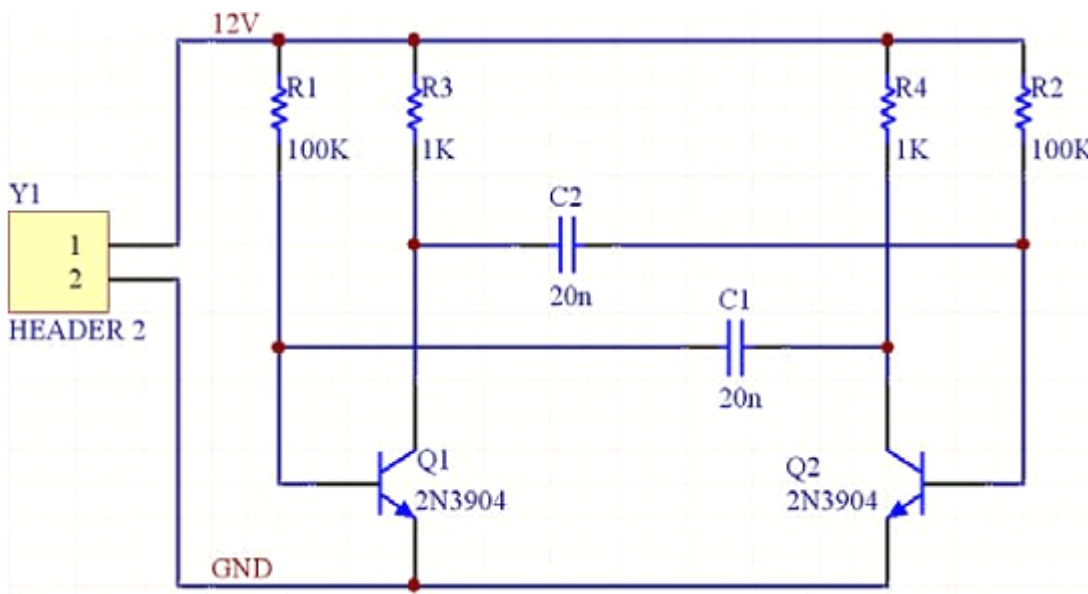
图6-8 完成布线的原理图
