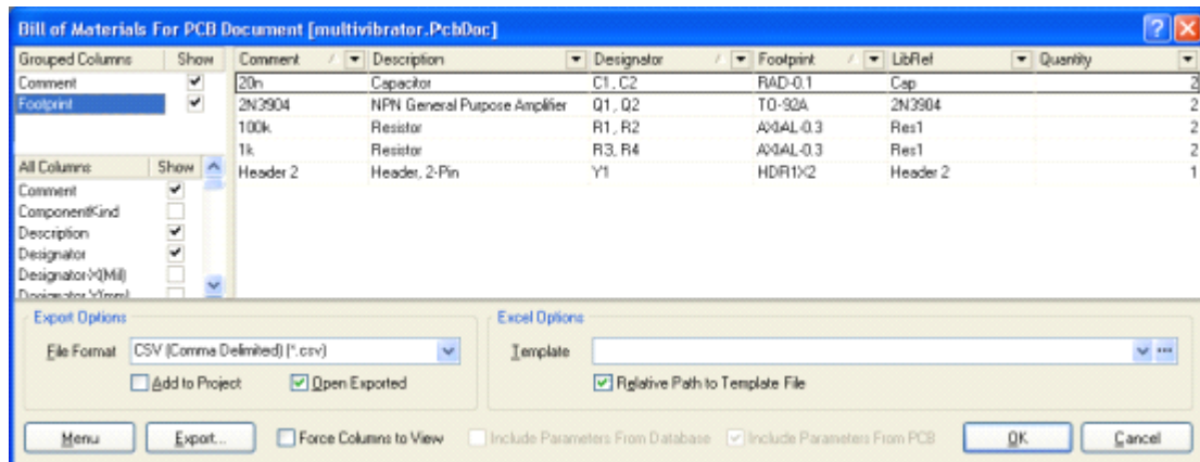
图6-37 器件清单
