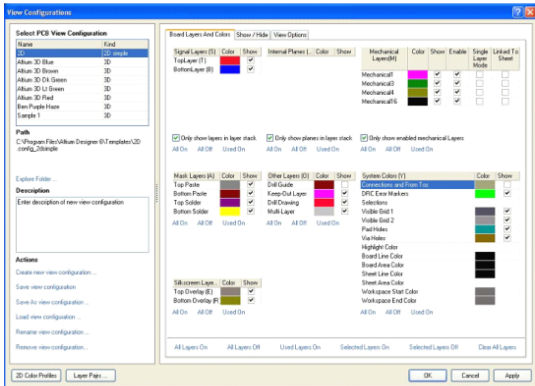
图6-17视图设置
