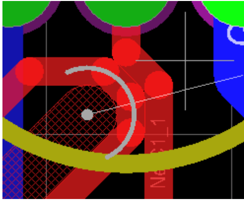
图6-28 双层手动布线?使用 Shift +SPACEBAR 来选择各种线的角度模式。角度模式包括：任意角度， 45^\circ ，弧度 45^\circ ， 90^\circ 和弧度 90^\circ 。按空格键切换角度。
