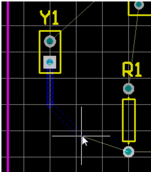
图6-26 手动布线检查文档工作区底部的层标签。Top Layer 标签当前应该是激活的。通过按下*键，来在不退出走线模式的情况下切换到底层。此键在可用信号层中循环。
