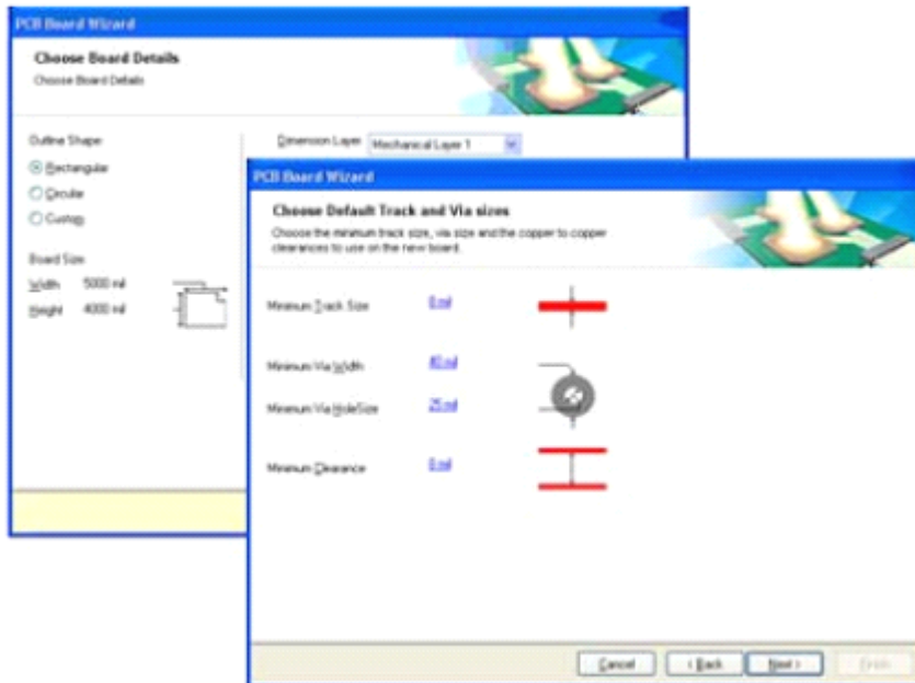
图6-12 PCB 板向导
