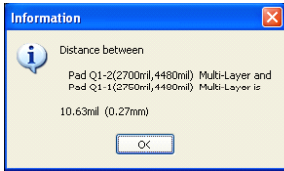
图6-34错误信息
