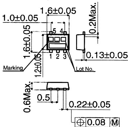
VSO5 (UNIT:mm)
