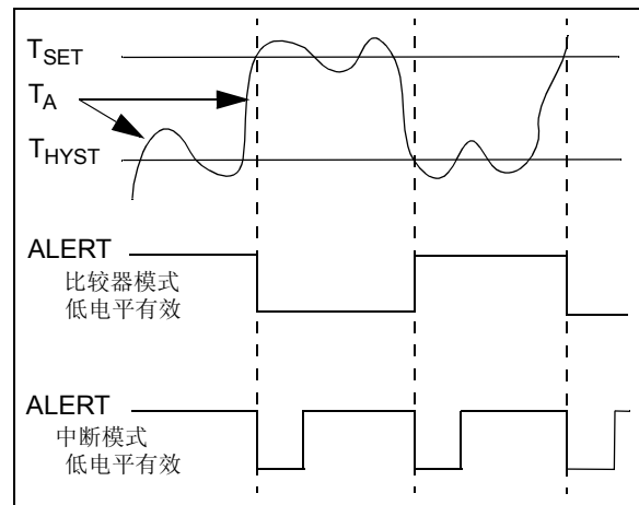
图 4-2: 报警输出
