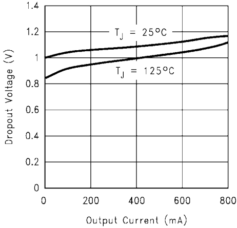
压差 ( V_{IN}-V_{OUT} )
