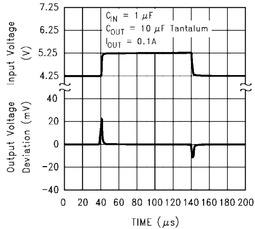
LM1117-2.85 线路负载瞬态响应
