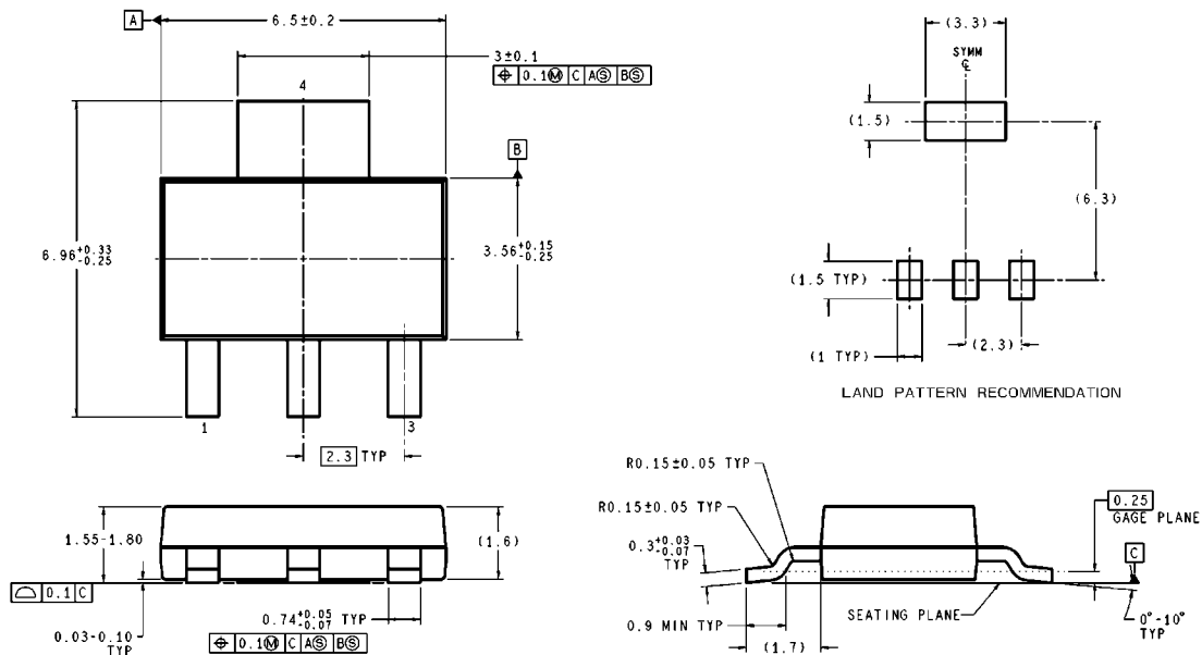
SOT-223 封装
