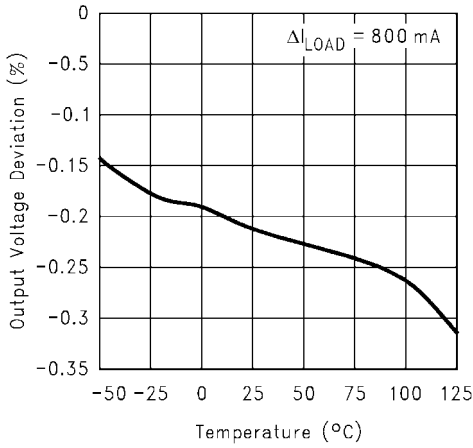
负载调整率
