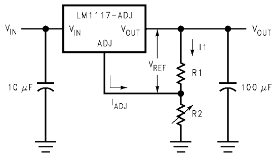
图 1 基本调压器
