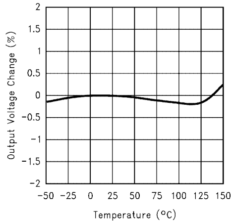
温度稳定性
