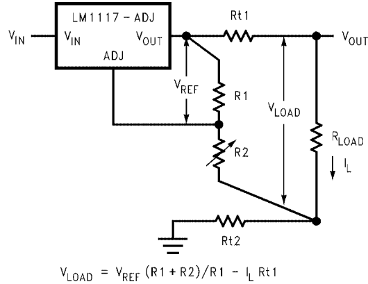
图 3 可调压输出的最佳负载调整
