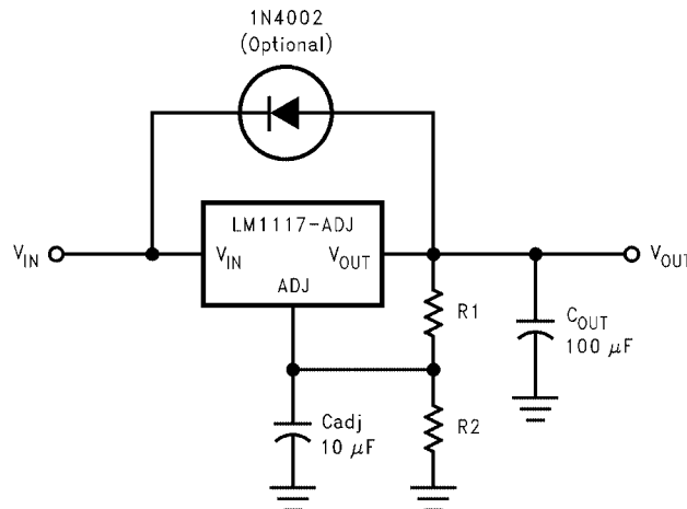
图 4 带保护二极管的调压器
