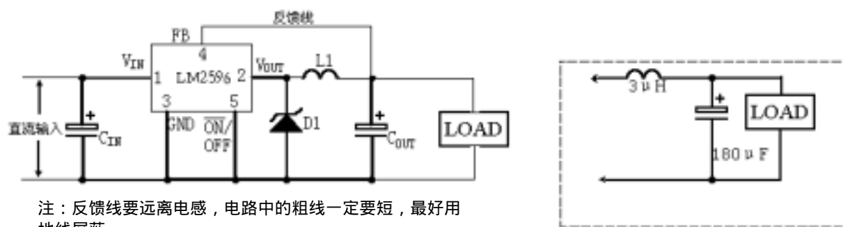
纹波滤波电路
