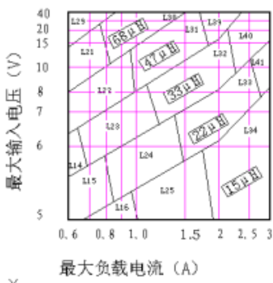
图 4 LM2596 —3.3
