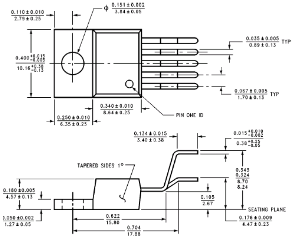
TO-220 封装 (T) 尺寸图 单位：英寸/毫米
