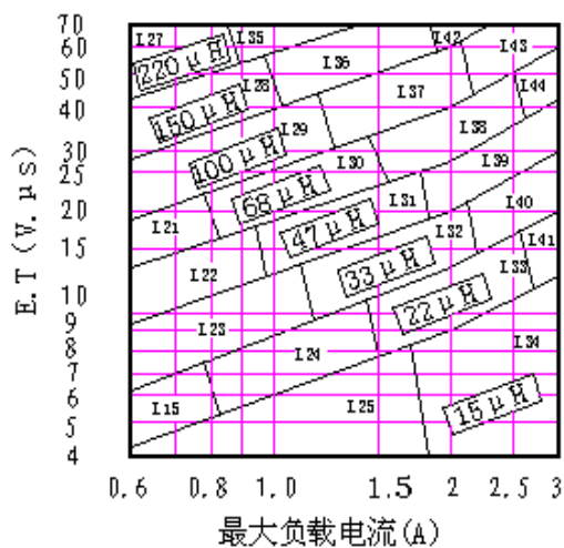
图 7 LM2596 —ADJ
