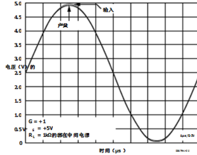
图5. 轨到轨响应
