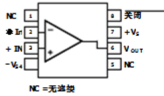
图1. SOIC-8 (R) 的
