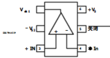
图2. 采用SC70-6 (KS)
