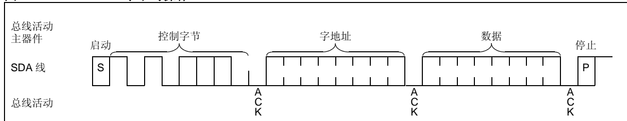
图 6-1: 字节写操作
