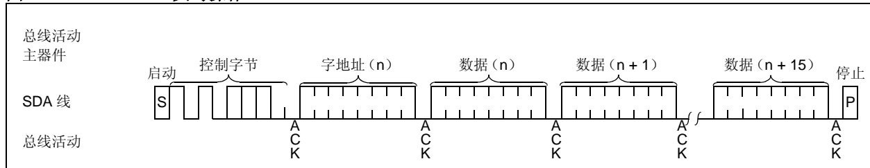
图 6-2: 页写操作
