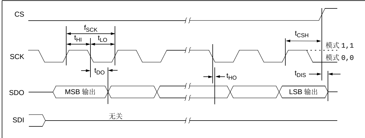
图 29-20: 串行输出时序图
