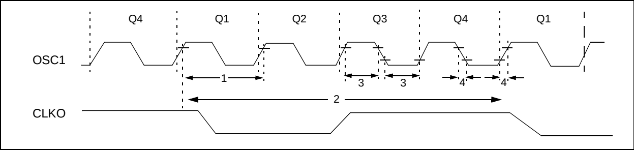
图 29-4: 外部时钟时序
