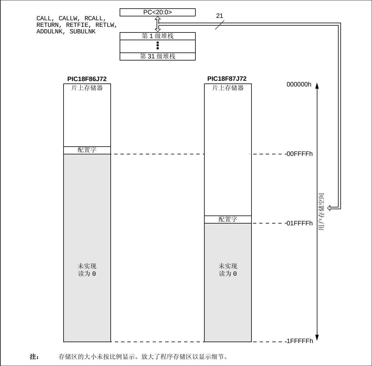
图 6-1: PIC18F87J72 系列器件的存储器映射
