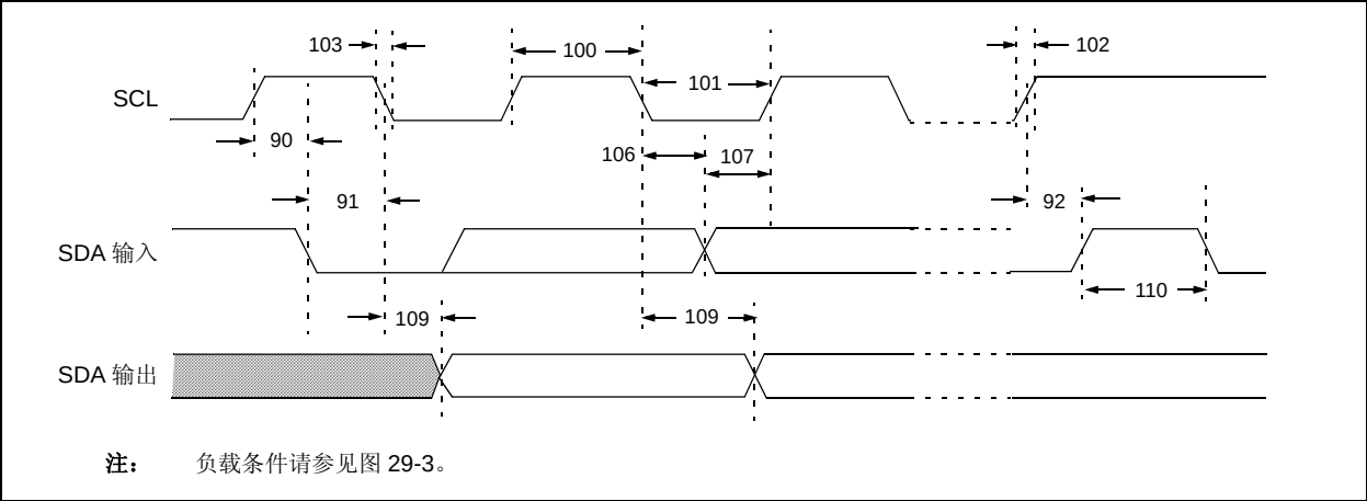
图 29-14: I 2 C™ 总线数据时序
