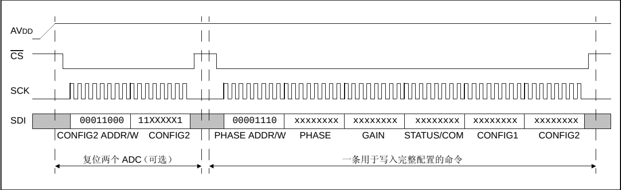
图 B-12: 上电时的建议配置序列
