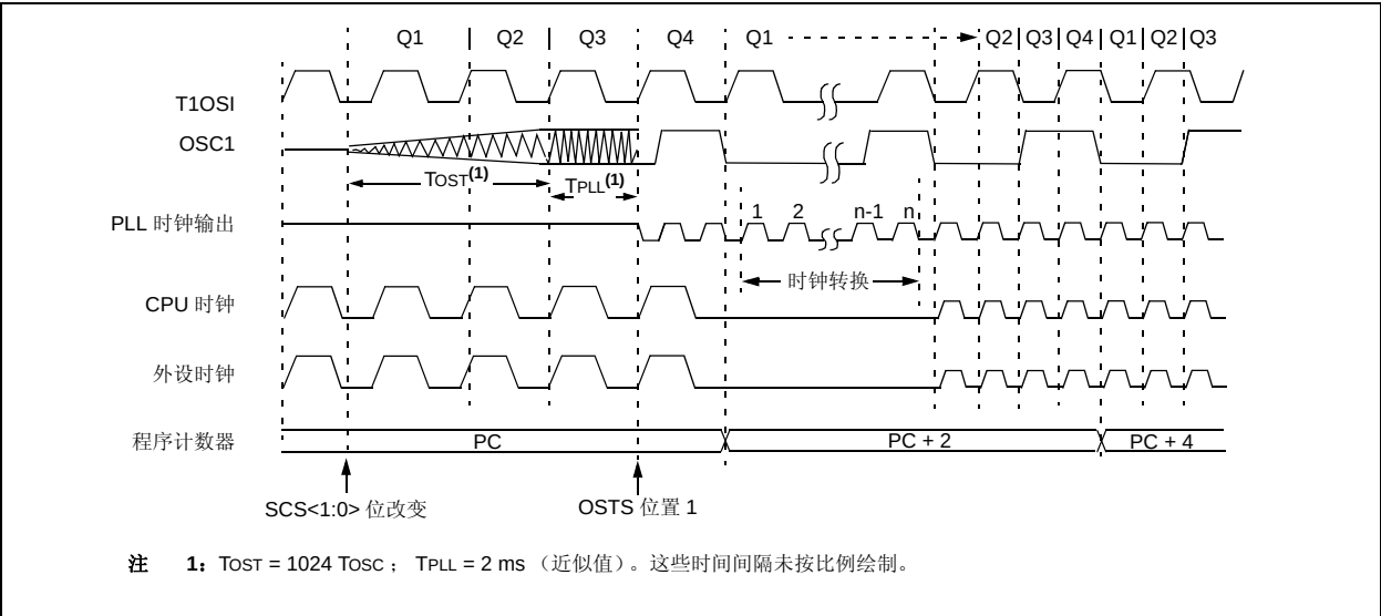
图 4-2: 从 SEC_RUN 模式切换到 PRI_RUN 模式的转换时序 (HSPLL)
