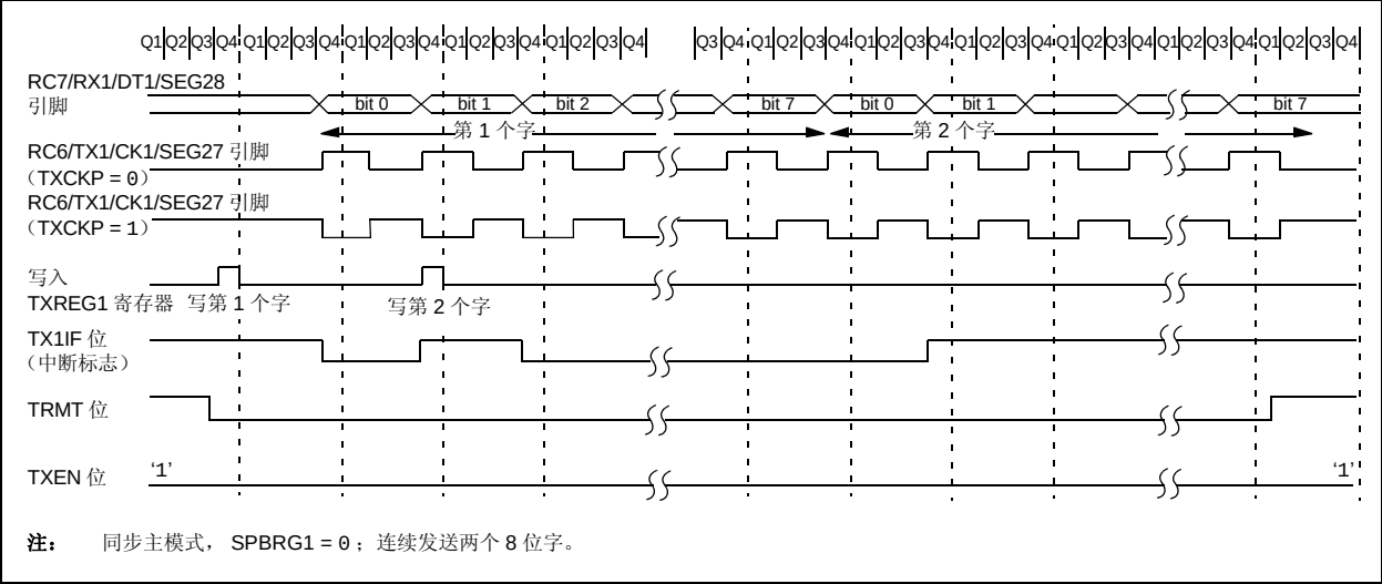
图 19-11: 同步发送
