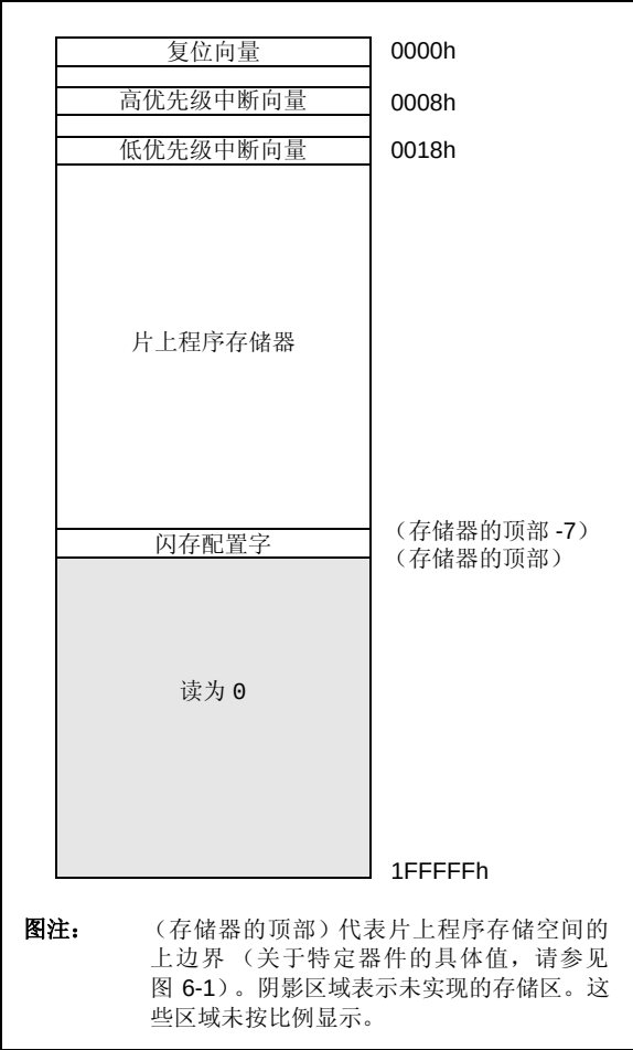
图 6-2: PIC18F87J72 系列器件的硬编码向量和配置字单元
