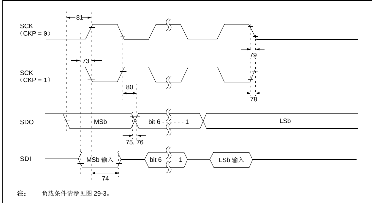
图 29-10: SPI 主模式时序示例 (CKE = 1)
