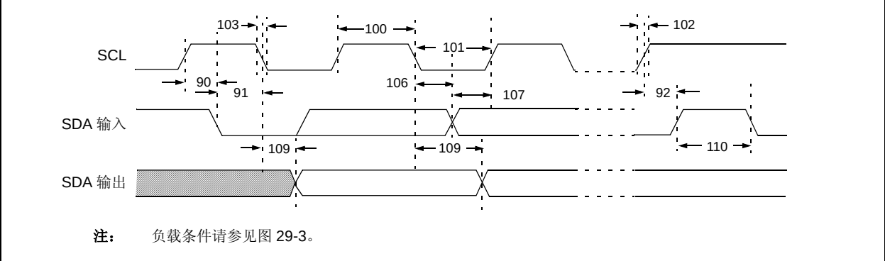
图 29-16: MSSP I 2 C™ 总线数据时序
