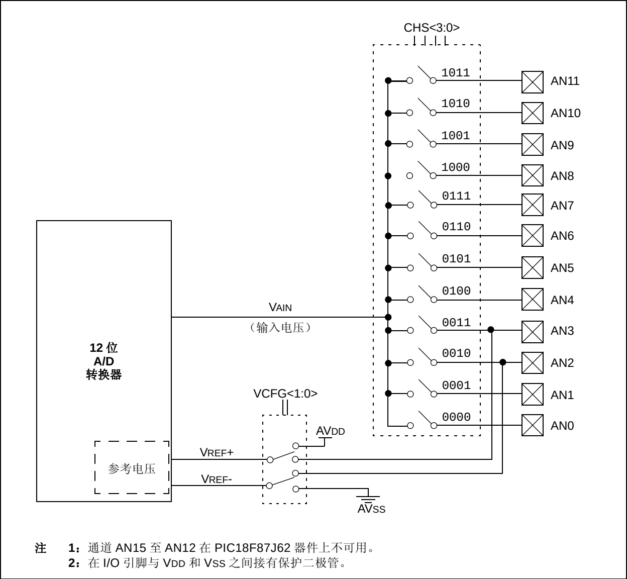
图 21-1: A/D 框图 (1,2)
