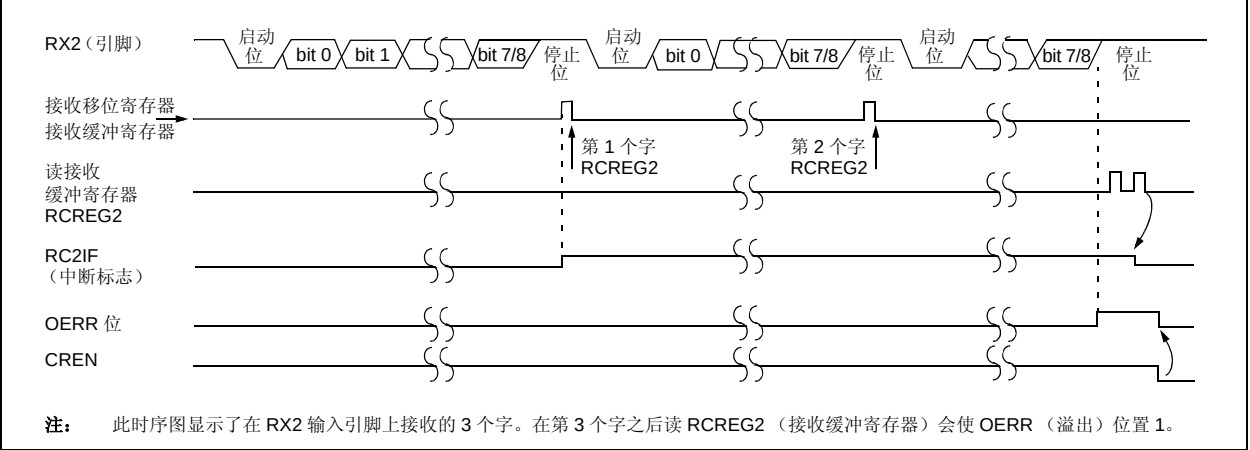
图 20-5: 异步接收
