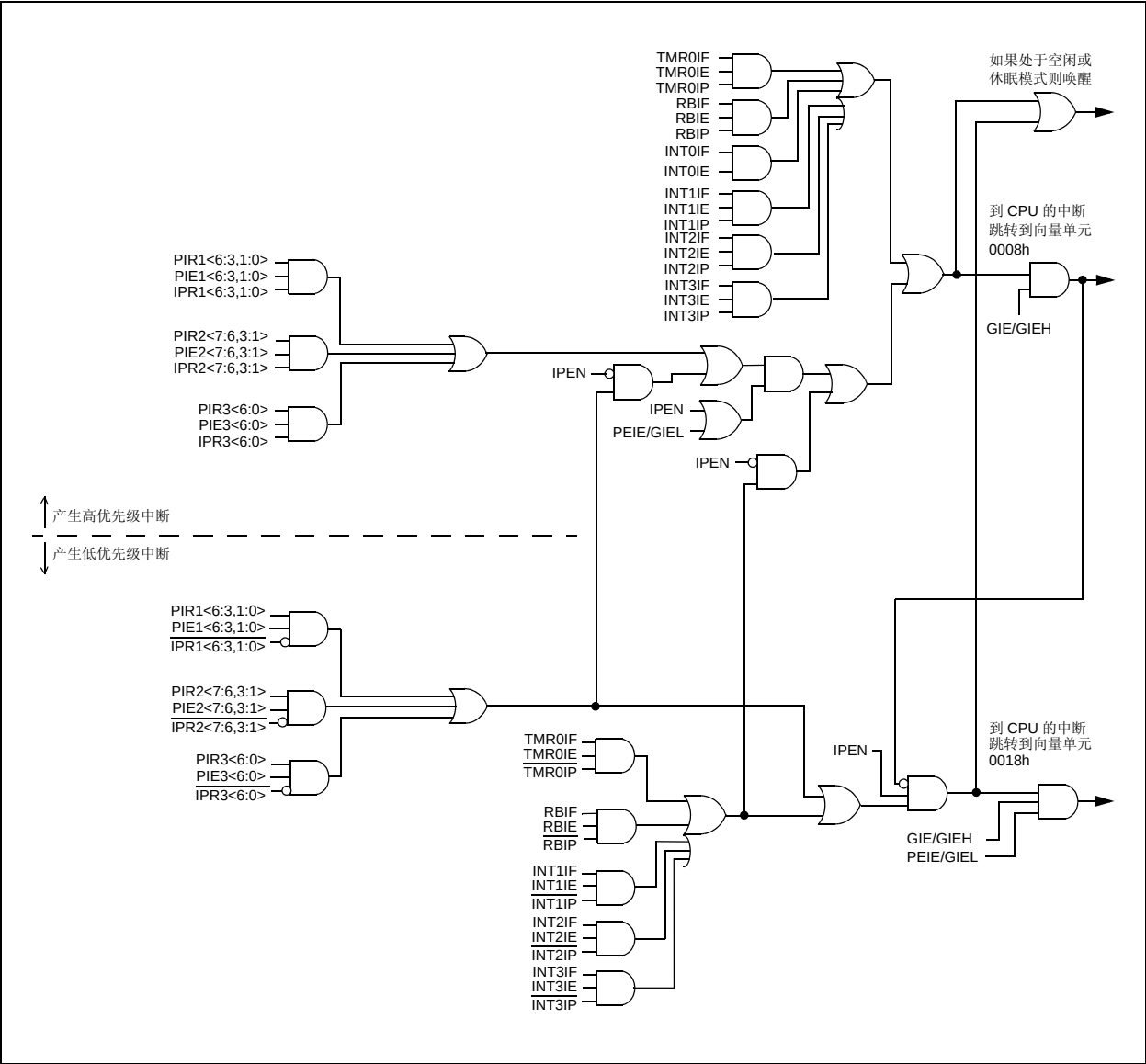
图 9-1: PIC18F87J72 系列中断逻辑
