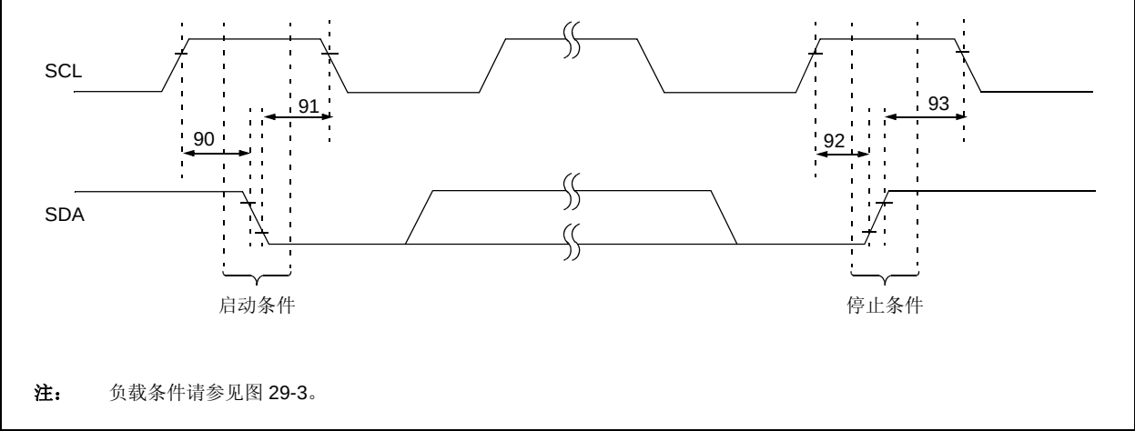
图 29-15: MSSP I 2 C™ 总线启动位 / 停止位时序波形
