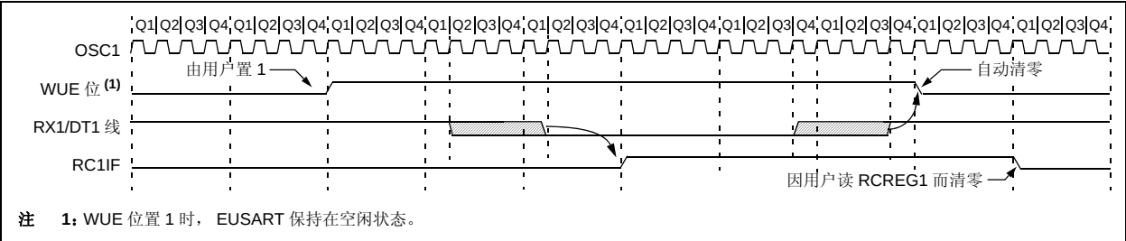
图 19-8: 正常操作时的自动唤醒位（WUE）时序
