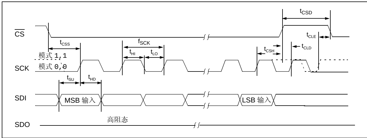
图 29-21: 串行输入时序图
