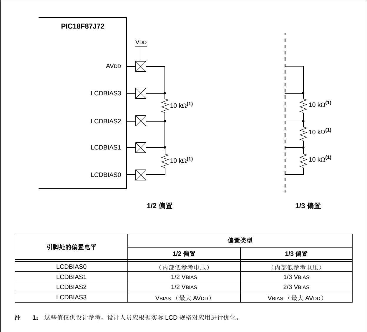
图 17-4: M2 配置的梯形电阻网络连接
