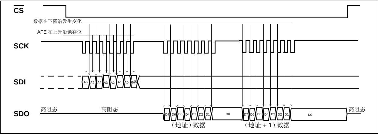
图 B-7: 器件读操作（SPI 模式 1,1——时钟空闲时为高电平）
