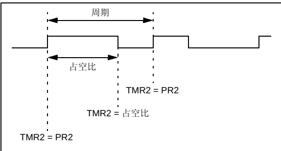
图 16-5: PWM 输出
