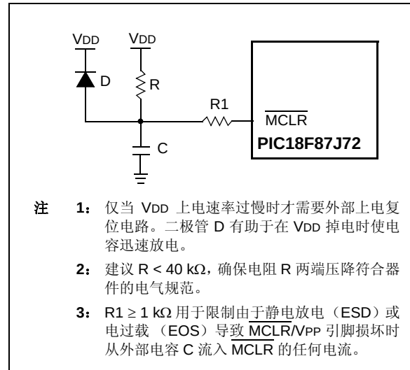
图 5-2: 外部上电复位电路 ( V_{DD} 缓慢上电的情况)
