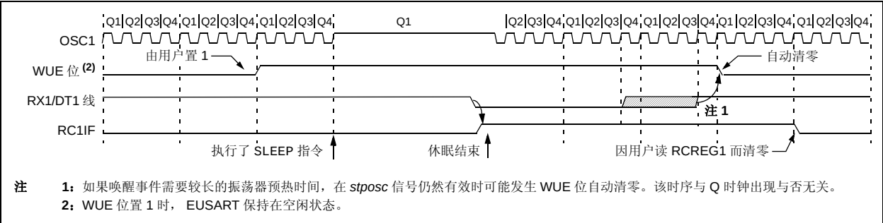
图 19-9: 休眠时的自动唤醒位（WUE）时序
