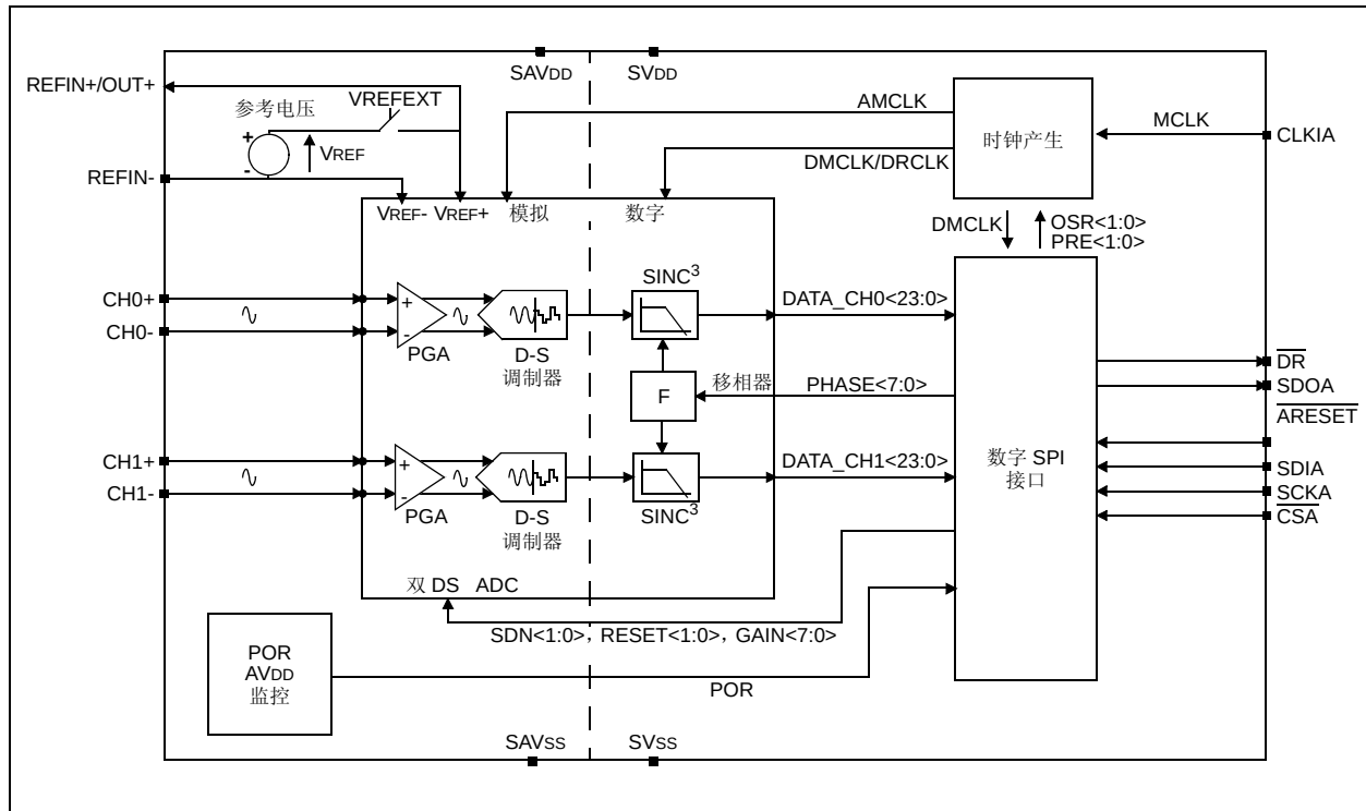
图 B-1: 双通道 AFE 功能框图
