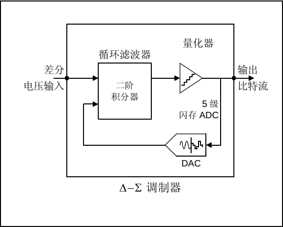
图 B-2: 简化的 Δ-Σ ADC 框图
