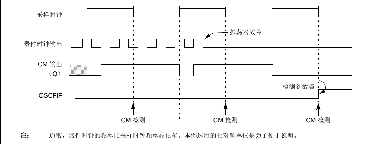
图 26-5: FSCM 时序图
