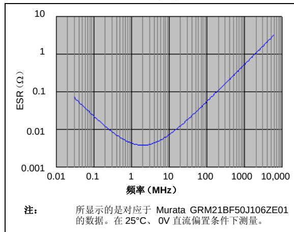
图 2-3: 建议的 VCAP 的频率与 ESR 性能
