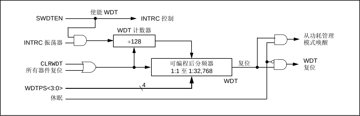
图 26-1: WDT 框图
