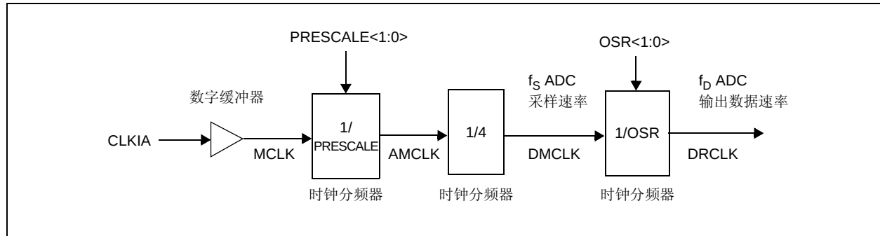
图 B-5: AFE 内部时钟详细信息
