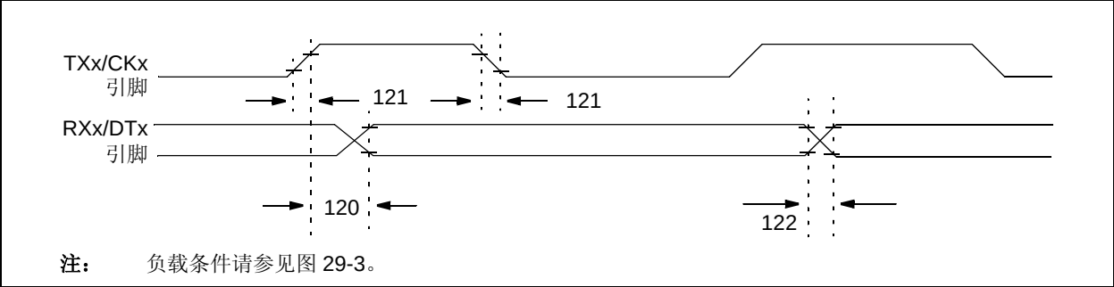
图 29-17: EUSART/AUSART 同步发送（主 / 从）时序
