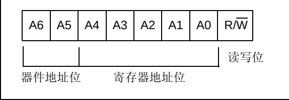
图 22-2: 控制字节
