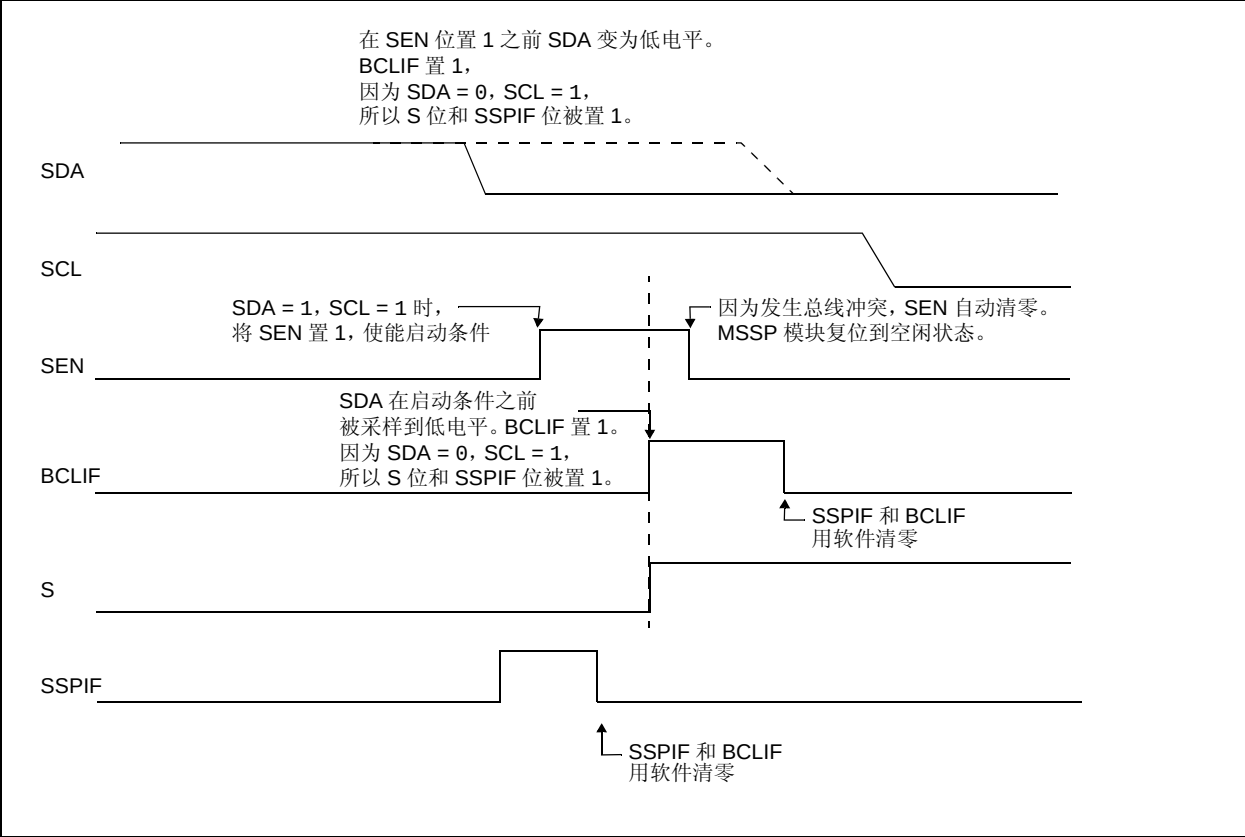
图 18-28: 启动条件期间的总线冲突（仅用于 SDA）
