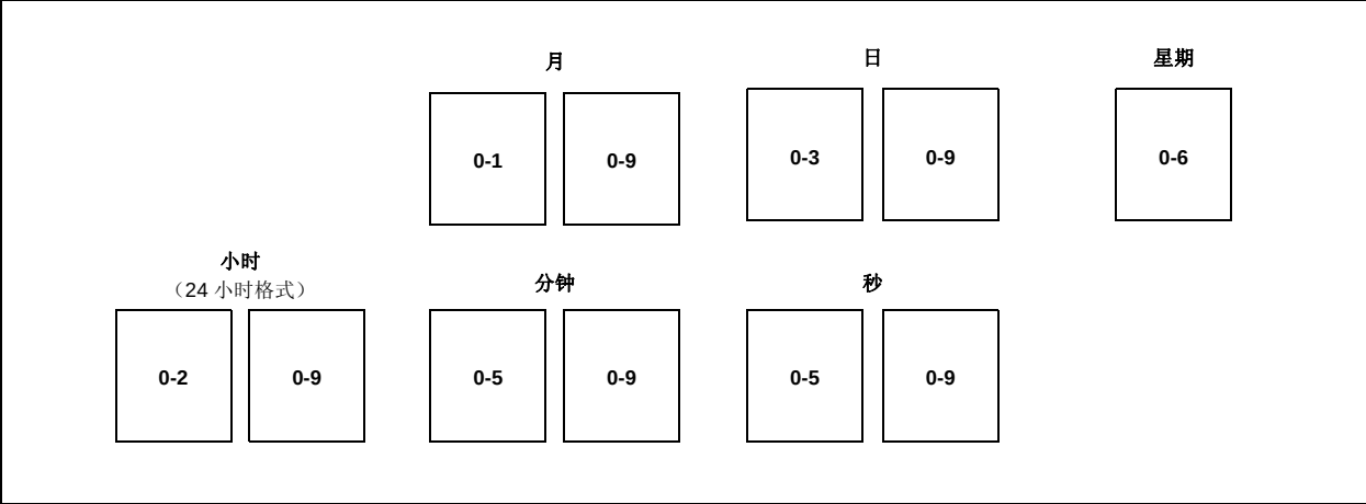
图 15-3: 闹钟位格式
