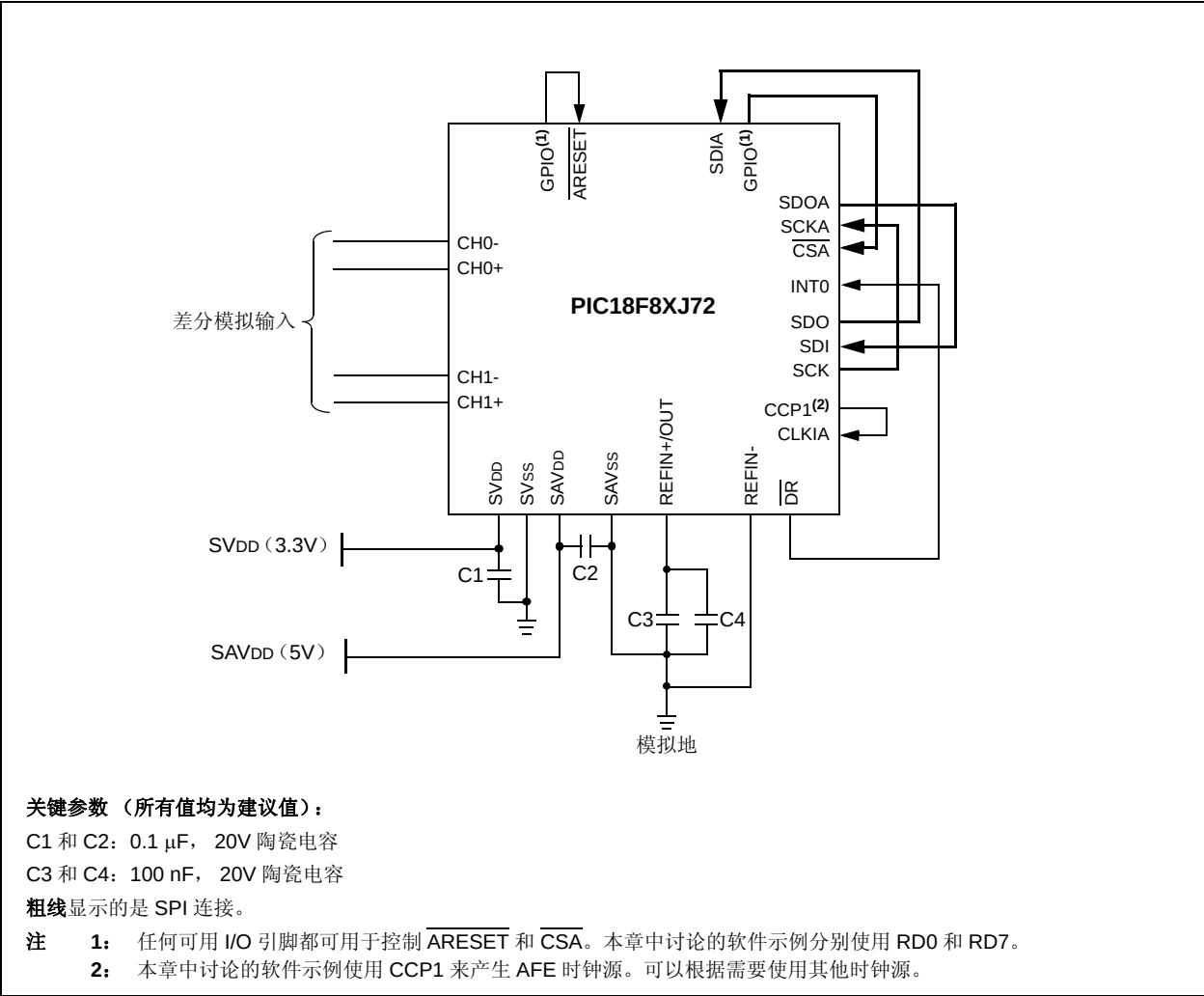
图 22-3: AFE 操作所必需的连接
