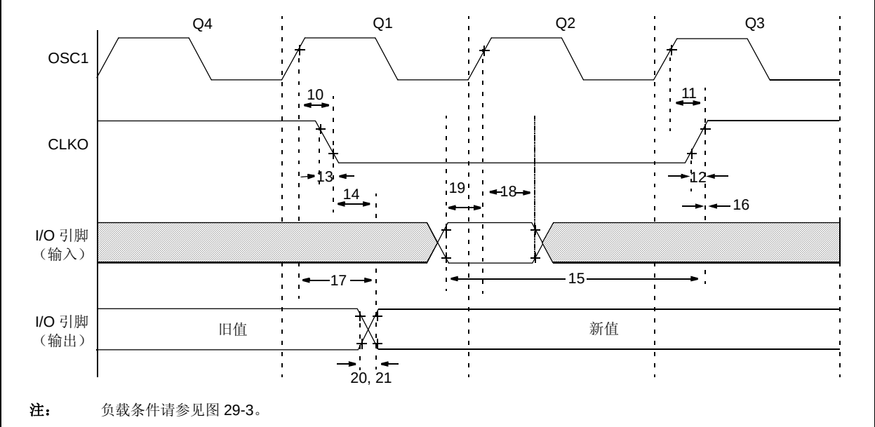
图 29-5: CLKO 和 I/O 时序
