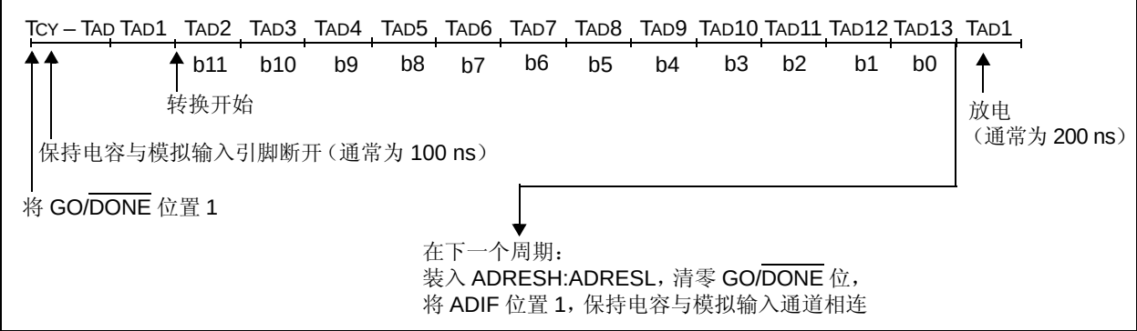
图 21-3: A/D 转换 TAD 周期 ( \text{ACQT}<2:0> = 000, \text{TACQ} = 0 )
