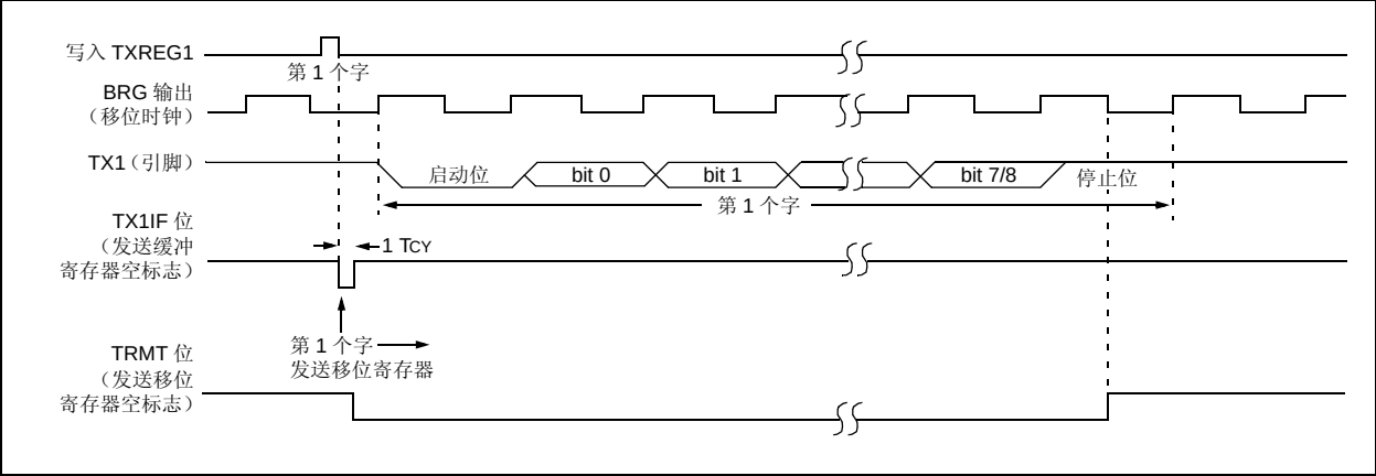
图 19-4: 异步发送
