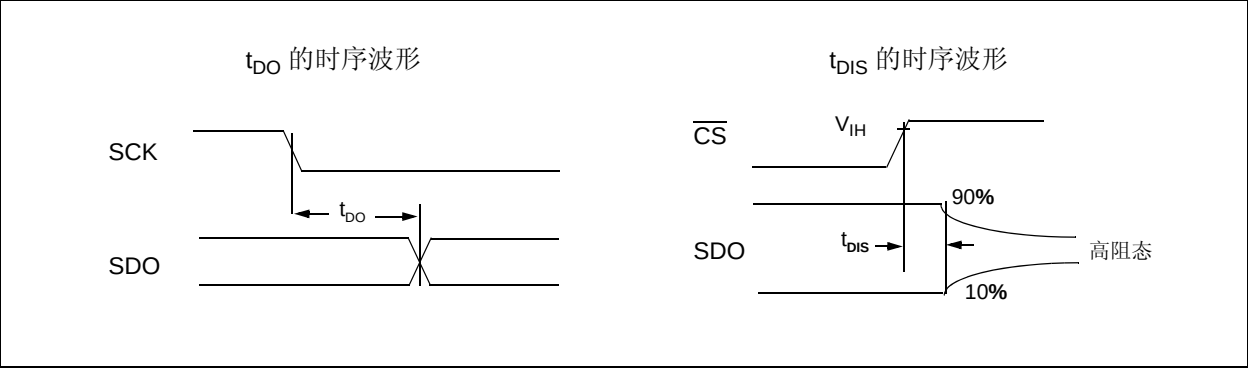
图 29-23: 具体时序图
