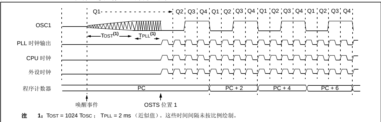
图 4-6: 从休眠模式唤醒的转换时序（HSPLL）
