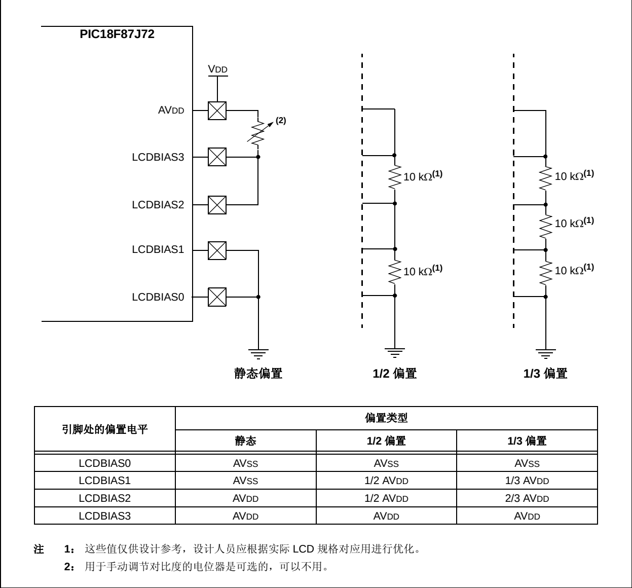
图 17-5: M3 配置的梯形电阻网络连接
