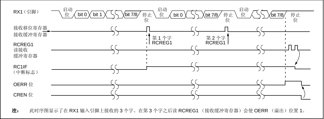
图 19-7: 异步接收
