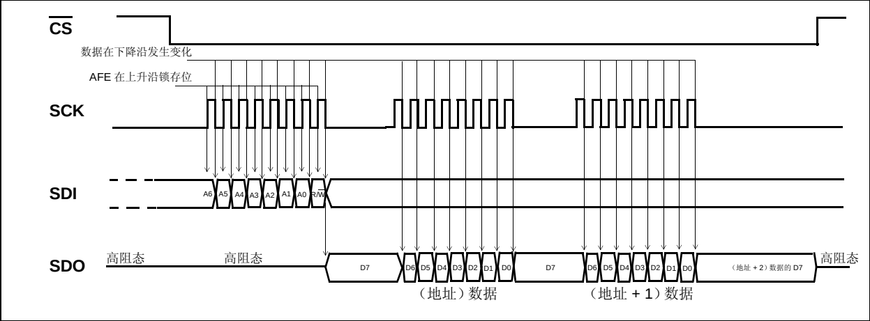
图 B-9: 器件读操作（SPI 模式 0,0——时钟空闲时为低电平）
