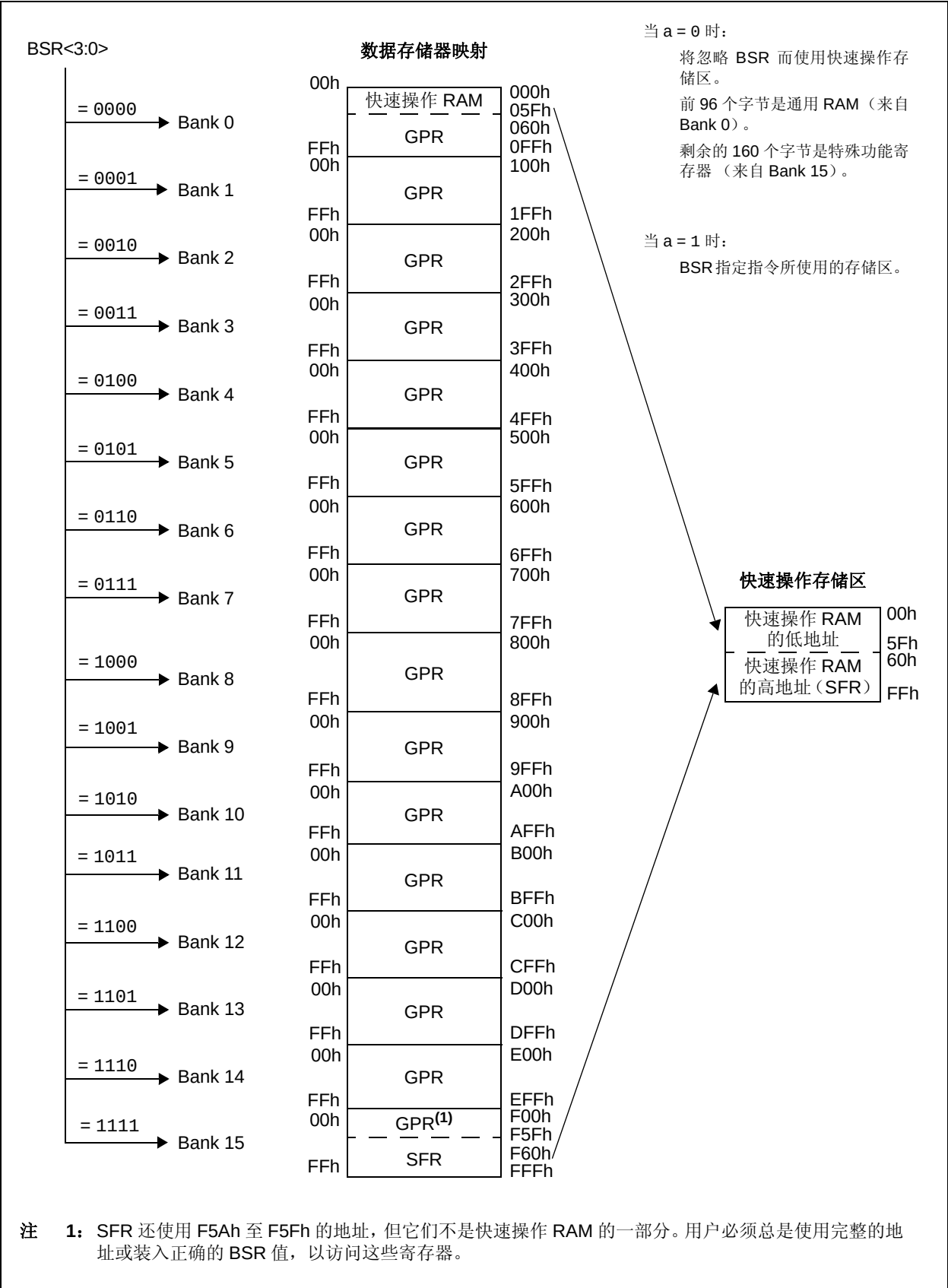
图 6-6: PIC18F86J72 和 PIC18F87J72 器件的数据存储器映射
