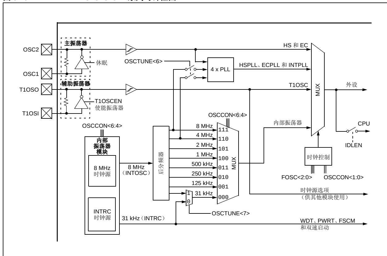
图 3-1: PIC18F87J72 系列时钟框图
