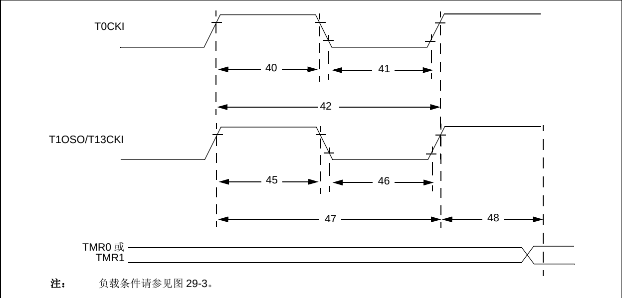
图 29-7: Timer0 和 Timer1 外部时钟时序
