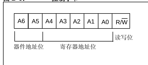
图 B-6: 控制字节
