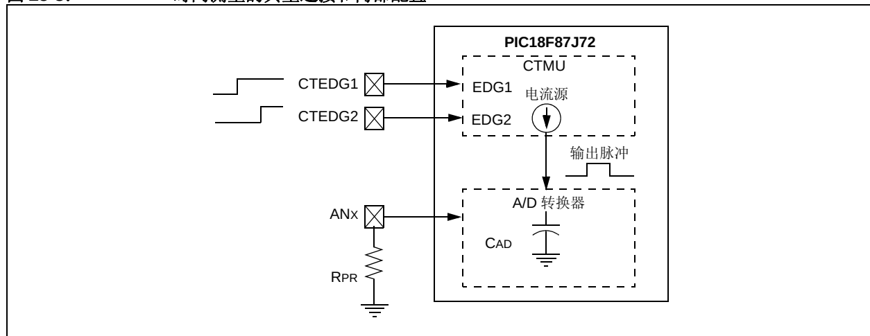
图 25-3: 时间测量的典型连接和内部配置
