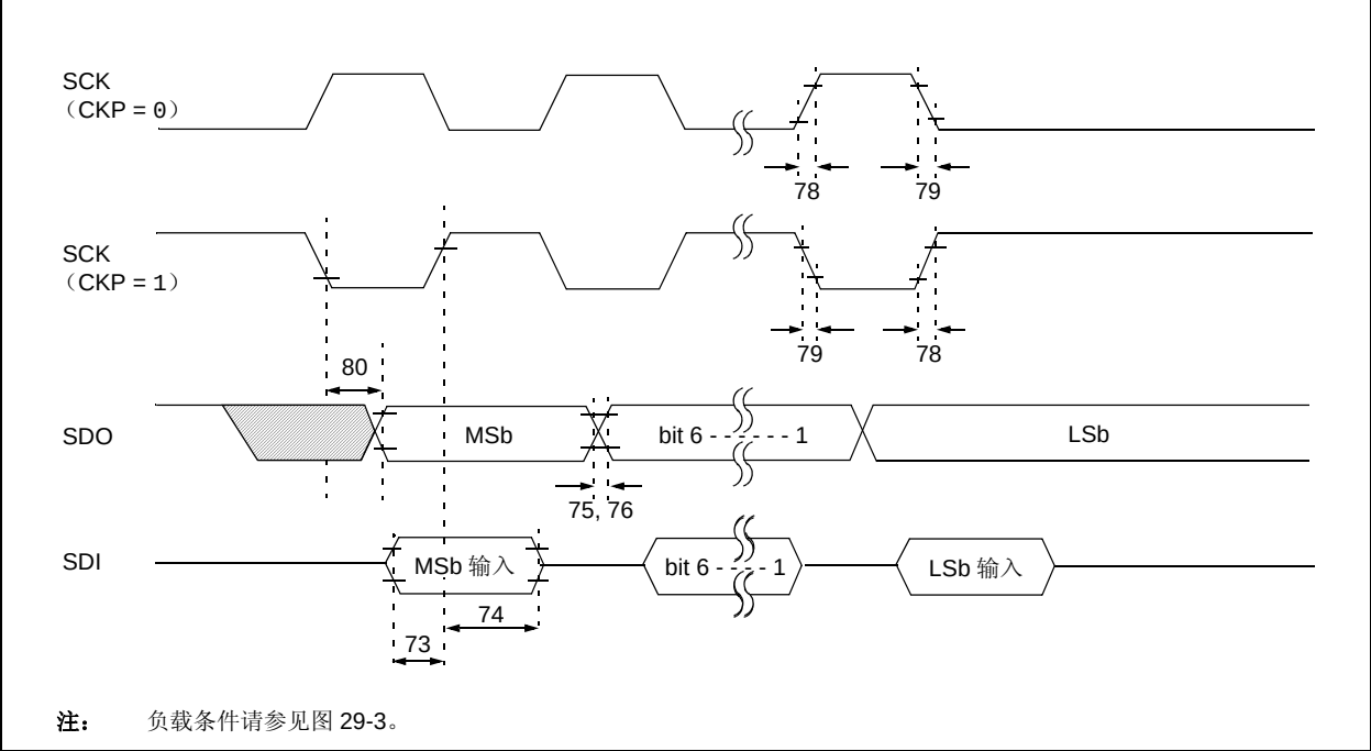
图 29-9: SPI 主模式时序示例 (CKE = 0)
