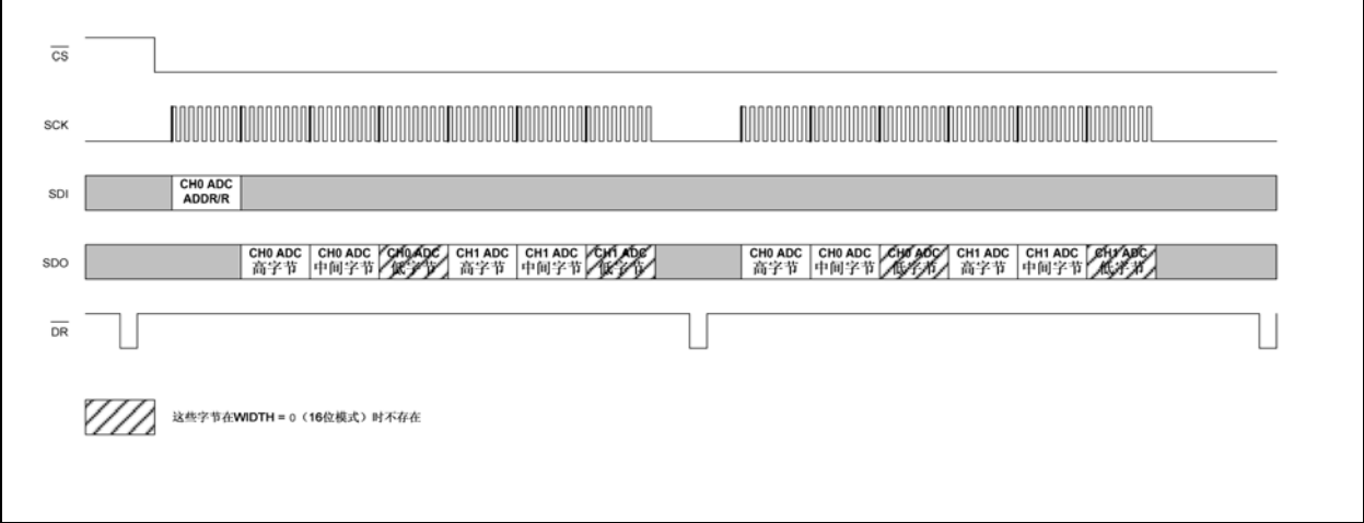
图 B-11: 典型的连续读通信
