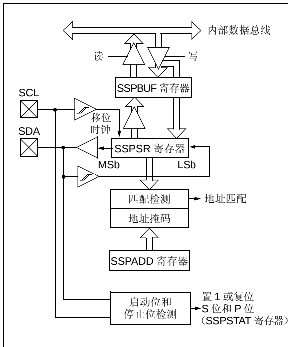
图 18-7: MSSP 框图 (I 2 C™ 模式)
