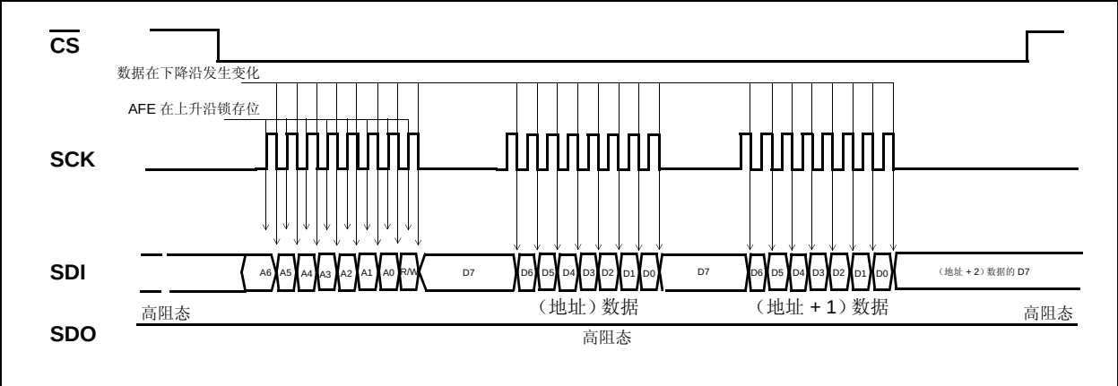
图 B-10: 器件写操作（SPI 模式 0,0——时钟空闲时为低电平）
