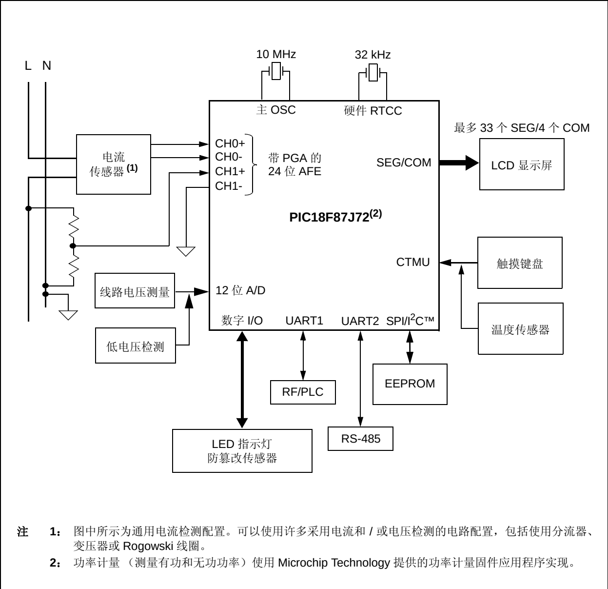
典型应用电路：单相电表
