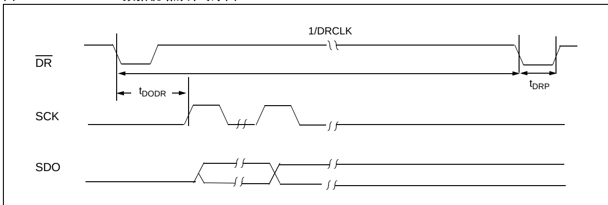
图 29-22: 数据就绪脉冲时序图
