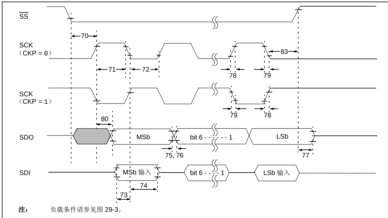
图 29-11: SPI 从模式时序示例 (CKE = 0)
