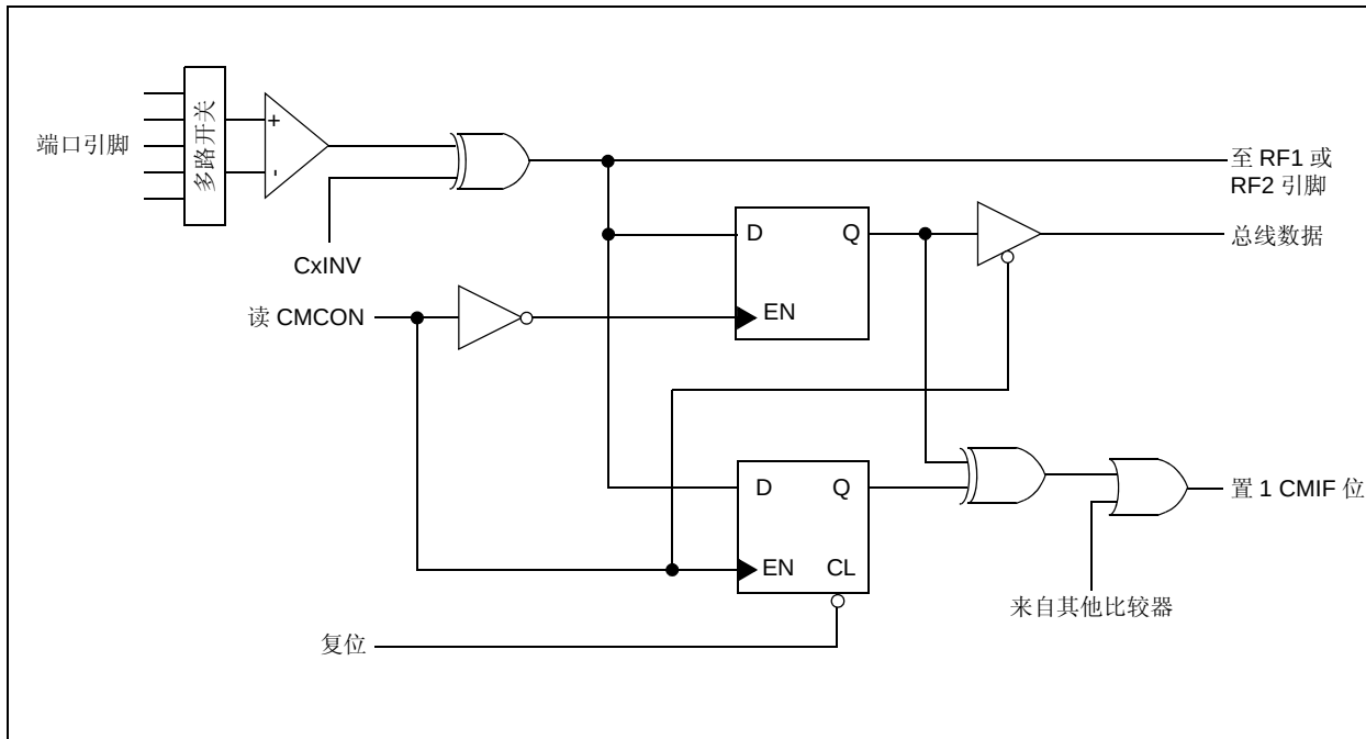
图 23-3: 比较器输出框图
