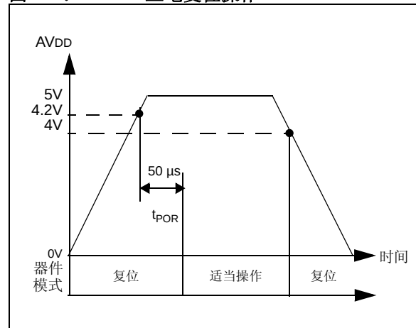
图 B-4: 上电复位操作
