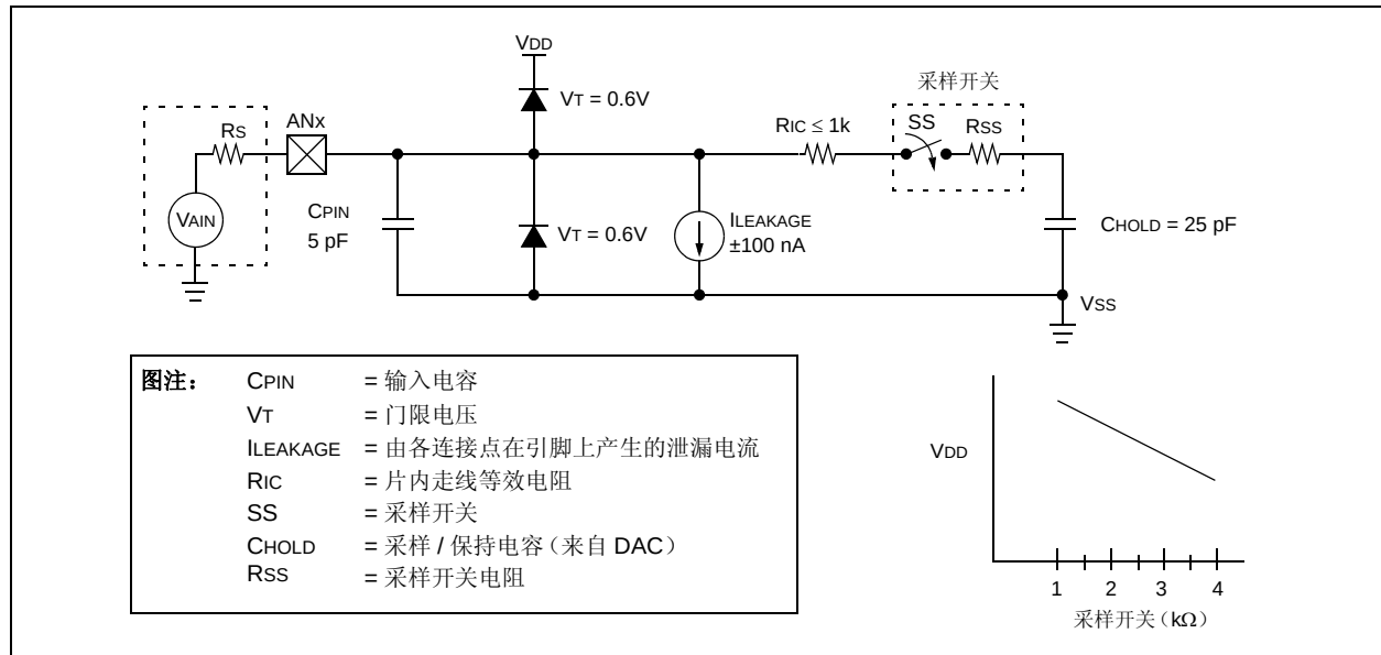
图 21-2: 模拟输入模型
