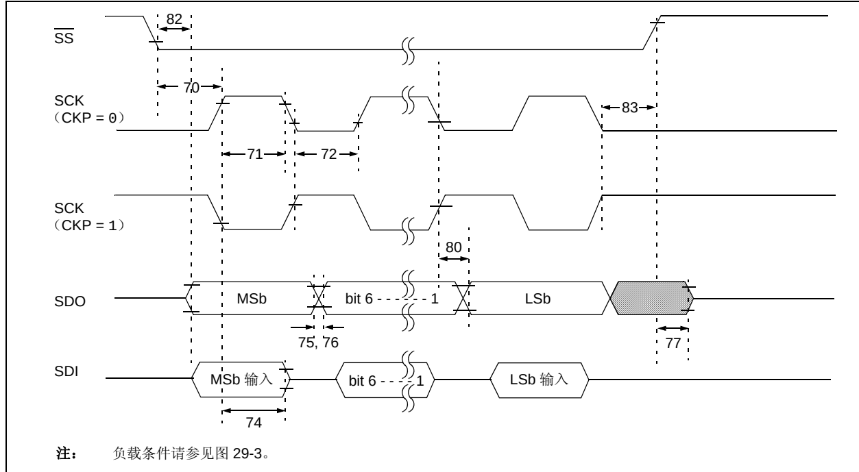
图 29-12: SPI 从模式时序示例 (CKE = 1)
