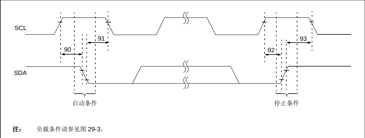
图 29-13: I 2 C™ 总线启动位 / 停止位时序
