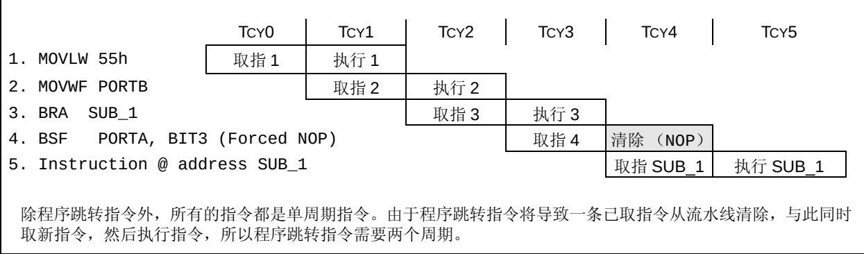
例 6-3: 指令流水线流程
