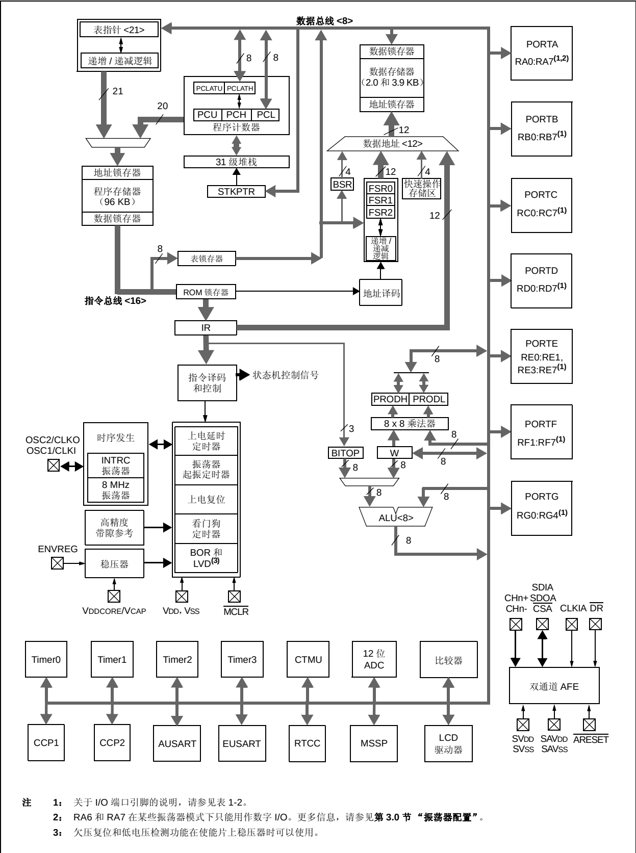
图 1-1: PIC18F8XJ72 (80 引脚) 框图
