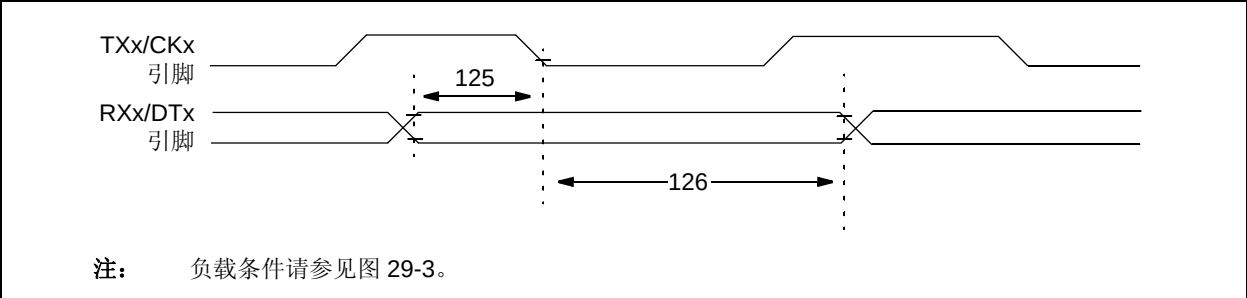
图 29-18: EUSART/AUSART 同步接收（主 / 从）时序
