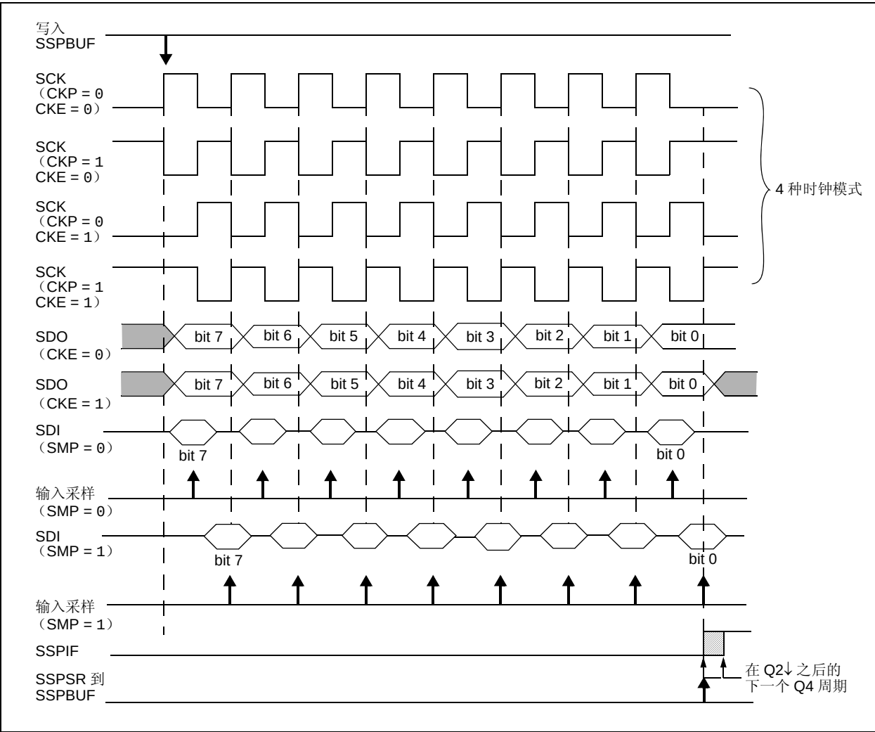
图 18-3: SPI 模式波形图（主模式）
