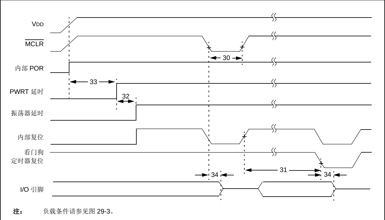
图 29-6: 复位、看门狗定时器、振荡器起振定时器和上电延时定时器时序
