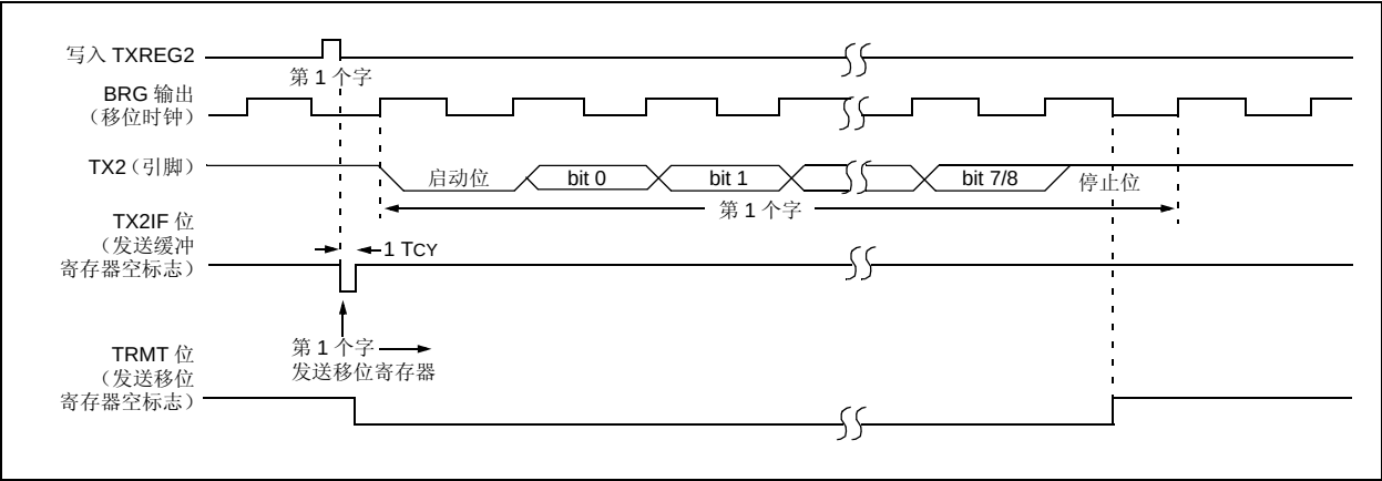
图 20-2: 异步发送
