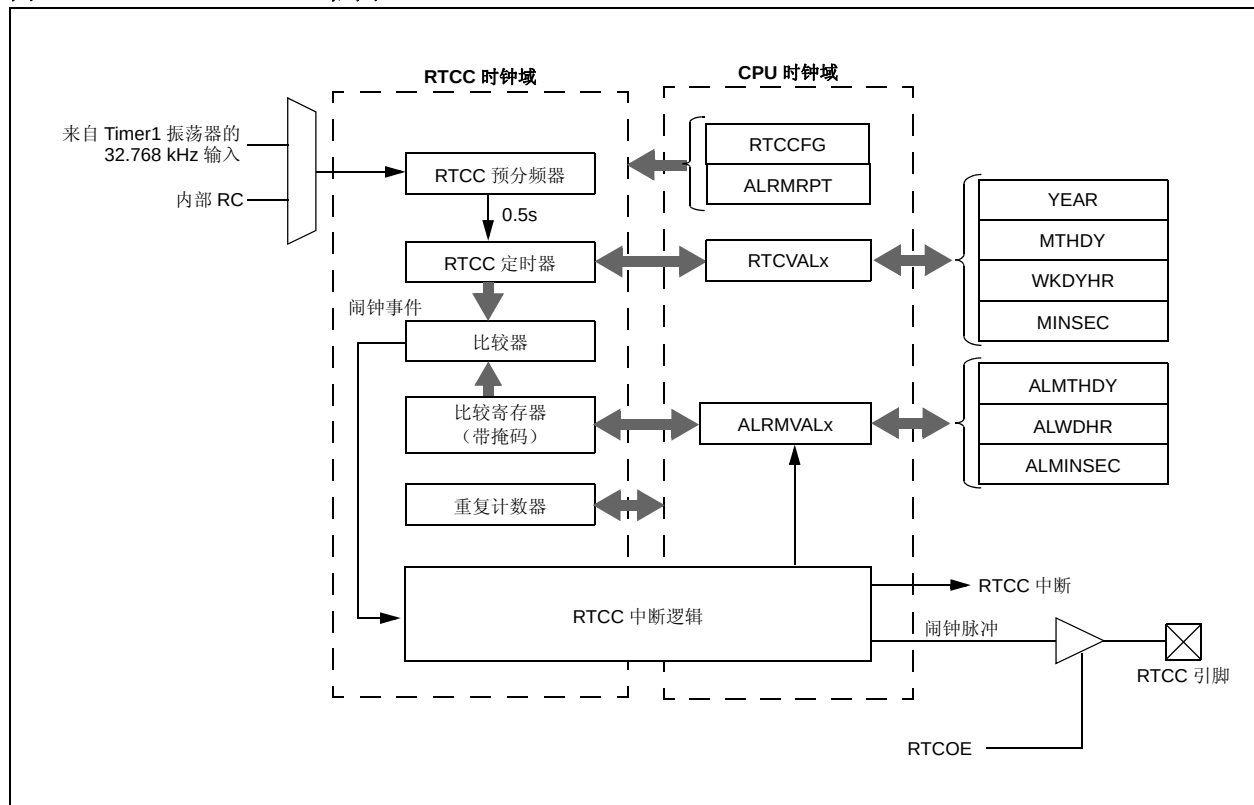
图 15-1: RTCC 框图
