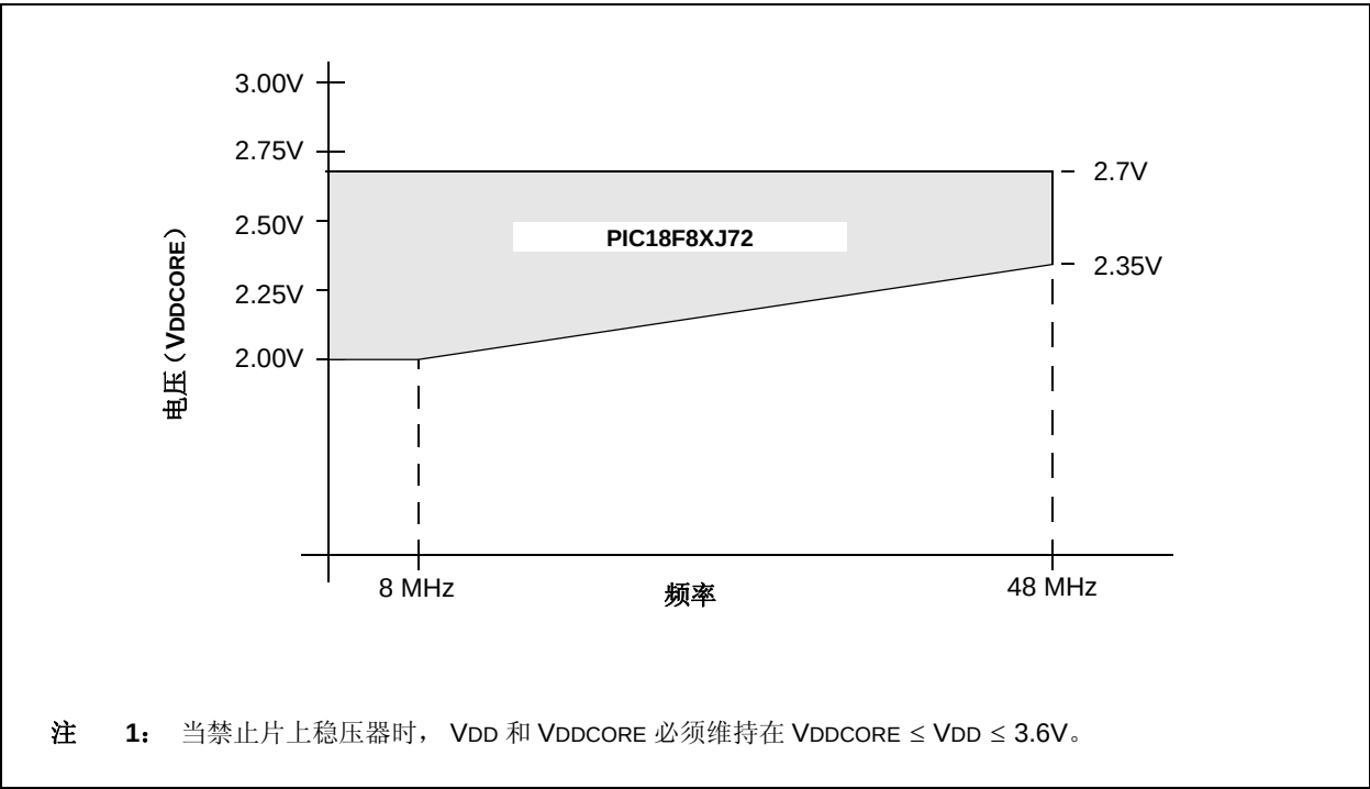
图 29-2: 电压—频率关系图，禁止稳压器（工业级） (1,2)
