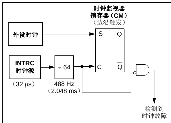
图 26-4: FSCM 框图
