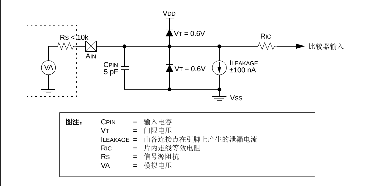
图 23-4: 比较器模拟输入模型
