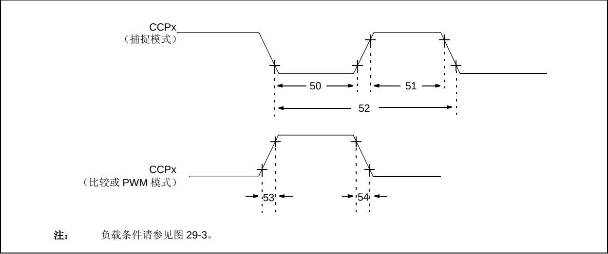
图 29-8: 捕捉 / 比较 / PWM 时序 (CCP1 和 CCP2 模块)
