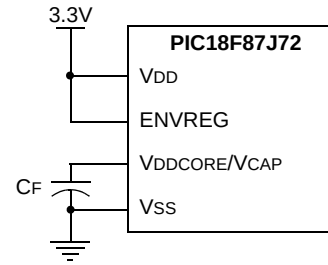
图 26-2: 片上稳压器连接
