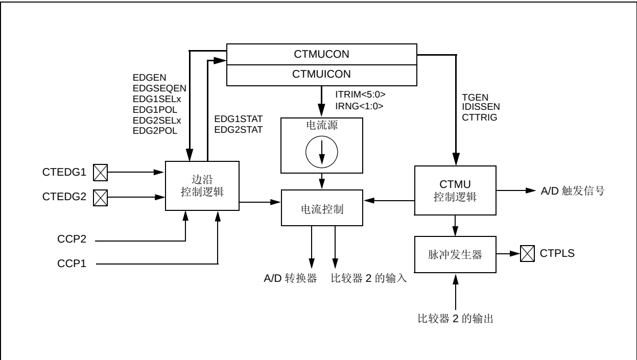
图 25-1: CTMU 框图
