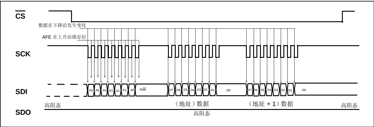
图 B-8: 器件写操作（SPI 模式 1,1——时钟空闲时为高电平）
