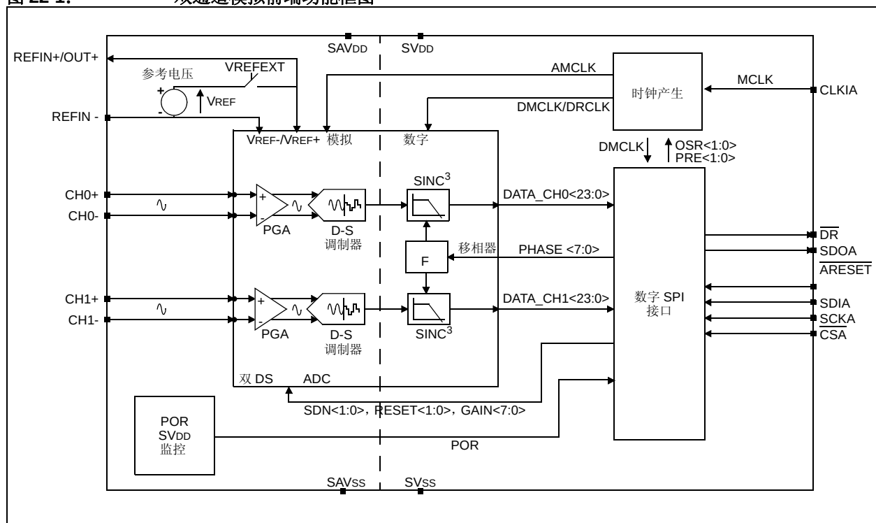
图 22-1: 双通道模拟前端功能框图
