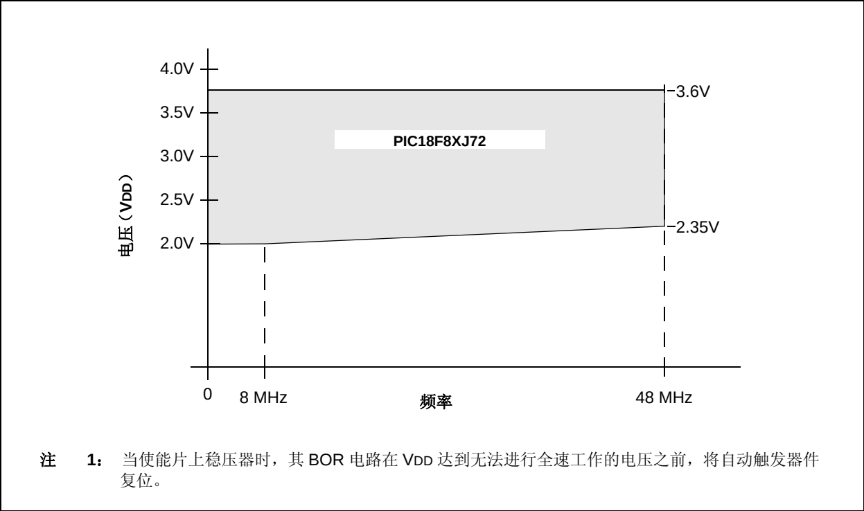
图 29-1: 电压—频率关系图，使能稳压器（工业级） (1)
