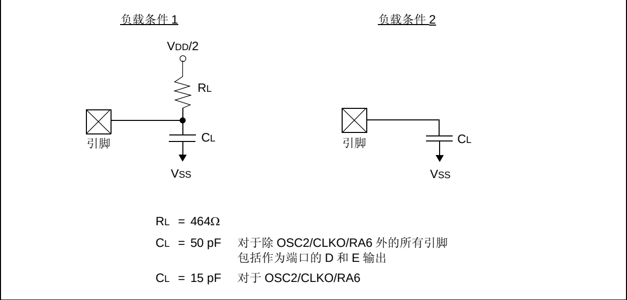
图 29-3: 器件时序规范的负载条件
