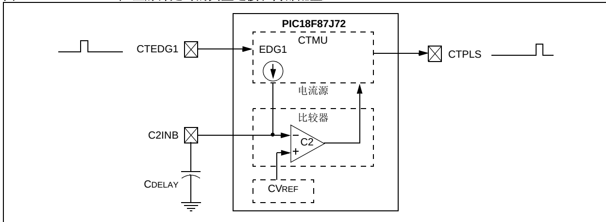
图 25-4：产生脉冲延时的典型连接和内部配置
