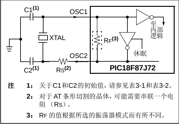
图 3-2: 晶振 / 陶瓷谐振器工作原理 (HS 或 HSPLL 配置)
