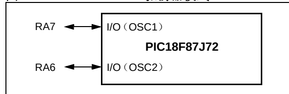
图 3-7: INTIO2 振荡器模式
