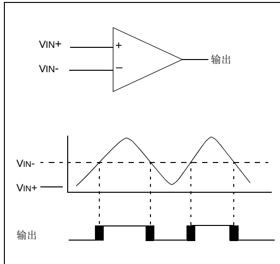
图 23-2: 单比较器
