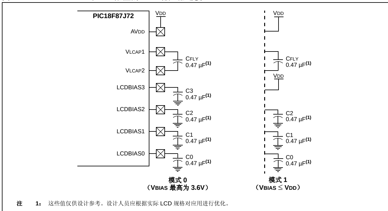
图 17-3: M0 和 M1 配置的 LCD 稳压器连接
