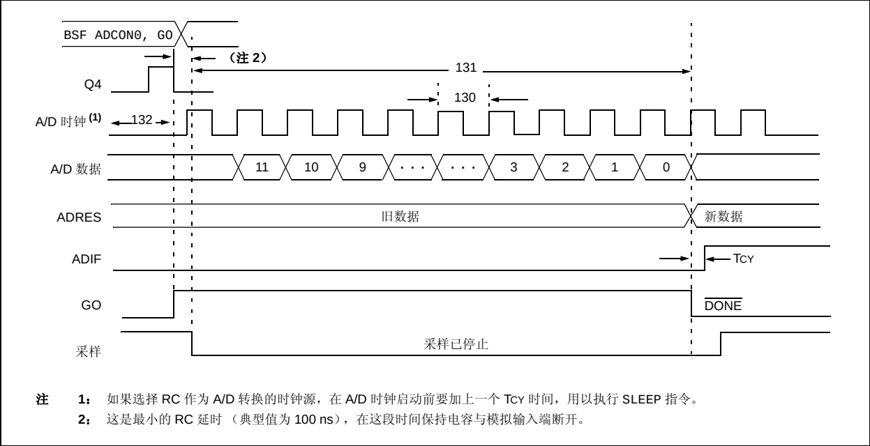
图 29-19: A/D 转换时序
