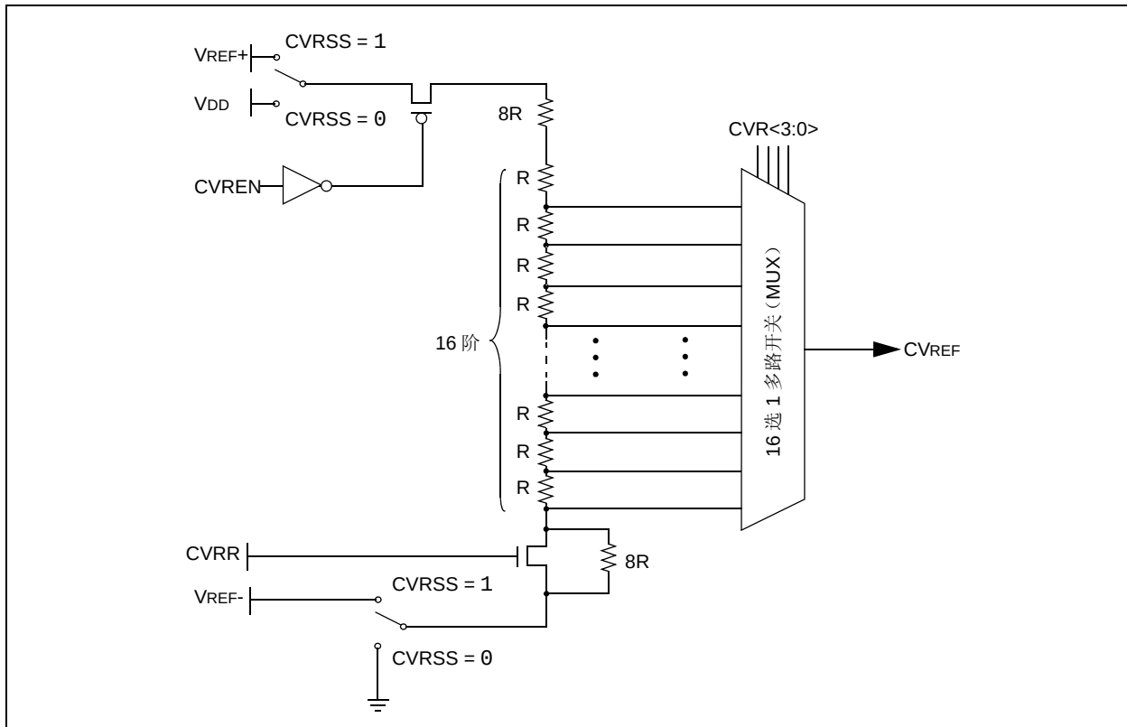
图 24-1: 比较器参考电压模块框图
