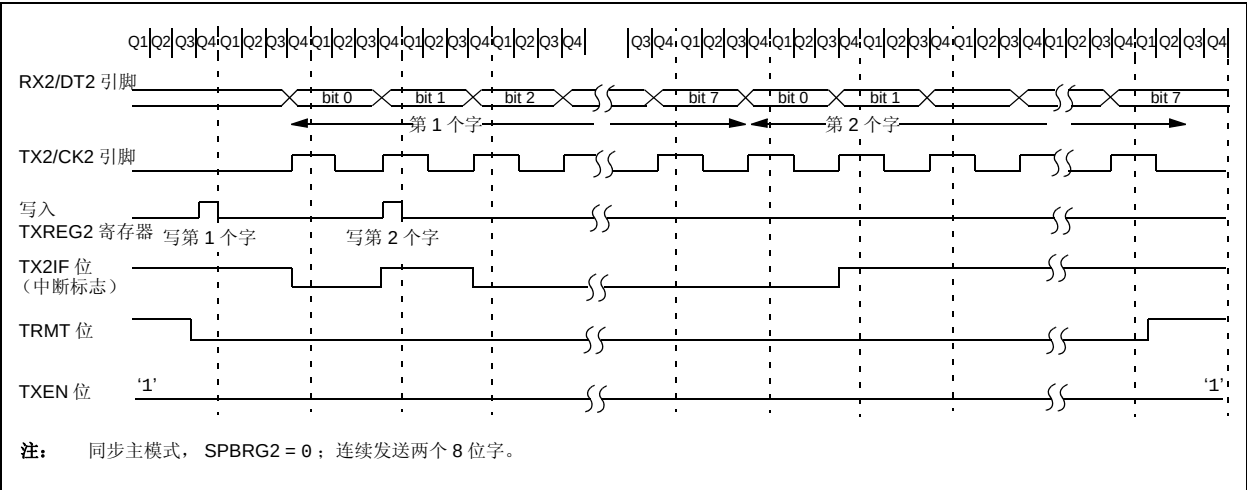
图 20-6: 同步发送
