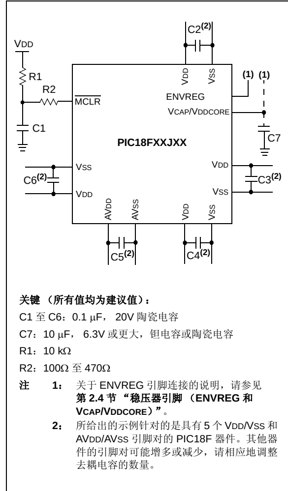
图 2-1: 建议的最低限度连接
