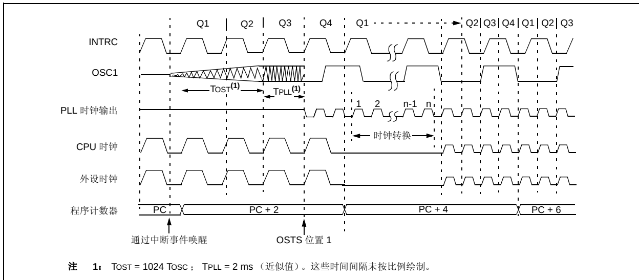
图 26-3: 双速启动时钟转换的时序图（从 INTRC 切换到 HSPLL）
