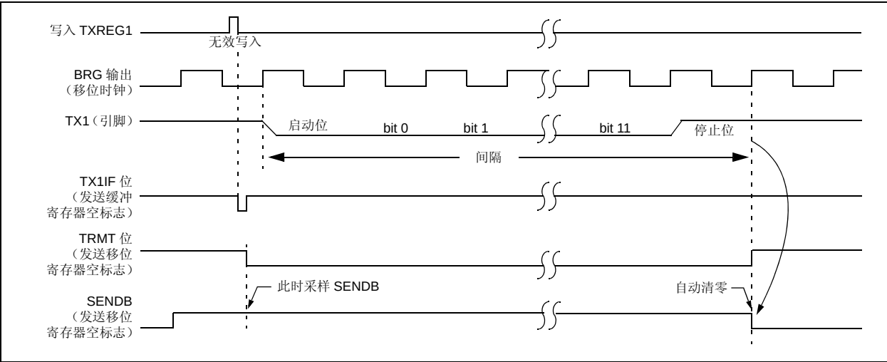
图 19-10: 发送间隔字符序列
