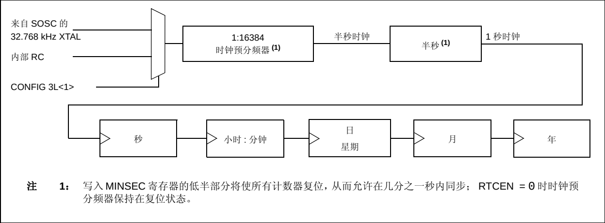
图 15-4: 时钟源复用
