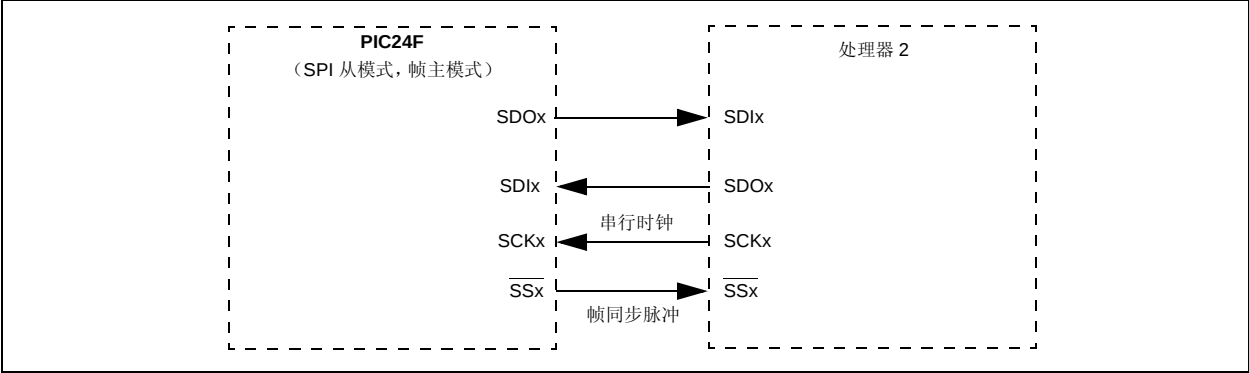
图 15-7: SPI 从 - 帧主模式连接图
