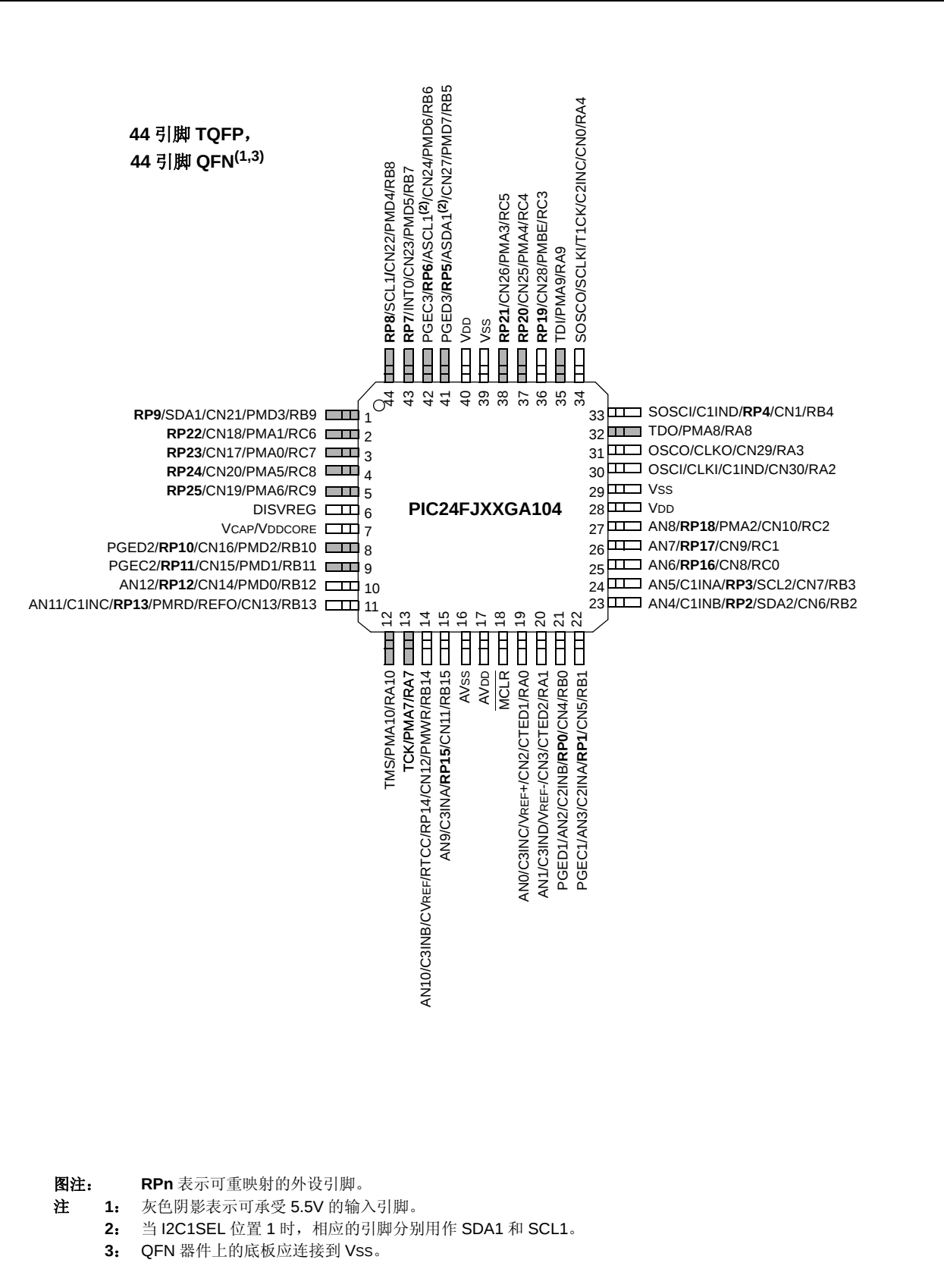
引脚图
