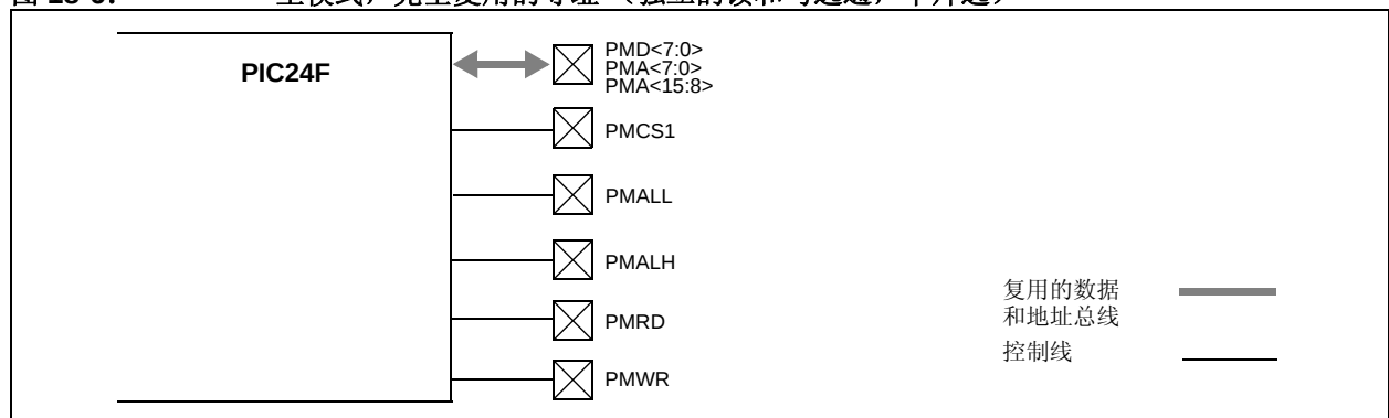
图 18-6: 主模式，完全复用的寻址（独立的读和写选通，单片选）
