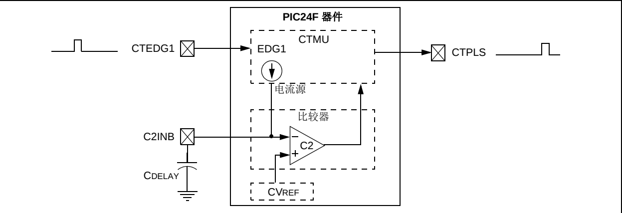
图 24-3: 产生脉冲延时的典型连接和内部配置
