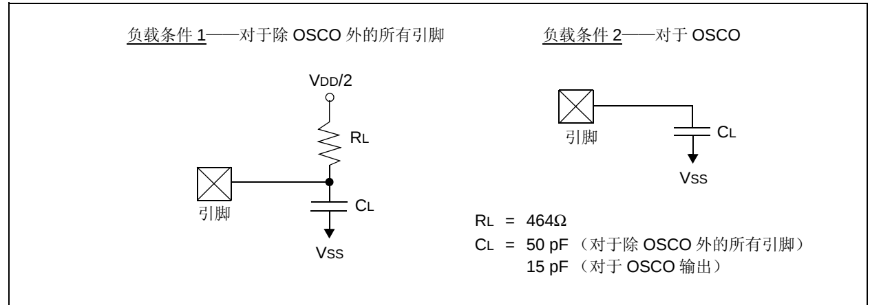
图 28-3: 器件时序规范的负载条件
