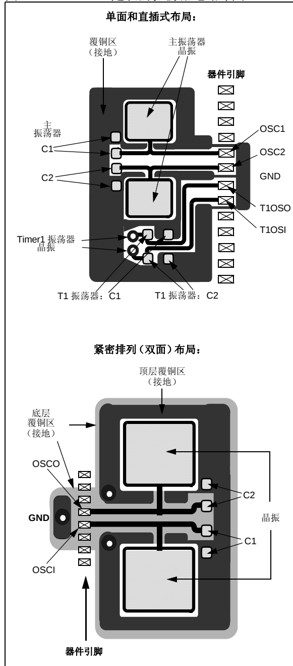
图 2-4: 建议的振荡器电路布局
