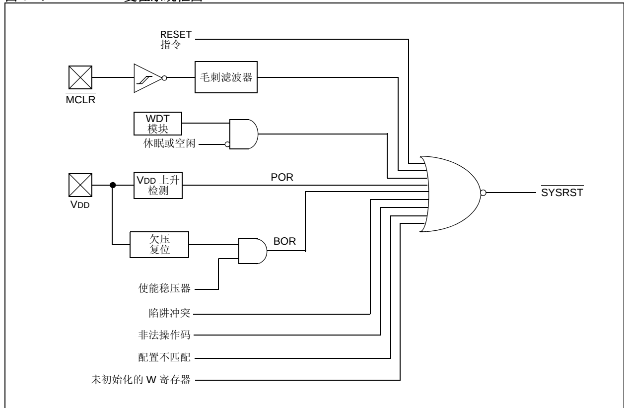
图 6-1: 复位系统框图
