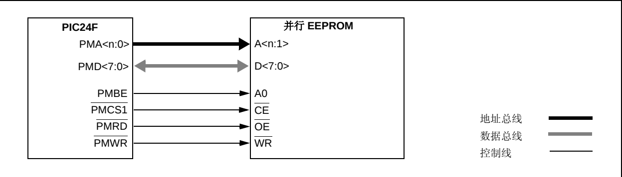
图 18-11: 并行 EEPROM 示例（最多 11 位地址，16 位数据）
