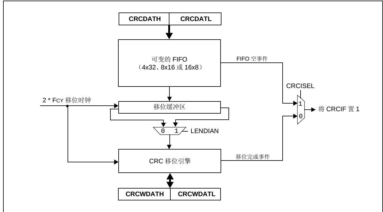
图 20-1: CRC 框图
