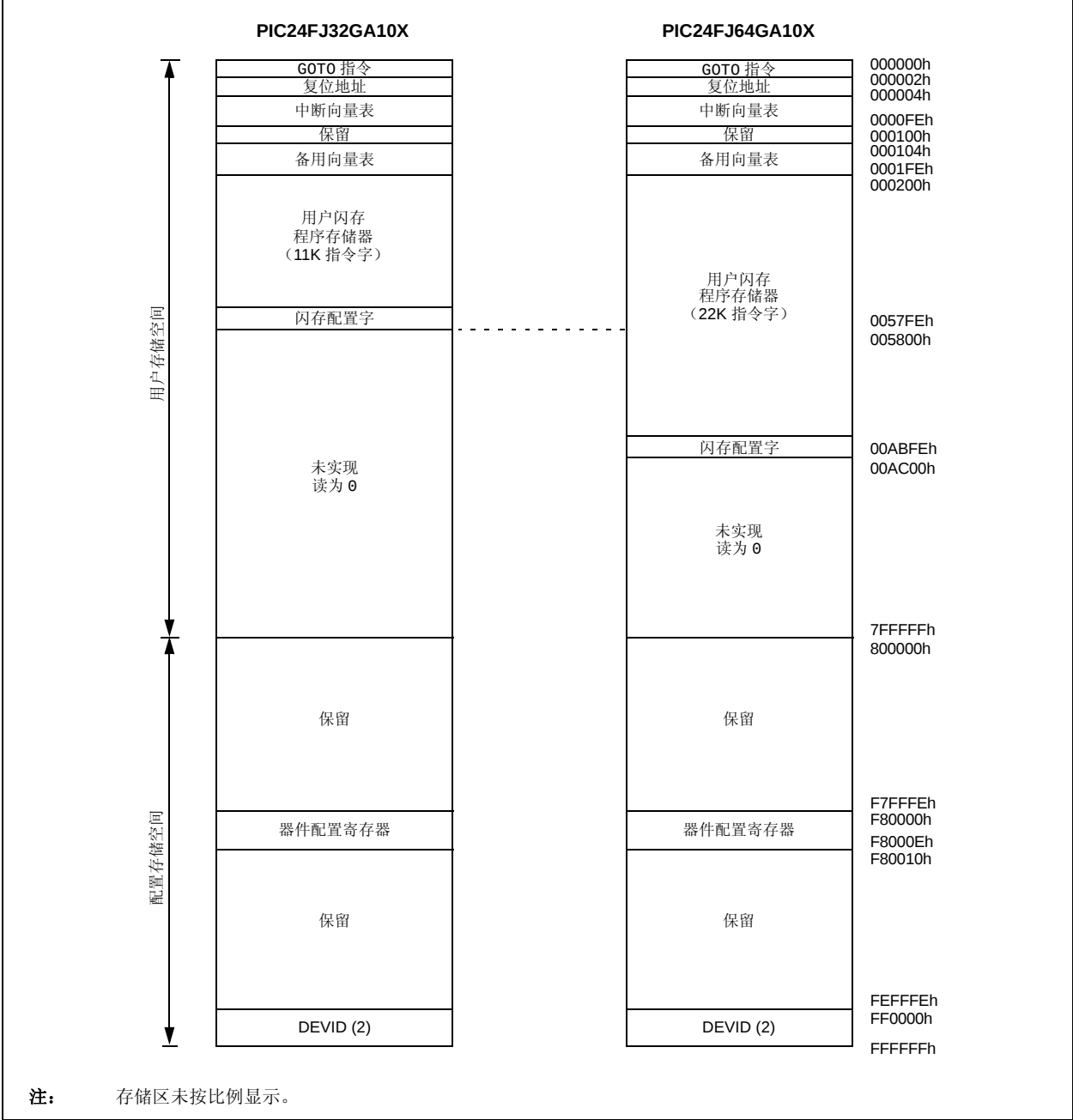
图 4-1: PIC24FJ64GA104 系列器件的程序存储空间映射
