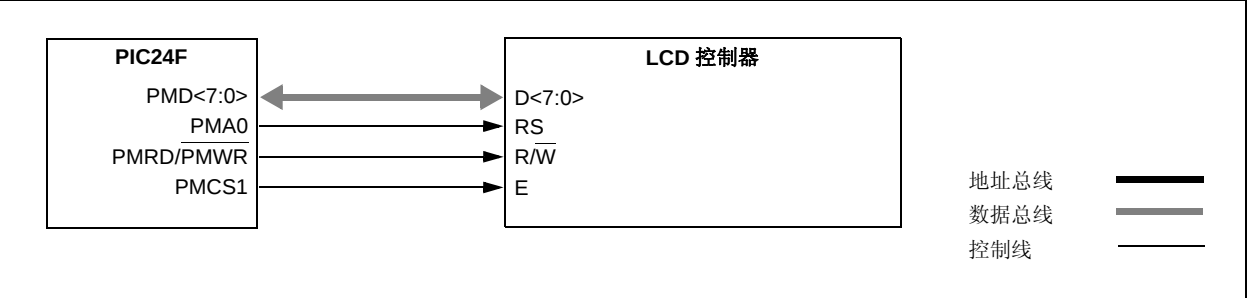
图 18-12: LCD 控制示例（字节模式操作）
