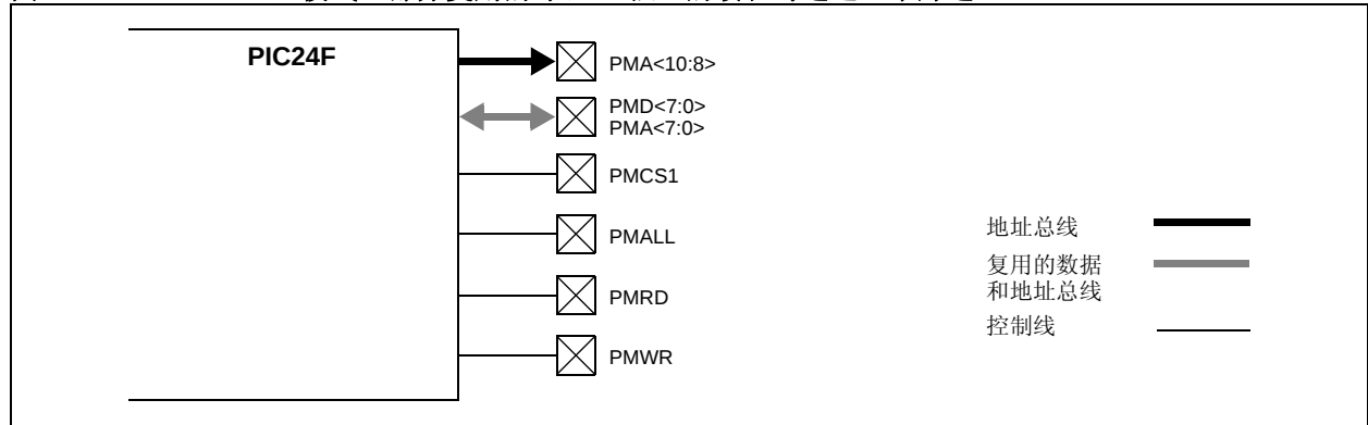
图 18-5: 主模式，部分复用的寻址（独立的读和写选通，单片选）
