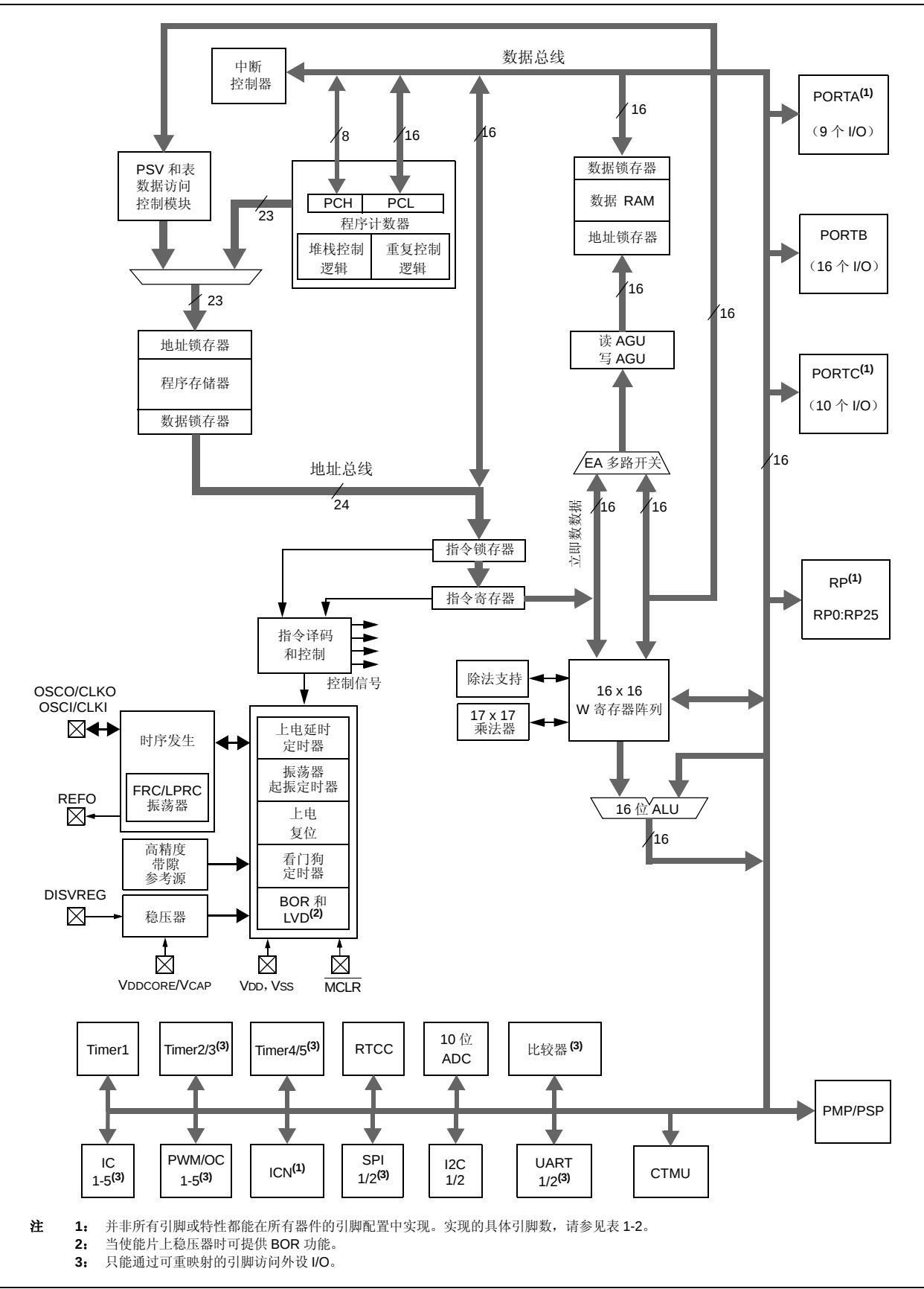
图 1-1: PIC24FJ64GA104 系列一般框图
