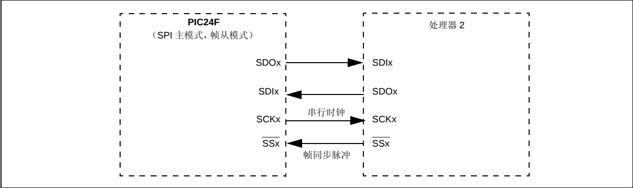
图 15-6: SPI 主 - 帧从模式连接图
