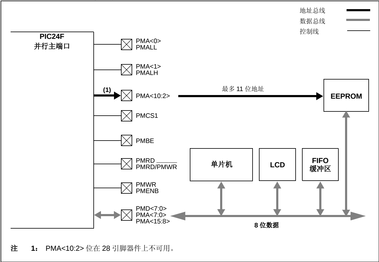
图 18-1: PMP 模块概述
