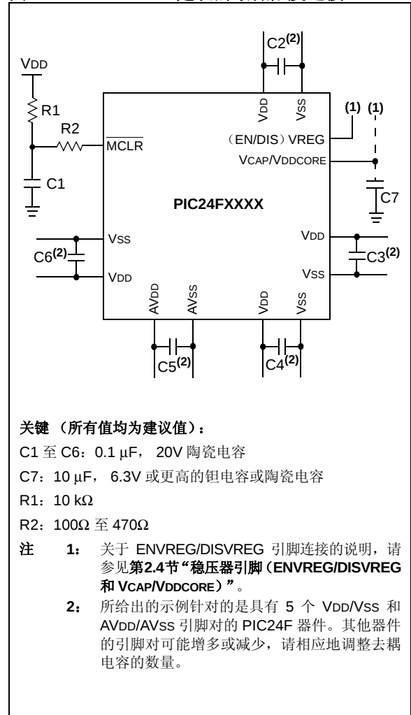
图 2-1: 建议的最低限度连接
