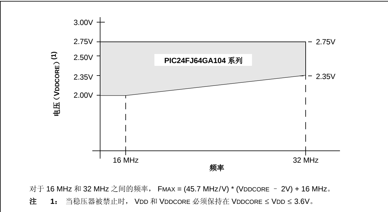
图 28-1: PIC24FJ64GA104 系列电压——频率关系图（工业级温度）
