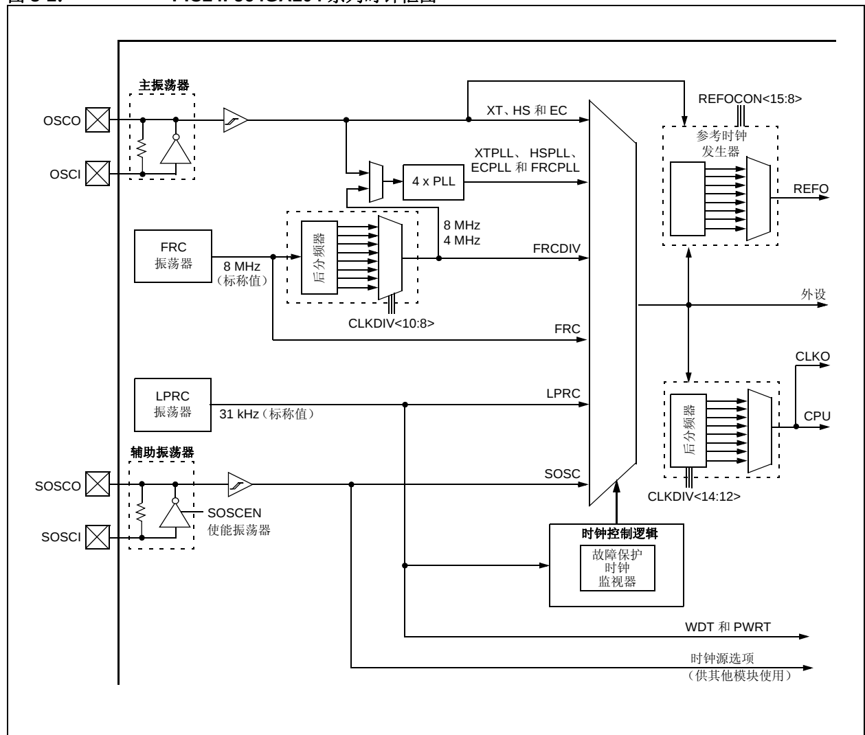
图 8-1: PIC24FJ64GA104 系列时钟框图
