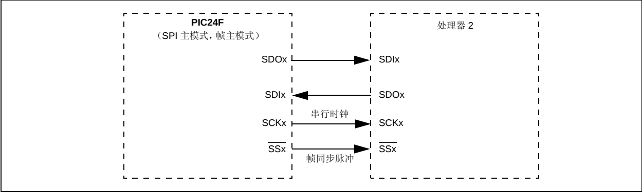
图 15-5: SPI 主 - 帧主模式连接图
