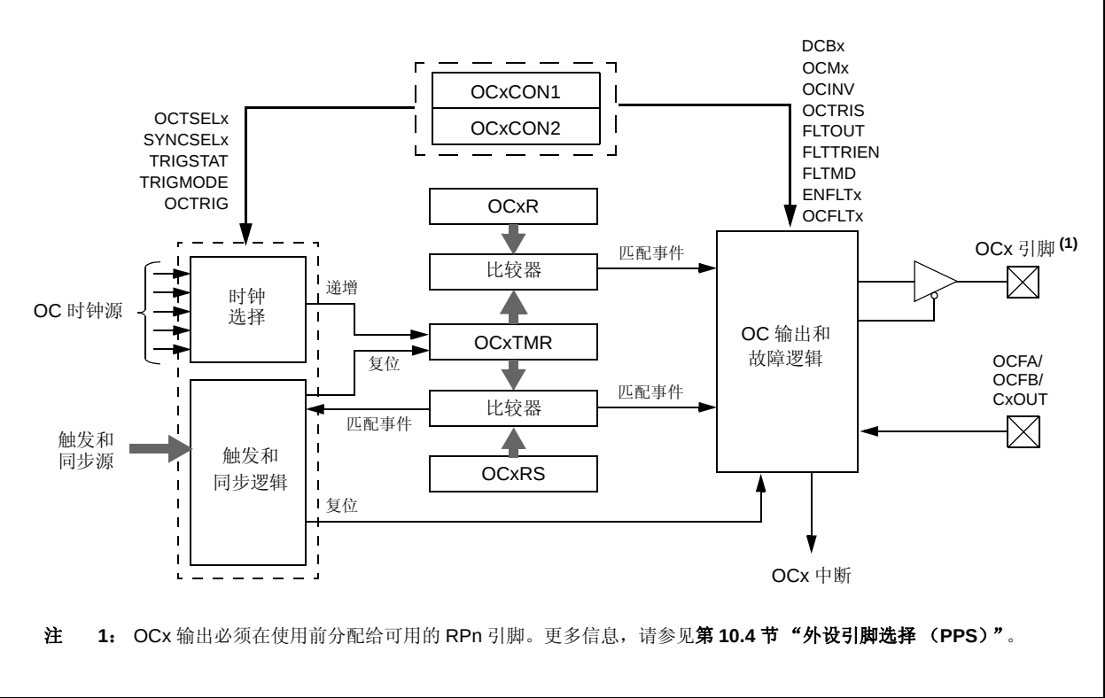
图 14-1: 输出比较框图 (16 位模式)
