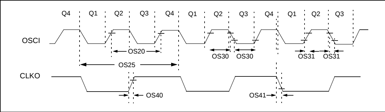
图 28-4: 外部时钟时序
