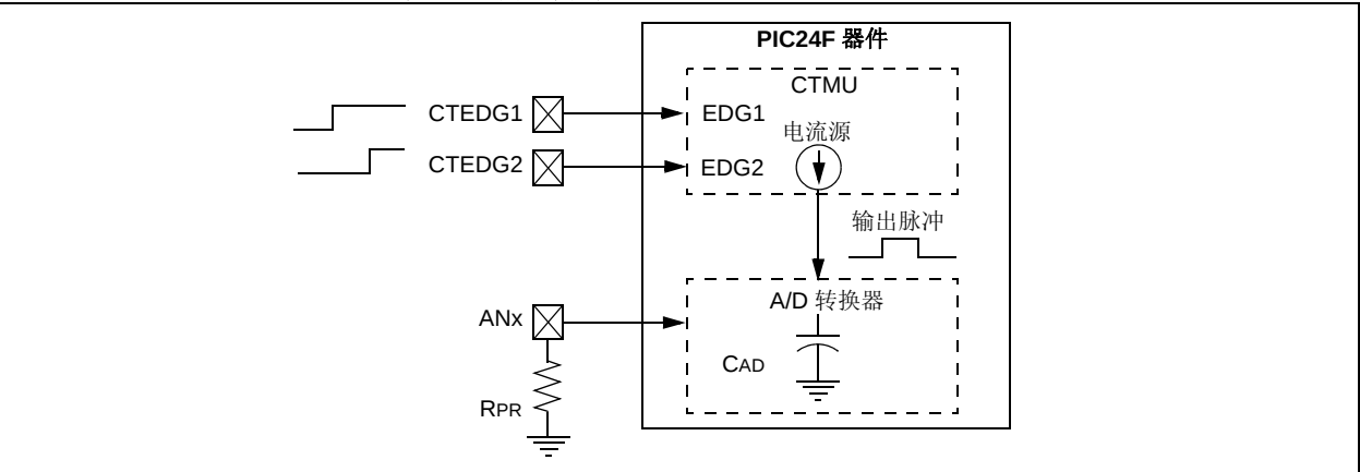
图 24-2: 时间测量的典型连接和内部配置
