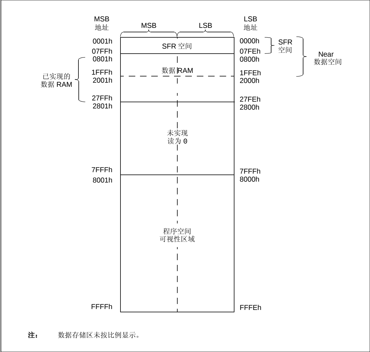
图 4-3: PIC24FJ64GA104 系列器件的数据存储空间映射
