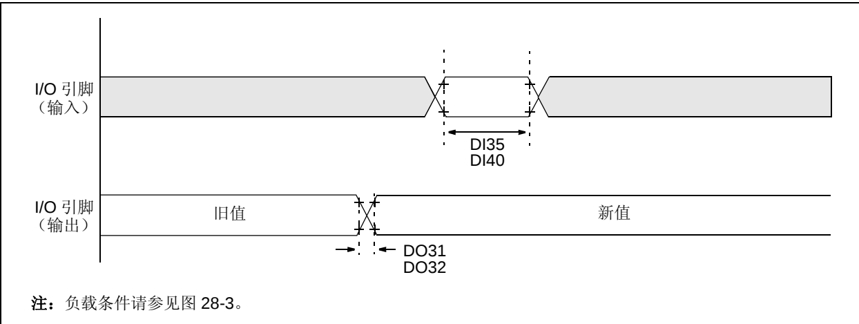
图 28-5: CLKO 和 I/O 时序特性
