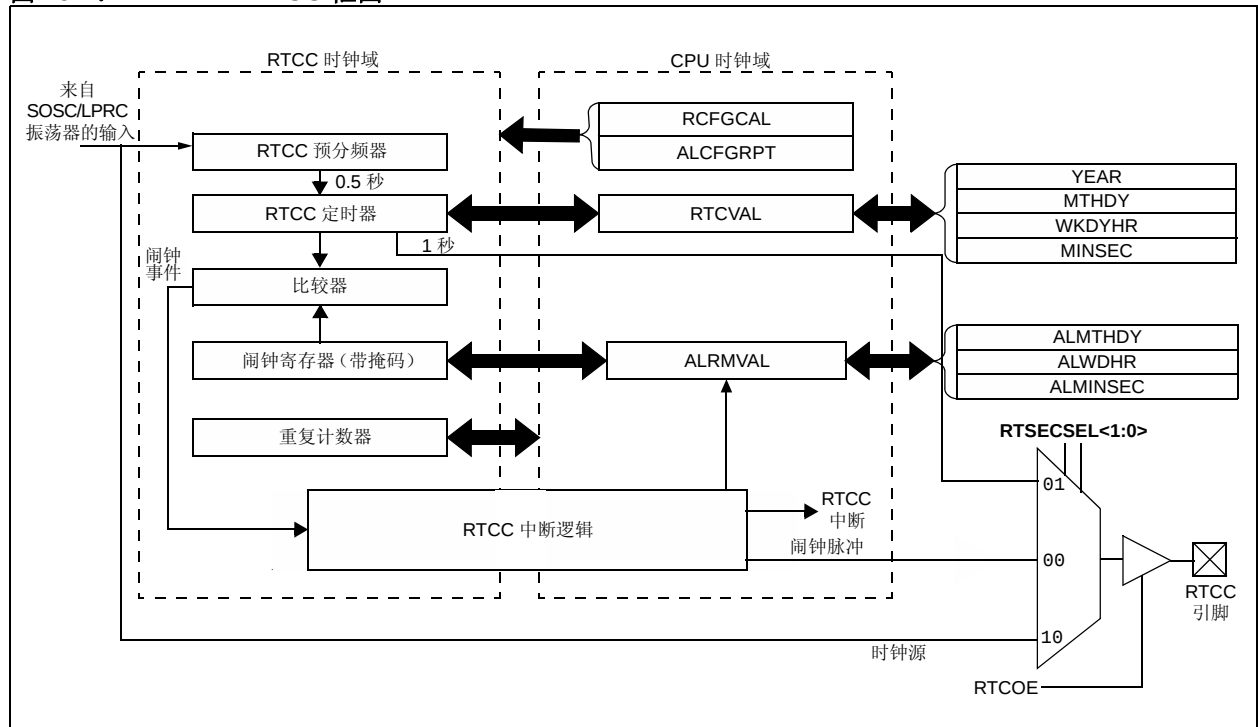
图 19-1: RTCC 框图
