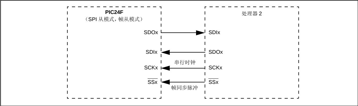
图 15-8: SPI 从 - 帧从模式连接图
