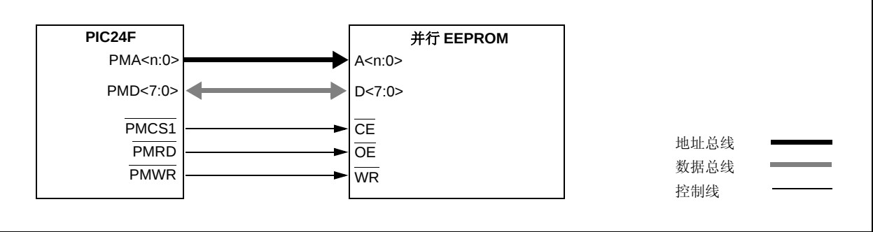
图 18-10: 并行 EEPROM 示例（最多 11 位地址，8 位数据）
