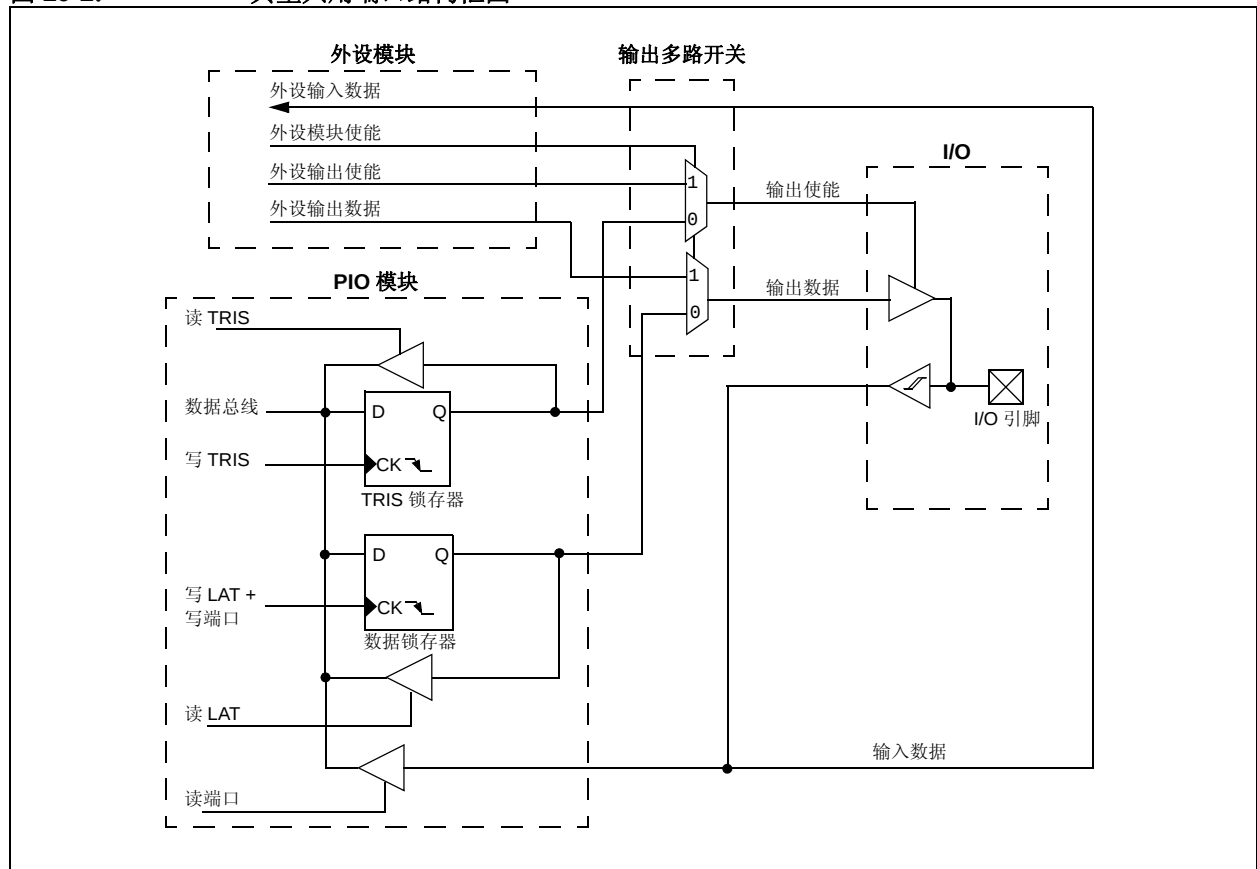
图 10-1: 典型共用端口结构框图
