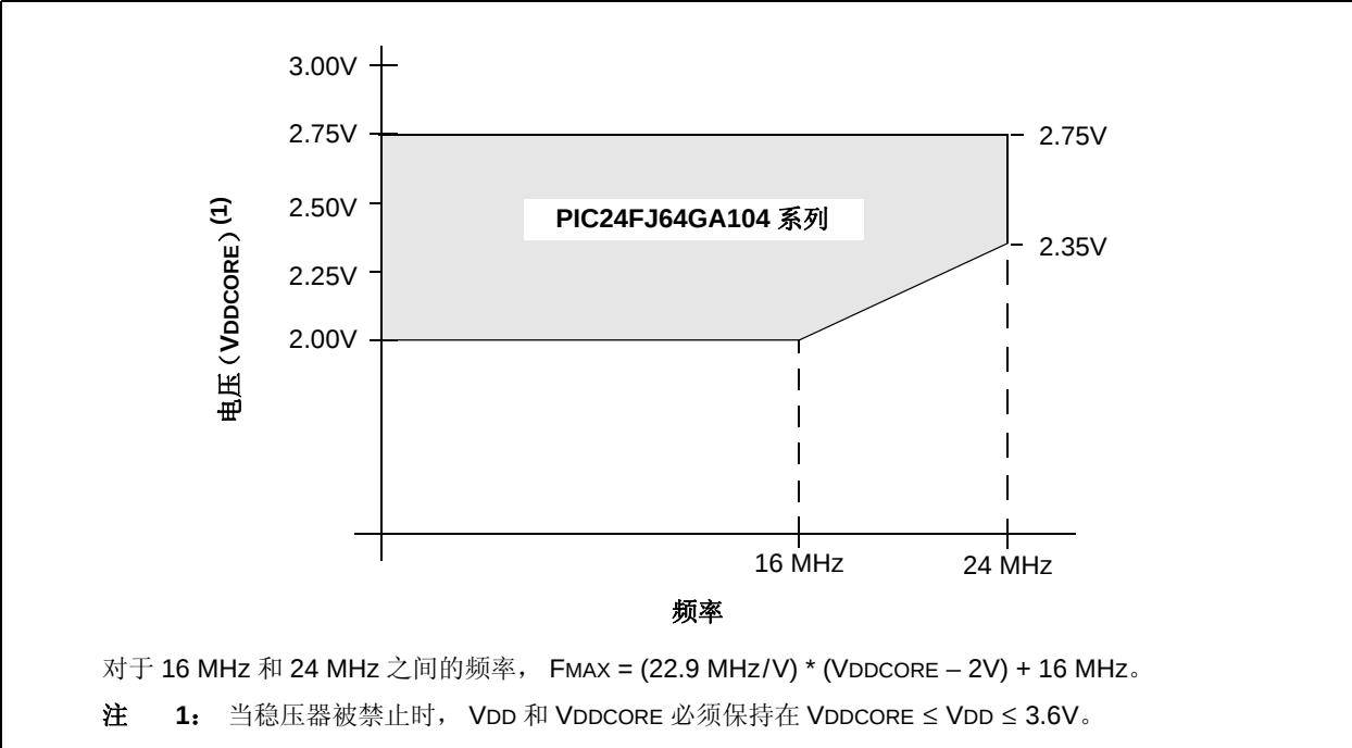
图 28-2: PIC24FJ64GA104 系列电压——频率关系图（工业级）（扩展级温度）
