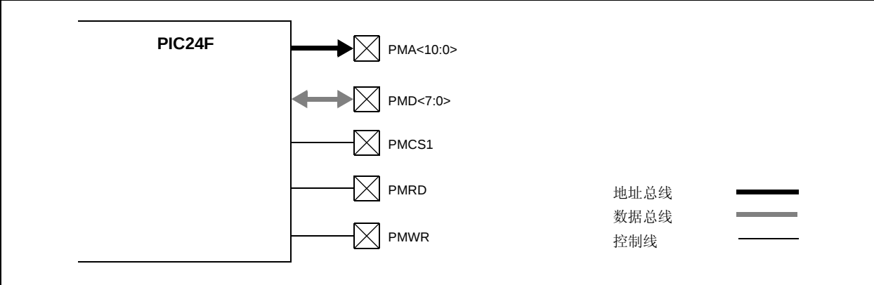
图 18-4: 主模式，解复用的寻址（独立的读和写选通，单片选）
