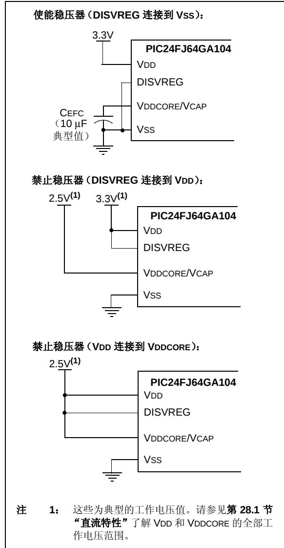
图 25-1: 片上稳压器的连接
