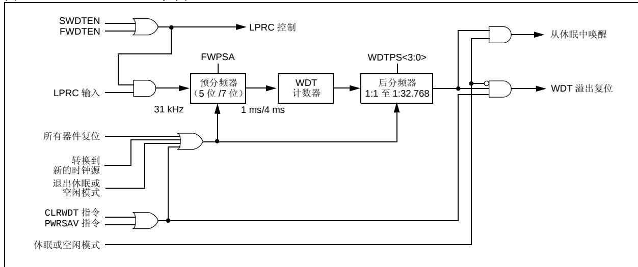
图 25-2: WDT 框图
