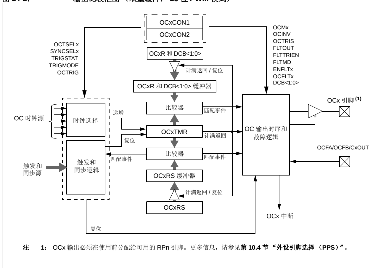
图 14-2: 输出比较框图（双重缓冲，16 位 PWM 模式）
