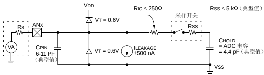
图 21-2: 10 位 A/D 转换器模拟输入模型
