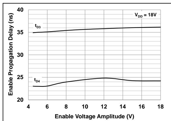
图 2-11: 使能传播延时 — 使能电压幅值曲线
