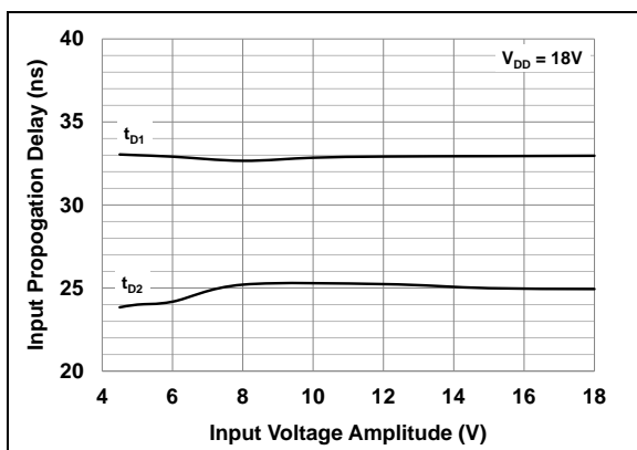
图 2-8: 输入传播延时 — 输入幅值曲线
