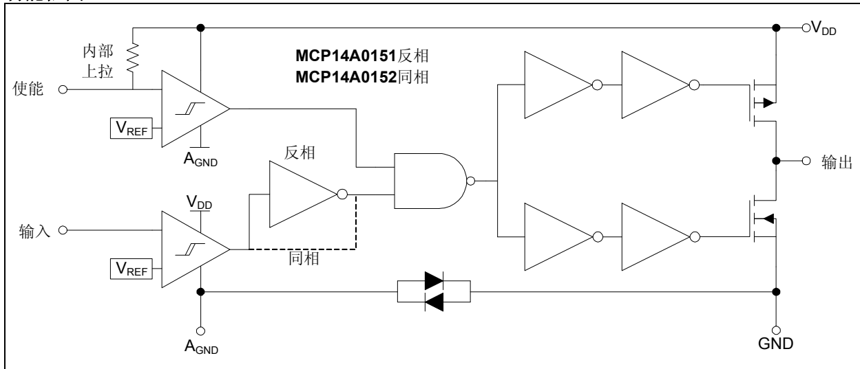
功能框图
