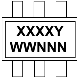
6 引脚 SOT-23
