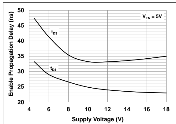
图 2-10: 使能传播延时 — 电源电压曲线
