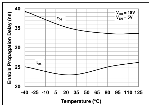
图 2-12: 使能传播延时 — 温度曲线
