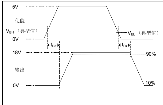
图 4-3: 使能时序波形
