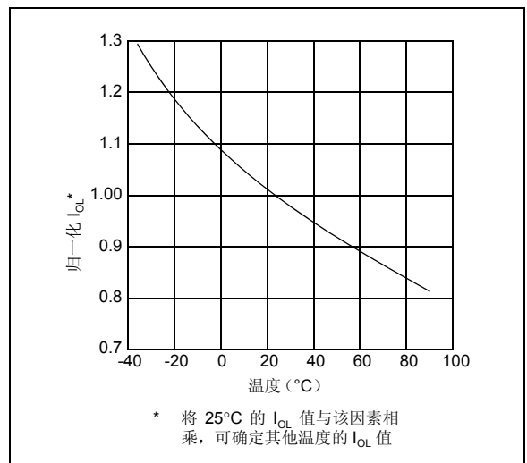
图 2-7: 归一化 I_{OL} —温度曲线
