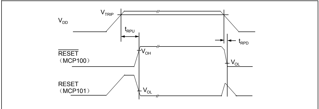
图 1-1: MCP100/101 时序图
