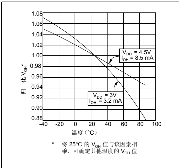
图 2-9: 归一化 V_{OH} - 温度曲线
