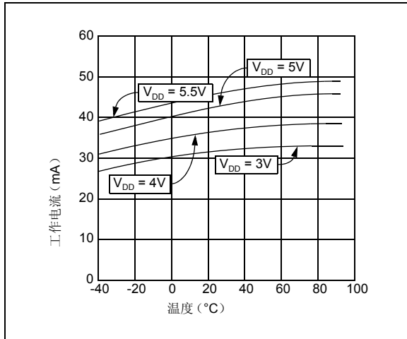
图 2-4: I_{DD} —温度曲线
