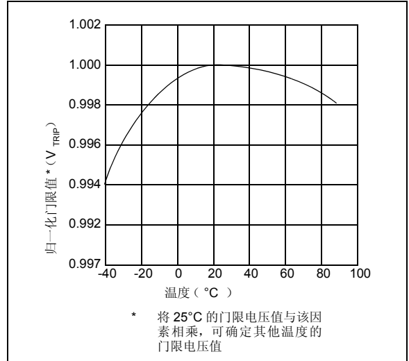
图 2-5: 归一化 V_{TRIP} —温度曲线
