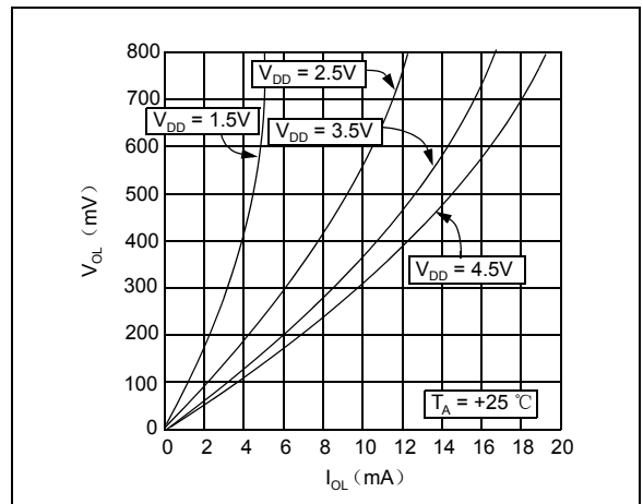
图 2-6: V_{OL} — I_{OL} 曲线
