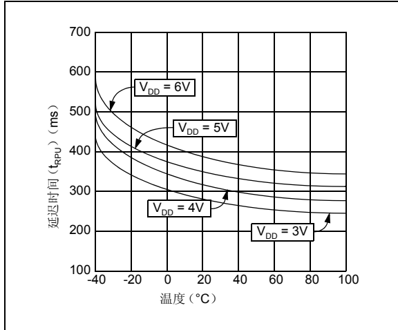
图 2-3: 典型 t_{RPU} —温度曲线
