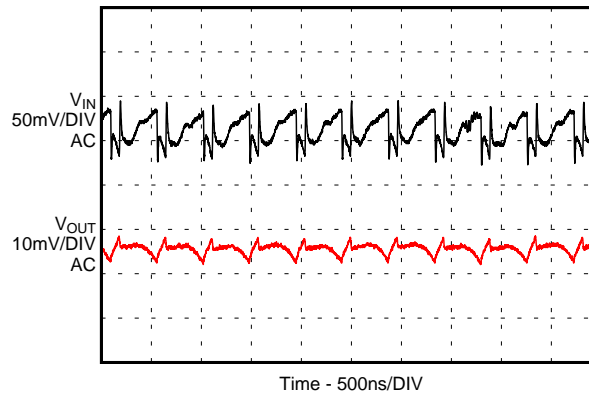
图 21. Switching Frequency
