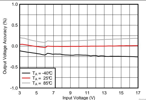
图 20. Line Regulation
