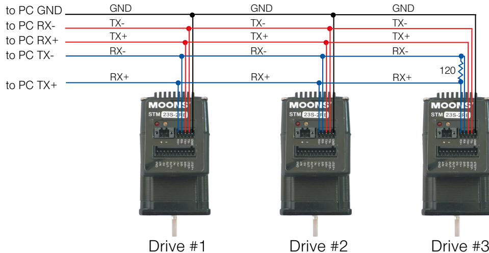
RS-485四线接线说明图
