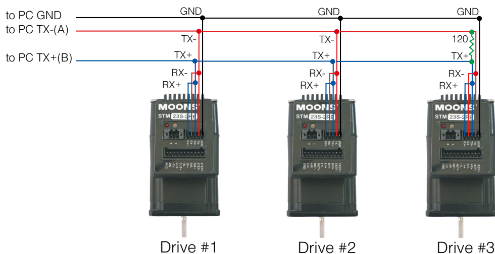
RS-485两线接线说明图
