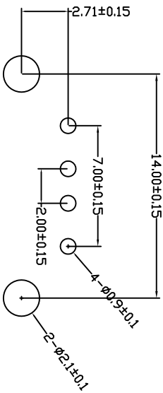
RBCOMMENDBD P.C.B PATTBRN LAYD UT
