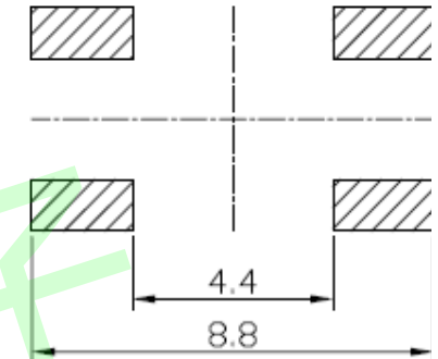
P.C.B LAND PATTE
