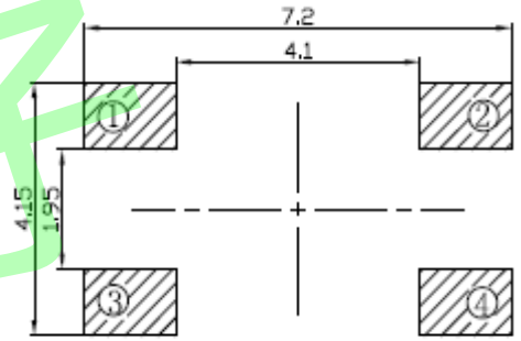
安装参考图
