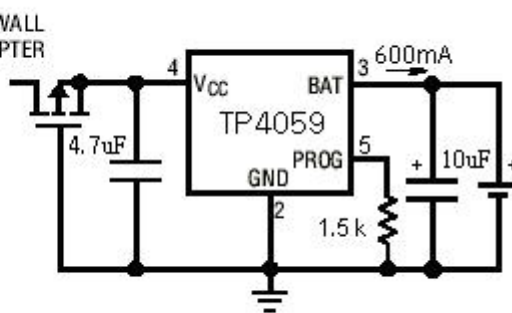
具有输入反向极性保护的充电器
