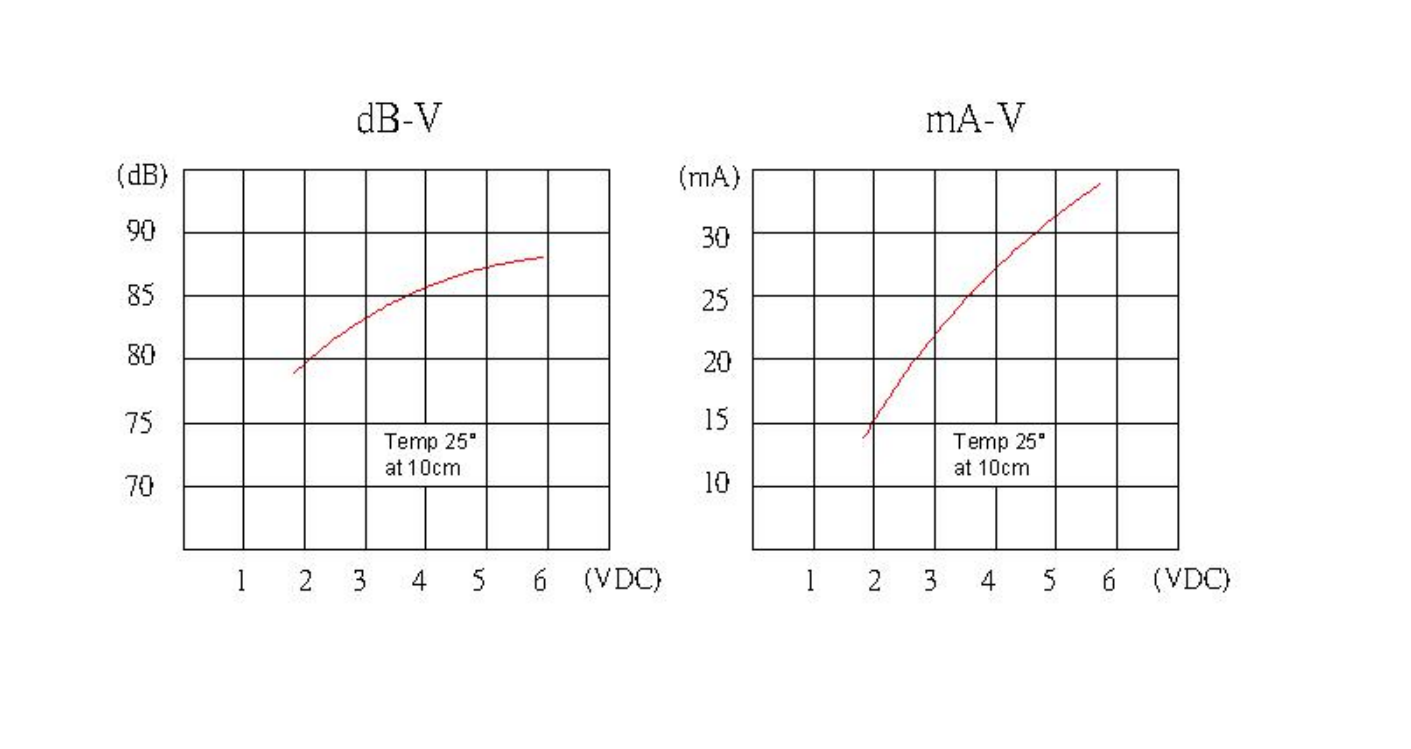
产品电流图
