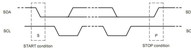
图 7: 起始和停止条件示意图
