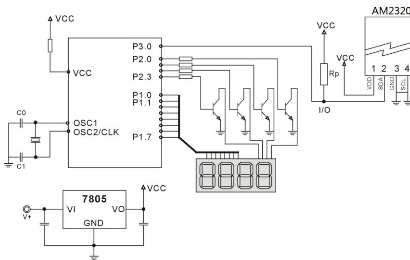
图 19: AM2320 单总线典型电路
