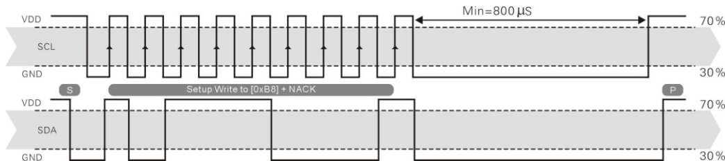
图 15: 唤醒传感器
