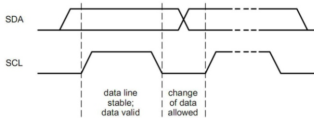
图 6: I 2 C 总线的位传输
