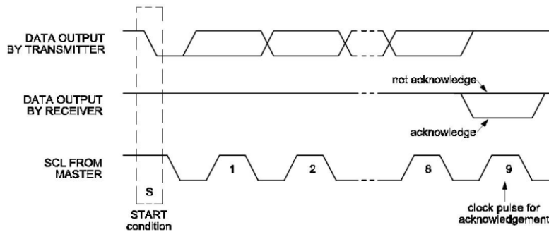
图 9： I 2 C 总线的响应
