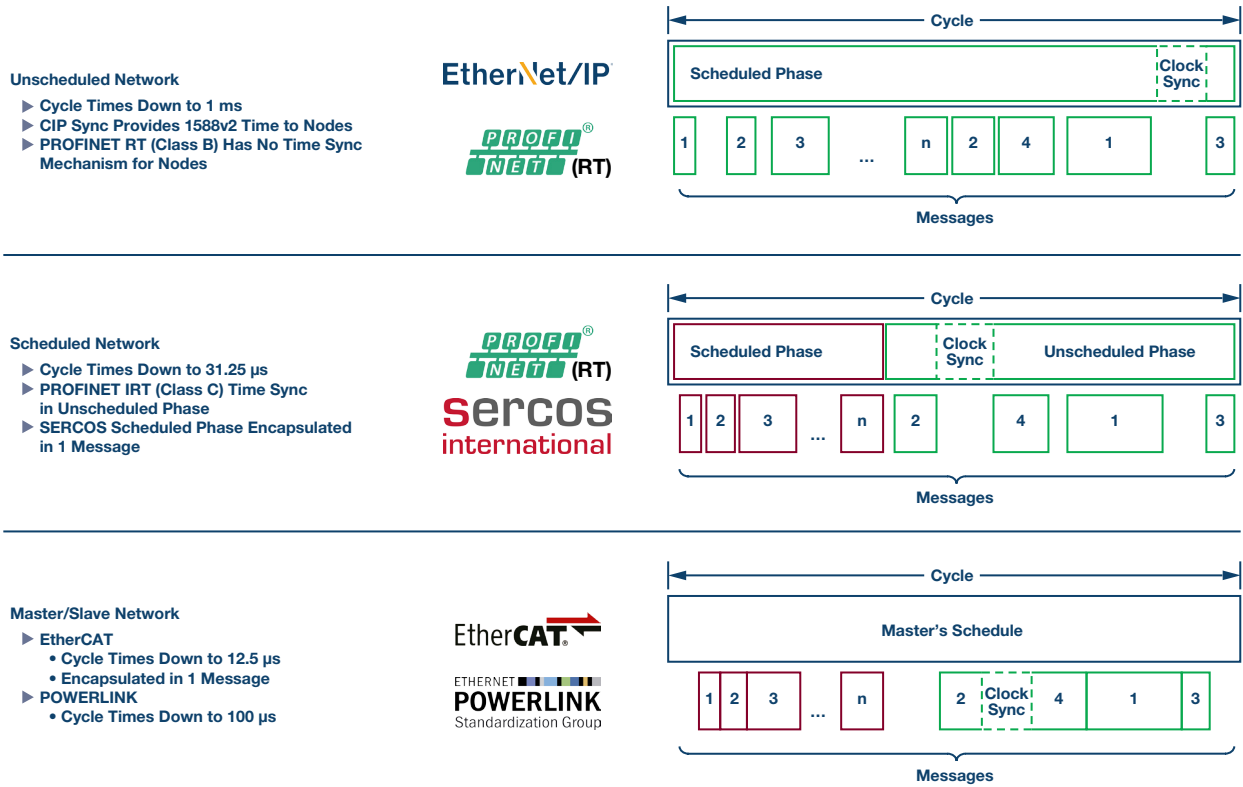
图3. 协议概述。
