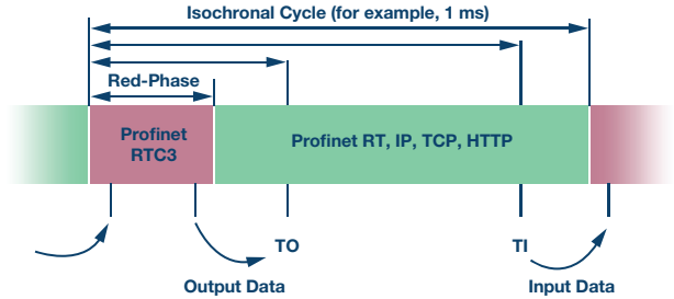
图4. PROFINET IRT。
