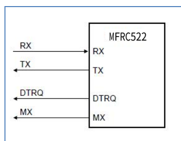
图 4 使用 UART 接口连接到微控制器
