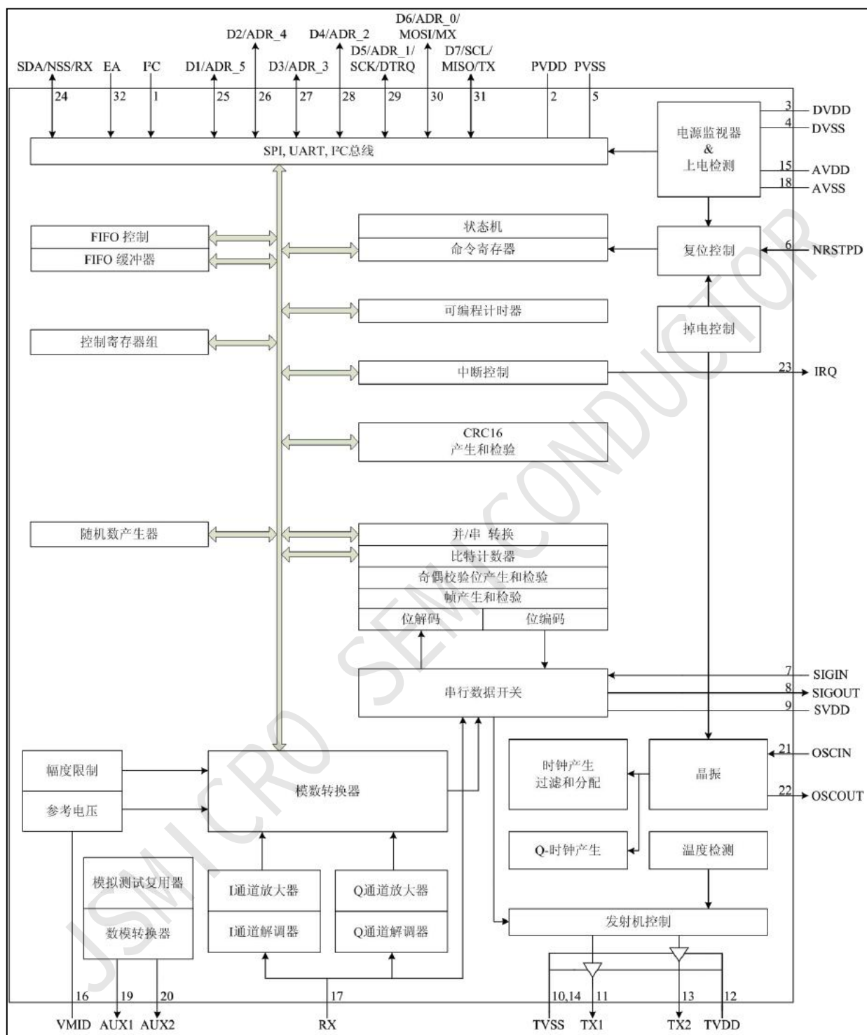
图 2 功能框图
