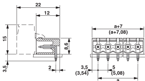
尺寸图
