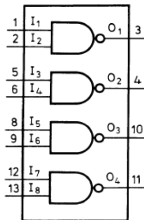
图 1 功能框图
