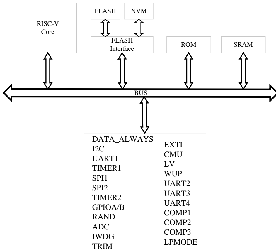
图 2-1 系统架构
