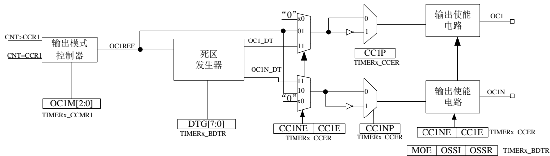
图 9-22 捕获/比较通道的输出部分
