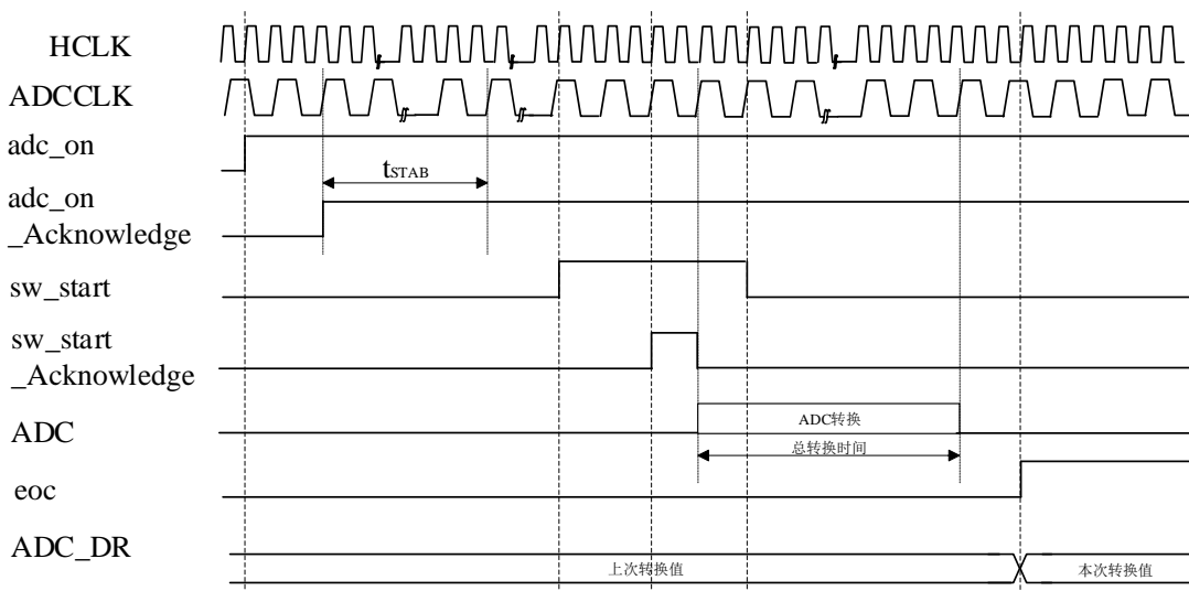
图 11-2 ADC 时序图
