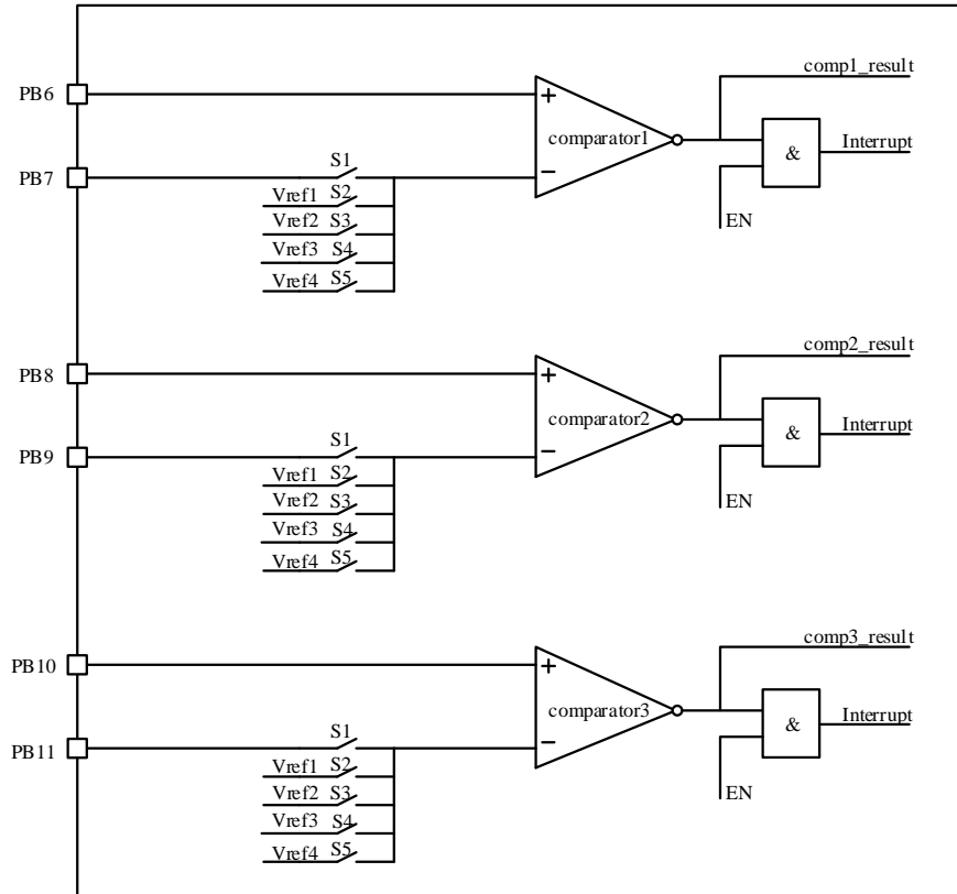
图 18-1 比较器框图
