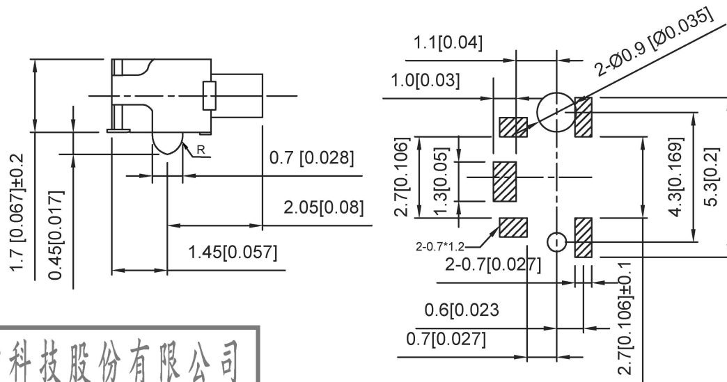
P.C.B LAYOUT
