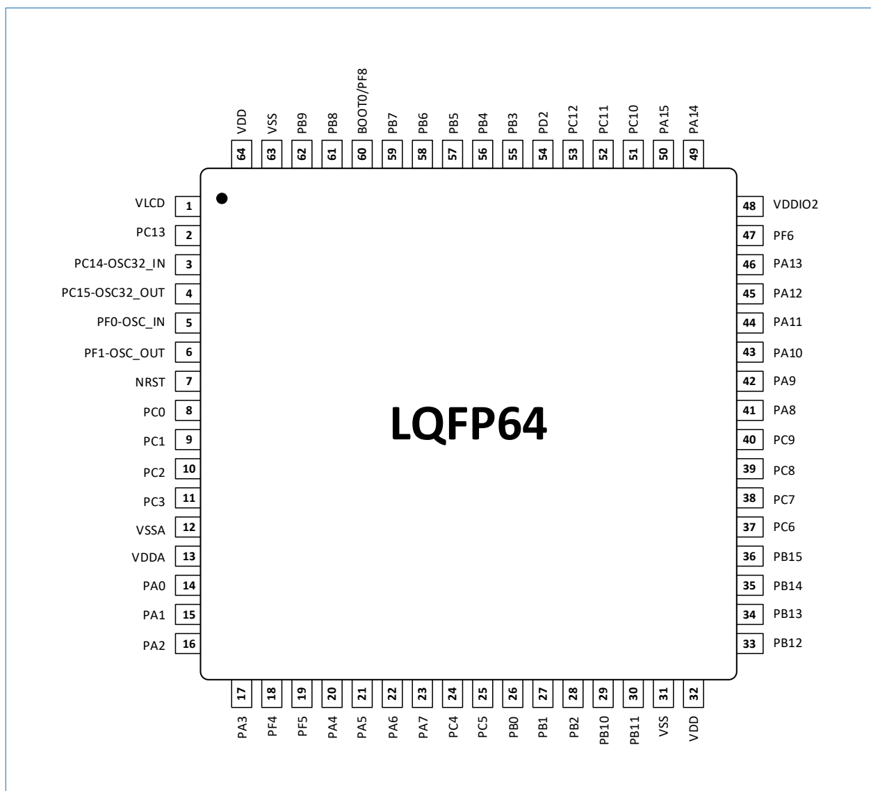
图 6-1 LQFP64 封装引脚排列
