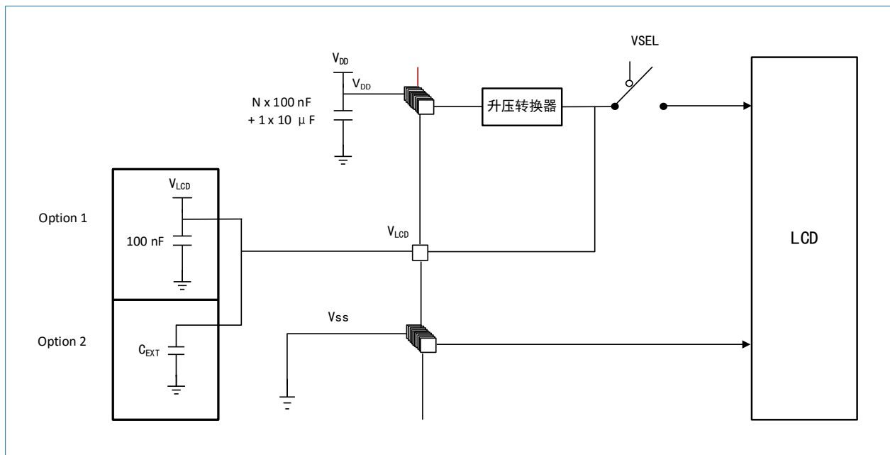
图 5-1 电源框图
