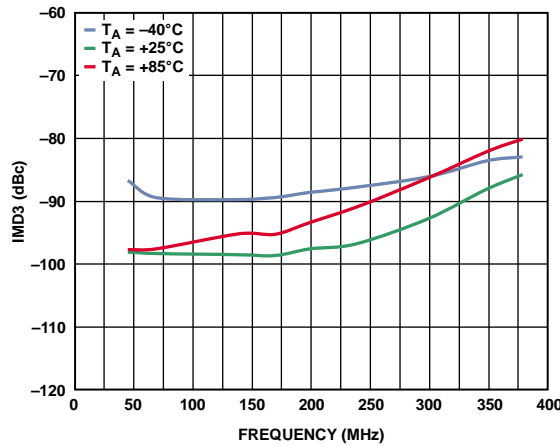
图29. 双音输出IMD3与频率的关系 (三种温度, 低功耗模式)
