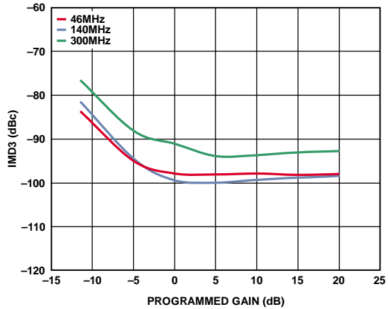
图26. 双音输出IMD3与编程增益的关系 (46 MHz、140 MHz和300 MHz, 低功耗模式)
