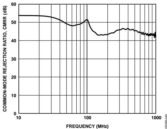
图45. 共模抑制比与频率的关系
