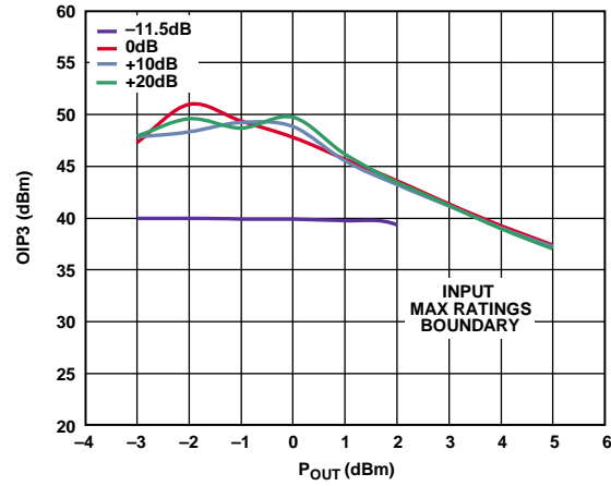
图27. 输出三阶交调截点与功率的关系 (四种增益代码, 频率 = 140 MHz, 低功耗模式)
