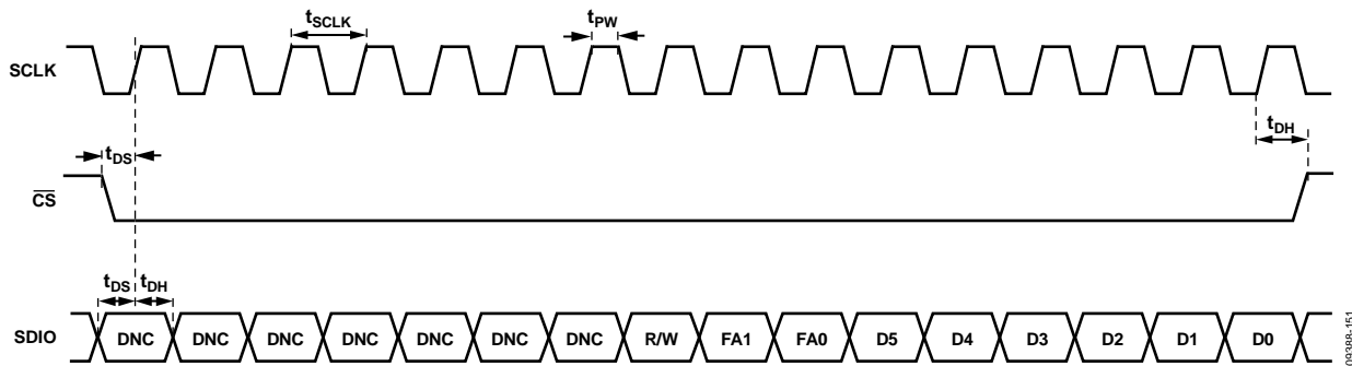
图51. SPI接口读/写模式时序图
