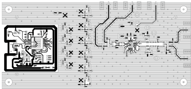
图62. 顶层
