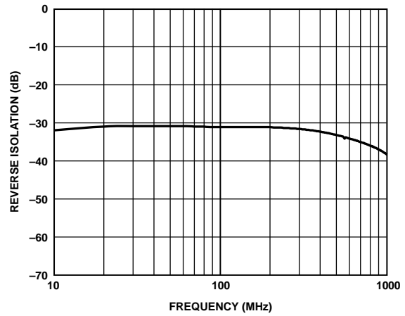
图41. 反向隔离与频率的关系
