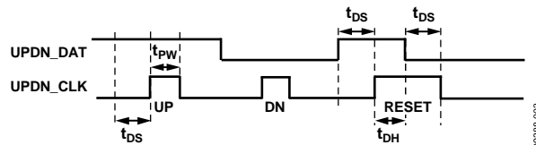
图3. 升降模式时序图
