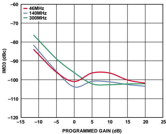
图14. 双音输出IMD3与编程增益的关系 (46 MHz、140 MHz和300 MHz)
