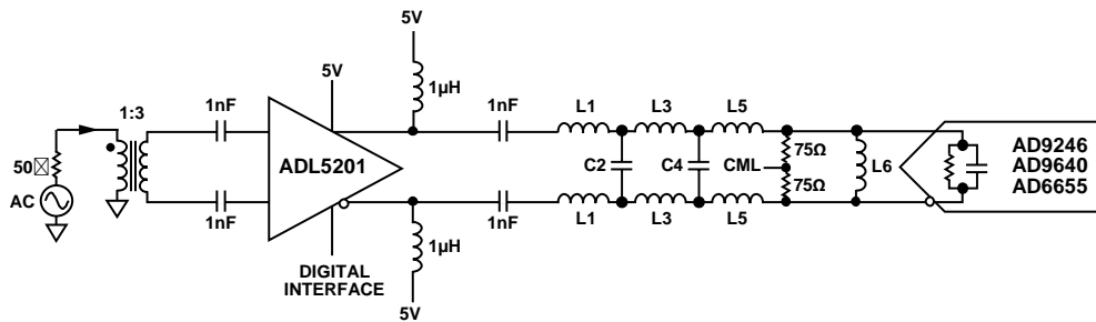
图58. 无缓冲ADC应用的窄带IF采样解决方案
