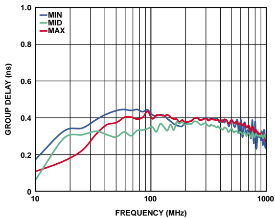
图42. 群延迟与频率的关系(最大、中等、最小增益输出)
