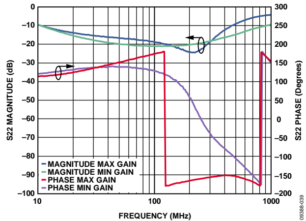
图40. S22幅度和相位与频率的关系
