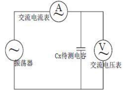
图 3. 交流阻抗测试电路图
