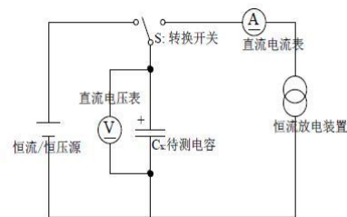
图 1. 容量测试电路
