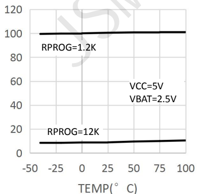
涓流充电电流与温度的关系曲线
