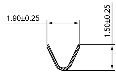
SEC:B-B
