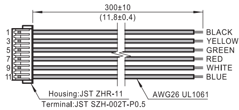
6 线零件号 4634 1402 04489
