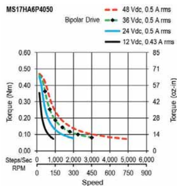
MS17HA6-0.9° 双极性
