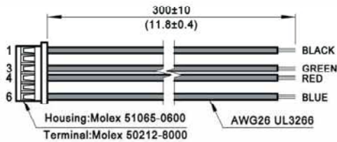
4 线零件 4634140204190
