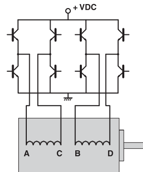
2 相(双极性)步进电机
