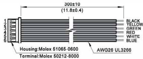
6 线零件 4634140204490
