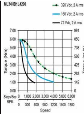
ML34HD1
