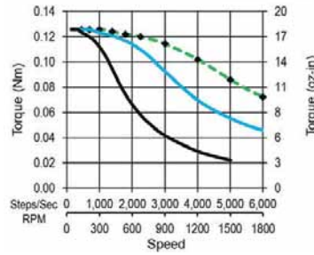
MS16HS0P6070 Unipolar Drive 36 Vdc, 0.7 A rms 24 Vdc, 0.7 A rms 12 Vdc, 0.7 A rms
