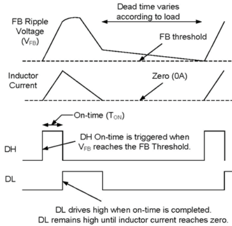
Fig. 6 - Power-Save Mode
