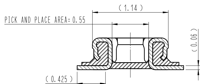
A-A (30:1)
