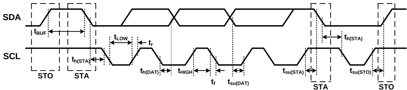
图 1. I²C Timing
