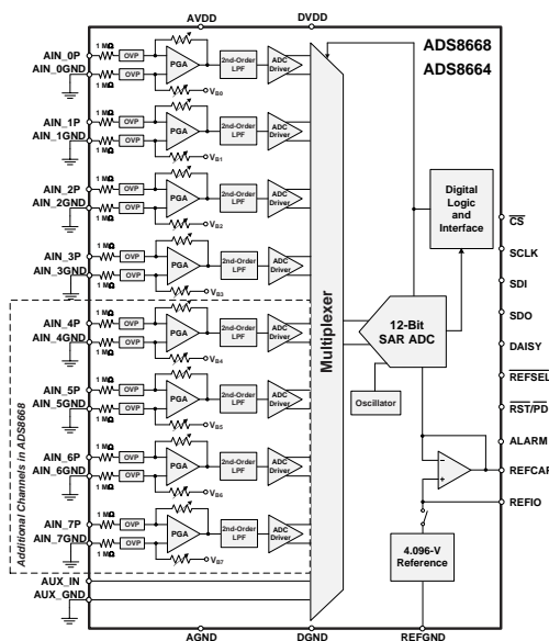
框图
