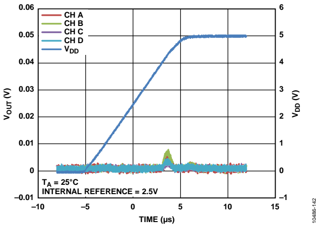
图36. 上电复位至0 V
