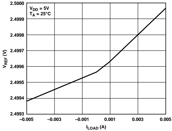
图11. 内部基准电压与负载电流的关系
