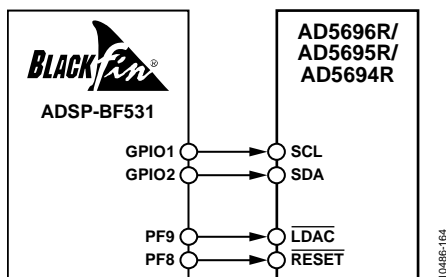
图58. ADSP-BF531接口
