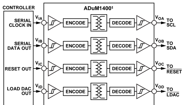
图60. 隔离接口
