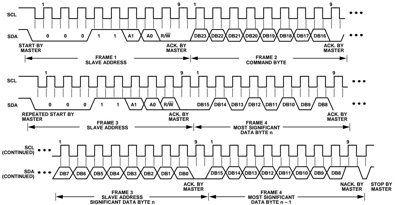
图52. PC读操作
