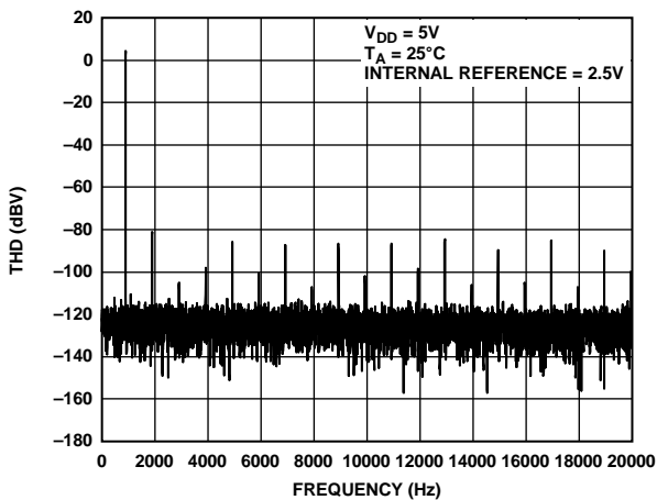
图43. 1 kHz时的总谐波失真
