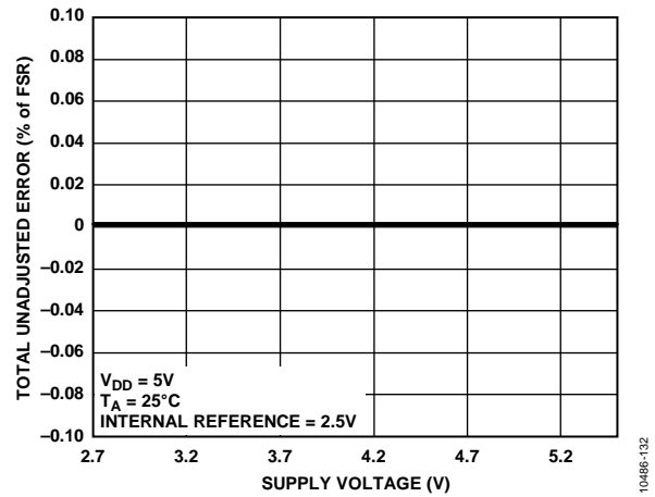
图27. TUE与电源的关系(增益=1)
