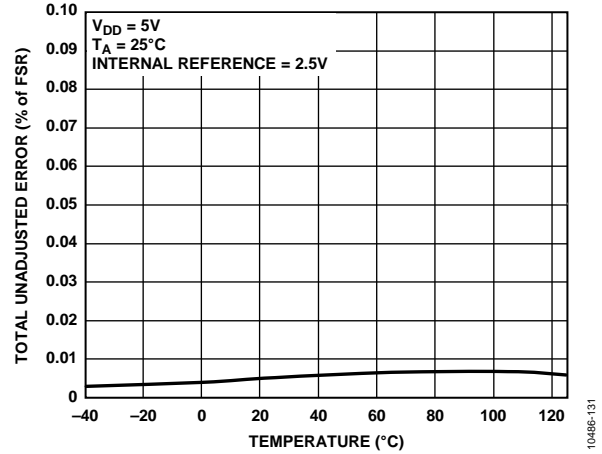
图26. TUE与温度的关系
