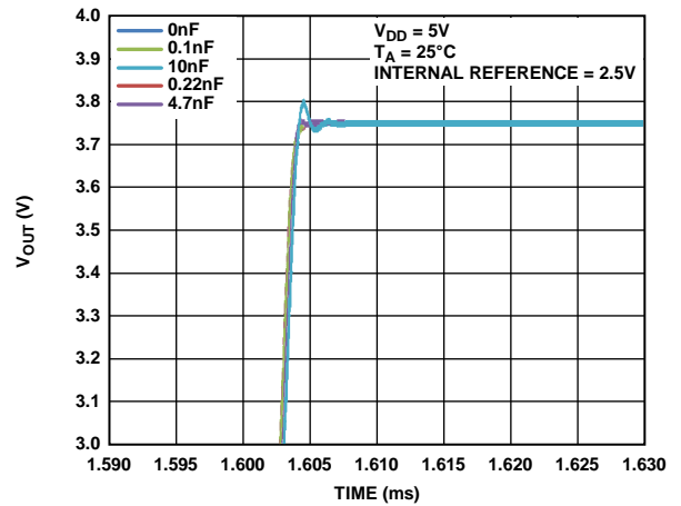
图44. 建立时间与容性负载的关系
