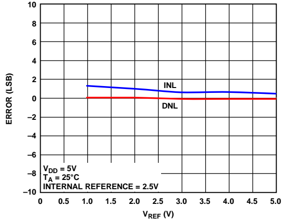
图20. INL误差和DNL误差与 V_{REF} 的关系
