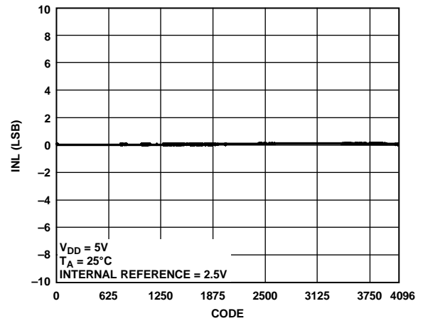
图15. AD5694R INL
