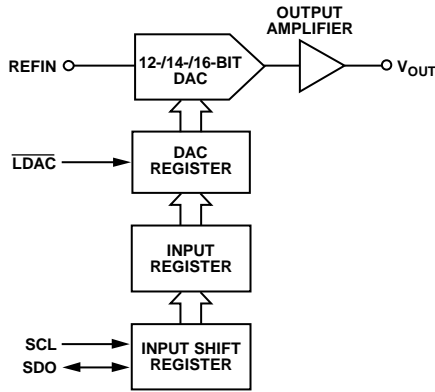
图54. 单个DAC的输入加载电路示意图
