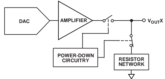
图53. 掉电模式下的输出级
