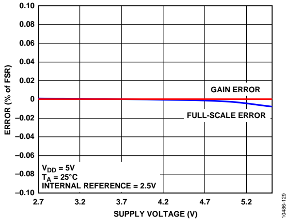
图24. 增益误差和满量程误差与电源的关系
