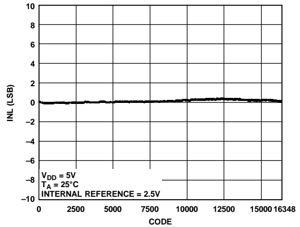
图14. AD5695R INL
