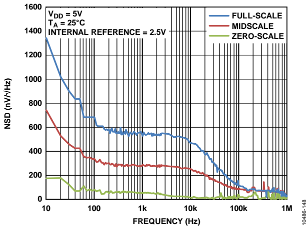
图42. 噪声频谱密度
