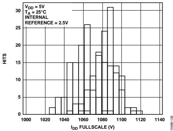
图30. 采用内部基准电压源时的 I_{DD} 直方图( V_{REFOUT} = 2.5 V , 增益 = 2)
