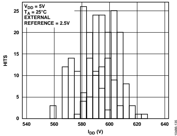
图29. 采用外部基准电压源时的 I_{DD} 直方图(5 V)
