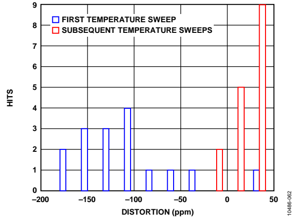
图57. 热滞
