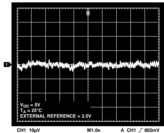
图40. 0.1 Hz至10 Hz输出噪声图, 外部基准电压源
