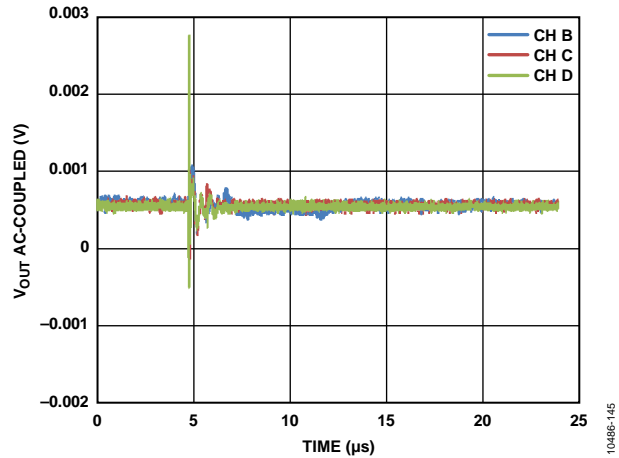
图39. 模拟串扰(通道A)
