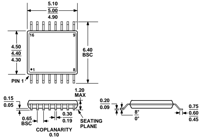
图62. 16引脚超薄紧缩小型封装[TSSOP] (RU-16) 尺寸单位: mm
