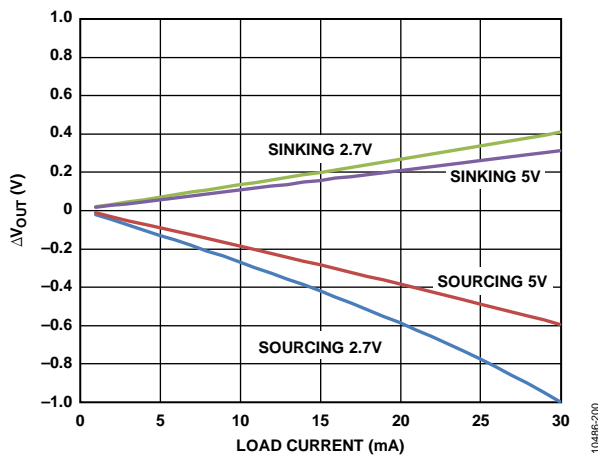
图31. 上裕量/下裕量与负载电流的关系
