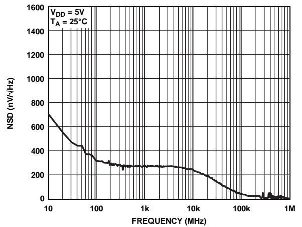
图9. 内部基准电压源噪声谱密度与频率的关系
