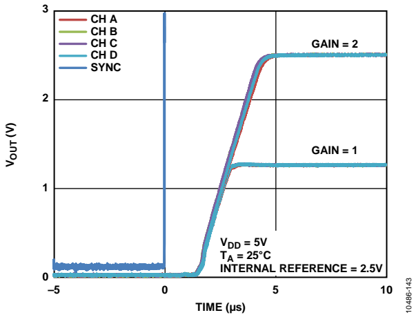
图37. 退出掉电模式进入中间电平
