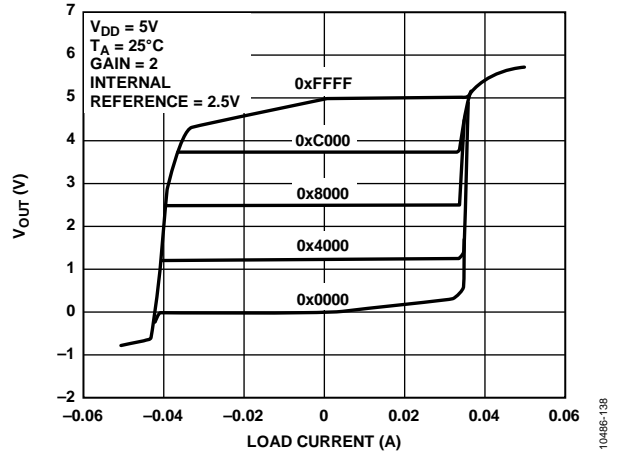
图32. 5 V时的源电流和吸电流能力
