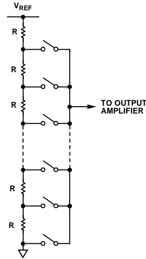
图47. 电阻串结构
