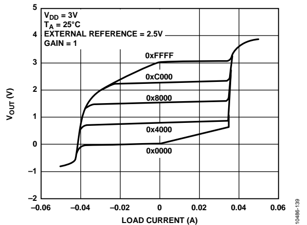
图33. 3 V时的源电流和吸电流能力
