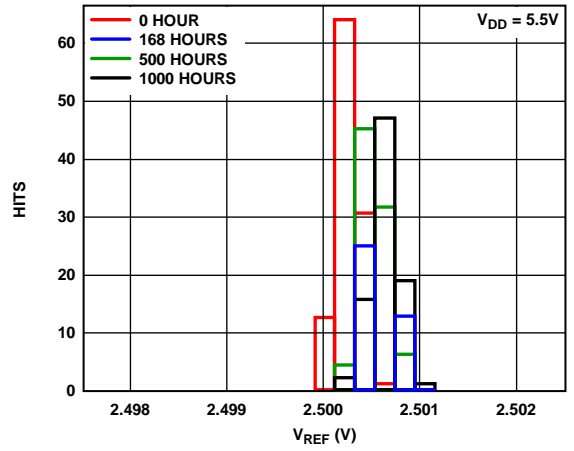
图8. 基准电压源长期稳定性/漂移
