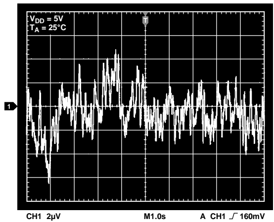
图10. 内部基准电压源噪声(0.1 Hz至10 Hz)
