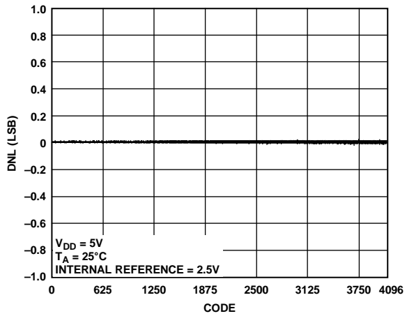
图18. AD5694R DNL
