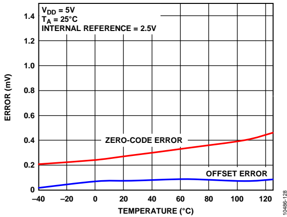
图23. 零代码误差和失调误差与温度的关系
