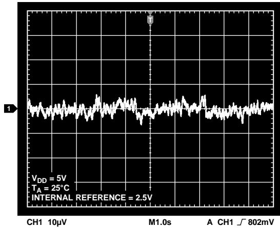
图41. 0.1 Hz至10 Hz输出噪声图, 2.5 V内部基准电压源
