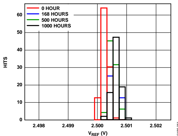
图56. 1000小时后的基准电压漂移
