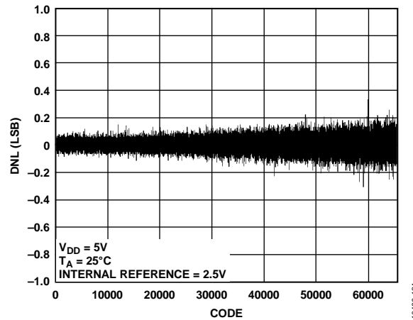
图16. AD5696R DNL
