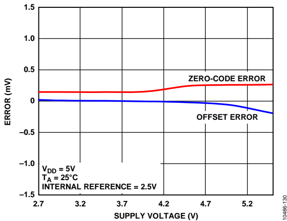
图25. 零代码误差和失调误差与电源的关系
