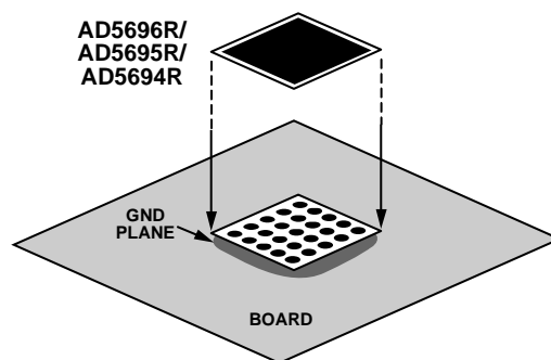
图59. 焊盘与电路板的连接
