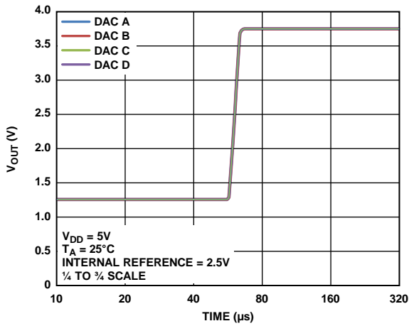
图35. 建立时间(5.25 V)
