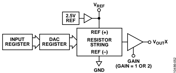
图46. DAC单通道架构框图
