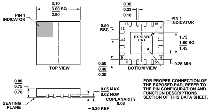
图61. 16引脚引脚架构芯片级封装[LFCSP_WQ] 3 mm x 3 mm, 超薄体 (CP-16-22) 尺寸单位: mm
