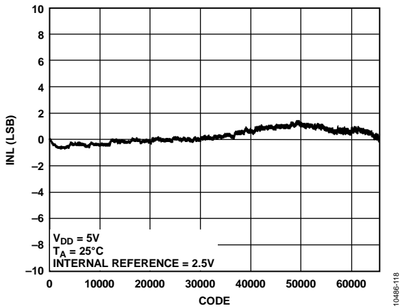
图13. AD5696R INL
