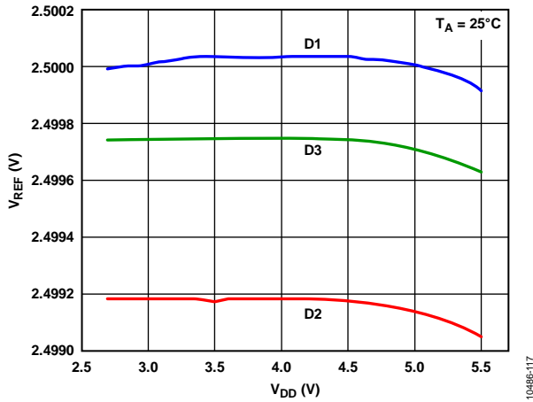
图12. 内部基准电压与电源电压的关系
