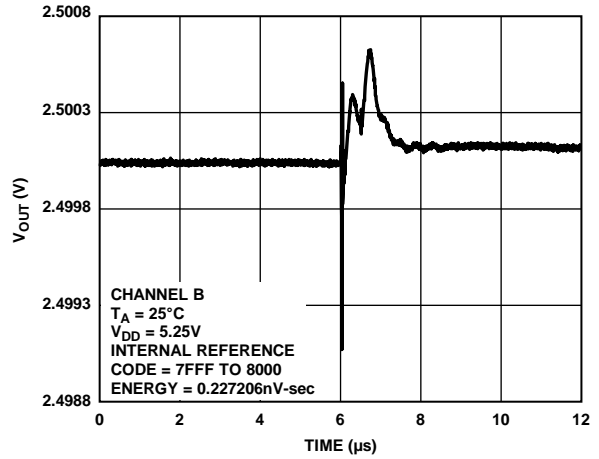
图38. 数模转换毛刺脉冲
