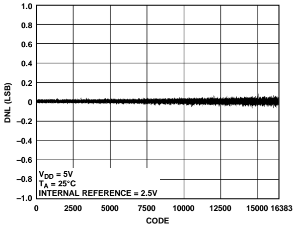
图17. AD5695R DNL
