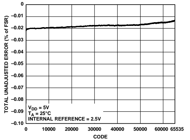
图28. TUE与代码的关系
