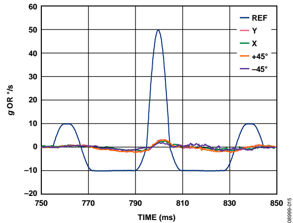
图15. 50 g、10 ms脉冲的g和g × g灵敏度
