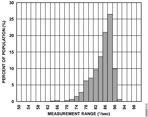
图10. 测量范围
