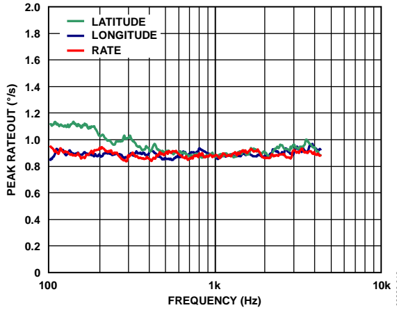
图16. 对10 g正弦振动的典型响应(传感器带宽 = 2 kHz)
