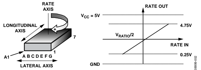
图2. 顺时针旋转时RATEOUT信号增大
