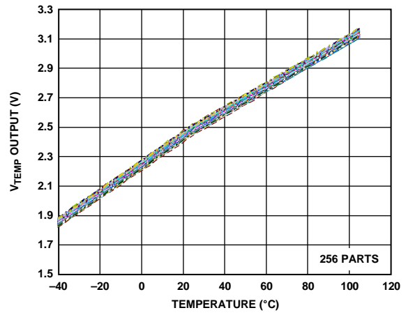
图14. 整个温度范围内的 V_{TEMP} 输出( V_{RATIO} = 5 V )
