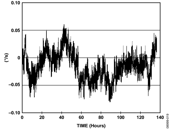
图19. 140小时内累积的90秒零点均值的典型偏移
