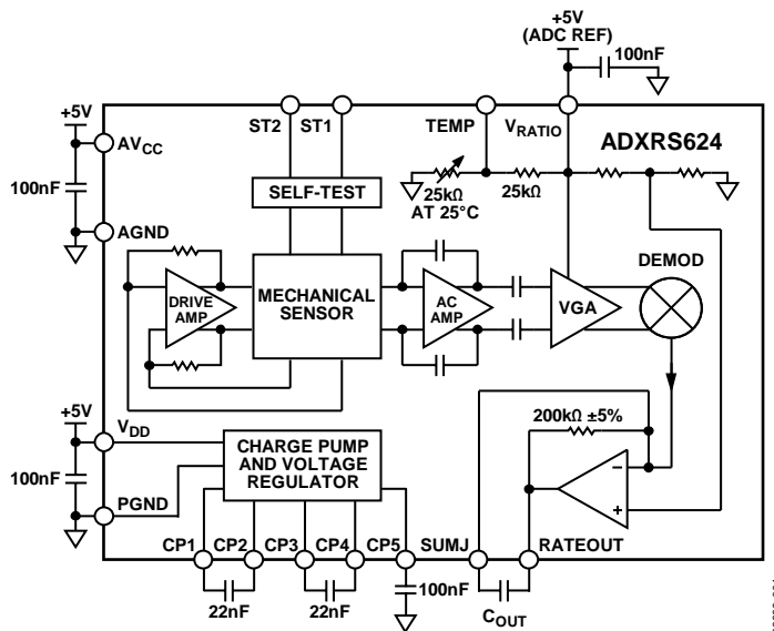
图1. ADXRS624框图
