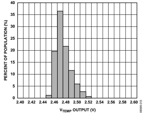
图13. 25°C时的 V_{TEMP} 输出( V_{RATIO} = 5 V )
