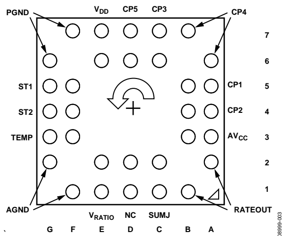
图3. 引脚配置
