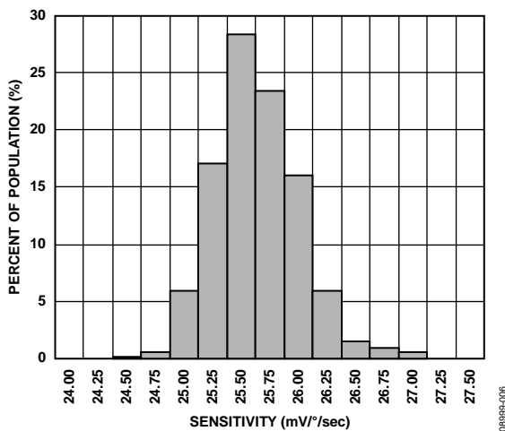
图6. 25°C时的灵敏度 ( V_{RATIO} = 5 V )
