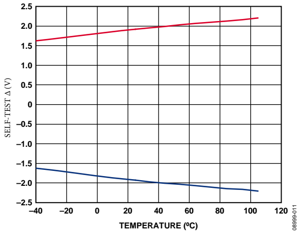
图11. 整个温度范围内的典型自测变化
