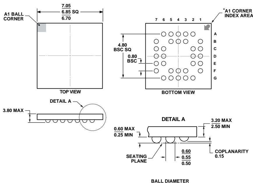
图24. 32引脚陶瓷球栅阵列封装[CBGA] (BG-32-3)
