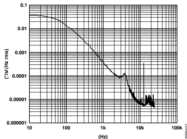
图22. 增加250 Hz滤波器后的噪声频谱密度
