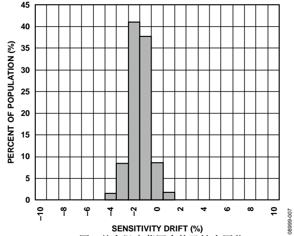
图7. 整个温度范围内的灵敏度漂移
