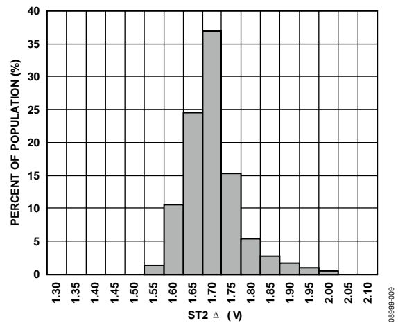
图9. 25°C时的ST2输出变化 ( V_{RATIO} = 5 V )
