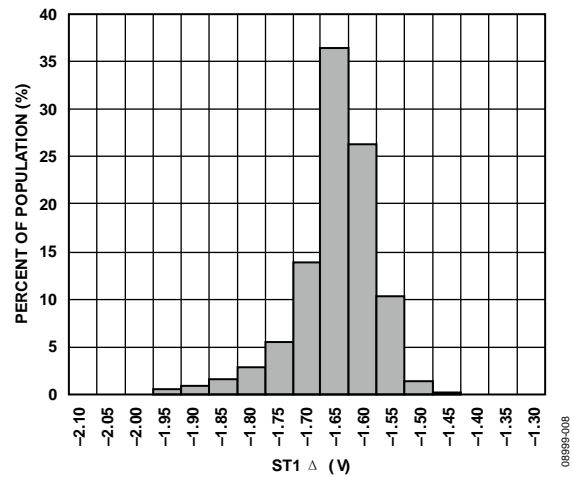
图8. 25°C时的ST1输出变化 ( V_{RATIO} = 5 V )
