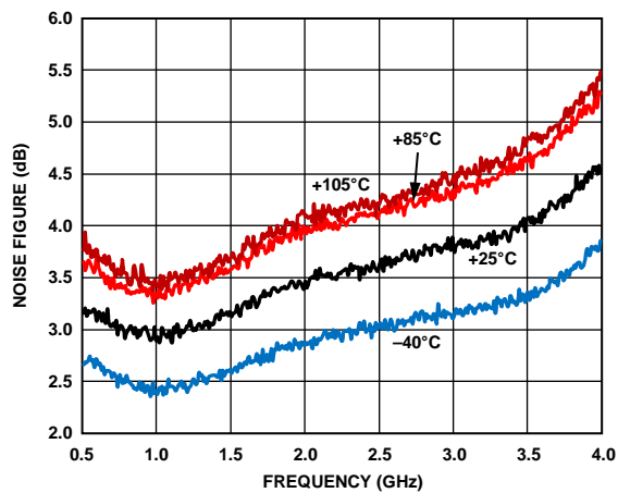
图8. 噪声系数与频率和温度的关系
