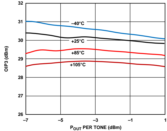
图37. 30 MHz时OIP3与 P_{OUT} 的关系
