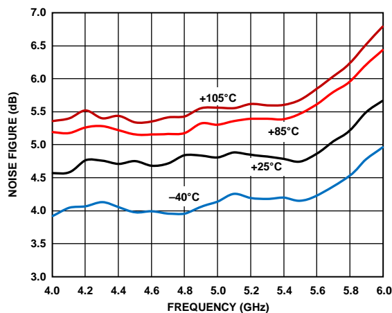
图20. 噪声系数与频率和温度、高频配置的关系
