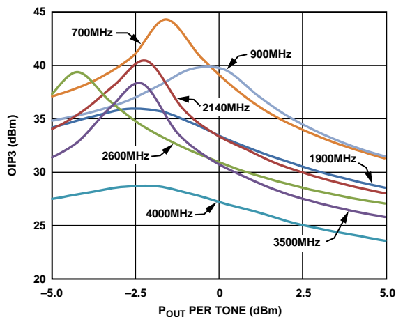
图6. OIP3与输出功率(P OUT )和频率的关系
