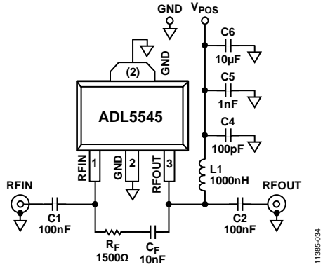
图34. 工作频率低至30 MHz的设置
