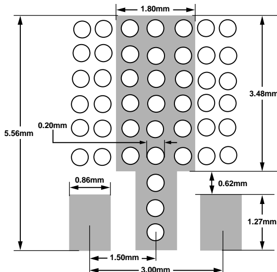
图33. 推荐焊盘图形
