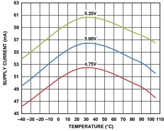
图21. 电源电流与温度的关系
