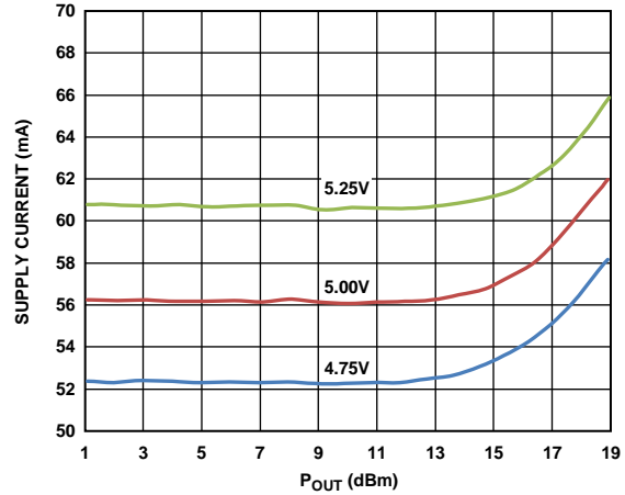
图24. 900 MHz时电源电流与P OUT 的关系
