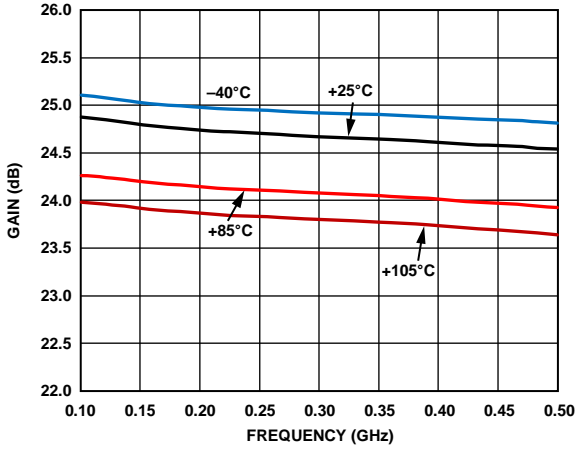
图10. 增益与频率和温度、低频配置的关系
