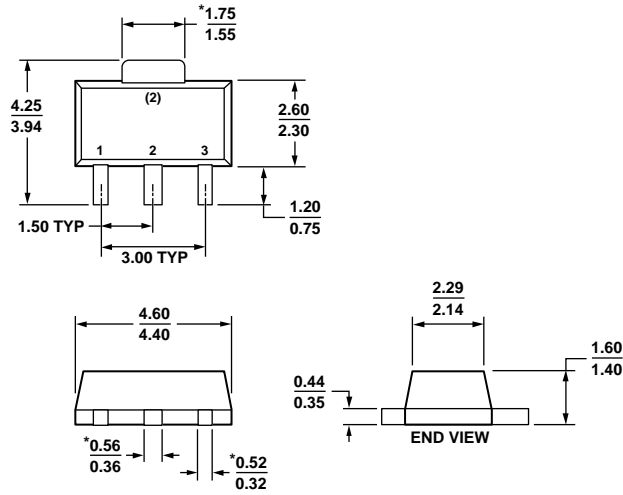
图41. 3引脚小型晶体管封装[SOT-89]
