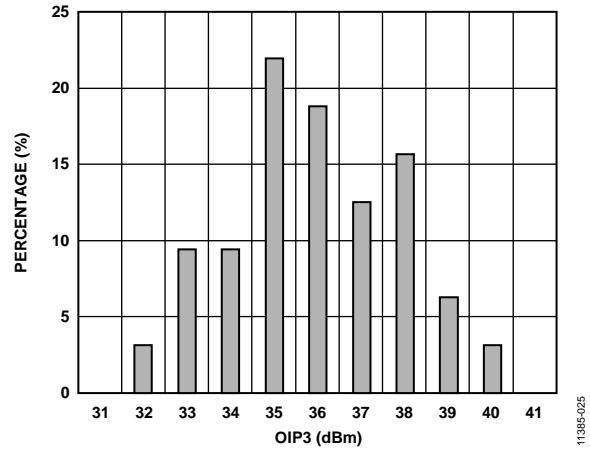
图25. 900 MHz时的OIP3分布(P OUT = -3 dBm/信号音)
