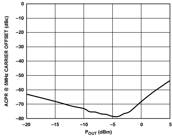
图38. ACPR与 P_{OUT} 的关系(2140 MHz时 W-CDMA单载波, 测试模型1-64)
