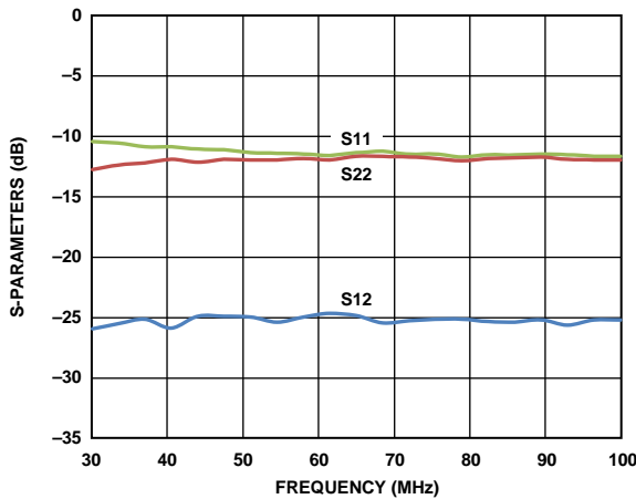
图36. 回损和反向隔离(30 MHz至100 MHz)
