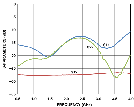
图7. 输入回损(S11)、输出回损(S22)和反向隔离(S12)与频率的关系
