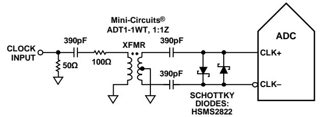
图35. 变压器耦合差分时钟(频率可达200 MHz)
