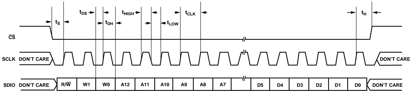
图58. 串行端口接口时序图
