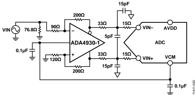
图30. 利用ADA4930-1进行差分输入配置
