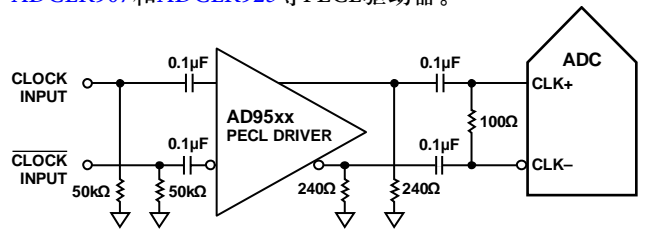
图37. 差分PECL采样时钟(频率可达625 MHz)
