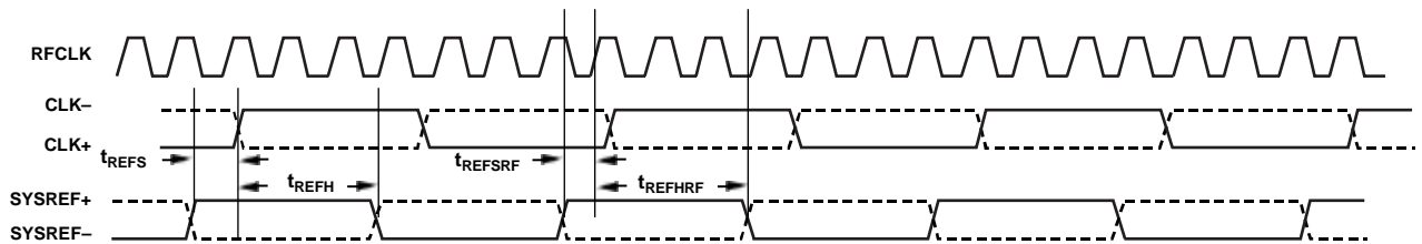
图3. SYSREF±建立和保持时间(时钟输入RFCLK或CLK±, 但不能同时)
