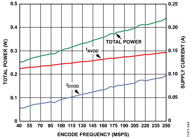
图44. 功耗与编码速率的关系
