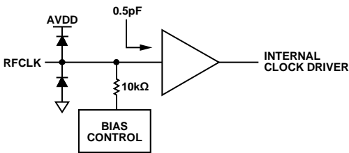
图22. 等效RF时钟输入电路
