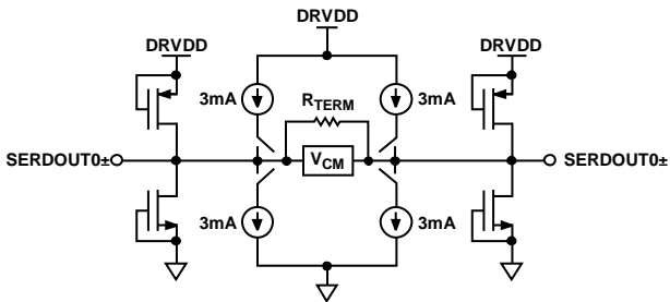
图21. 数字CML输出电路
