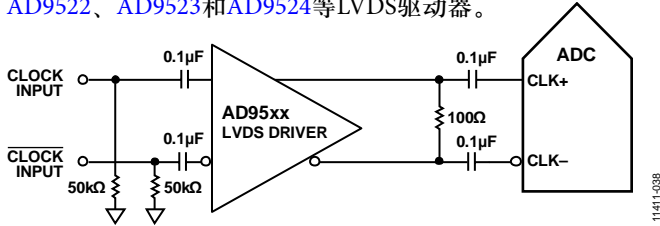
图38. 差分LVDS采样时钟(频率可达625 MHz)
