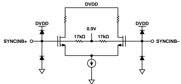
图25. 等效SYNCINB±输入电路
