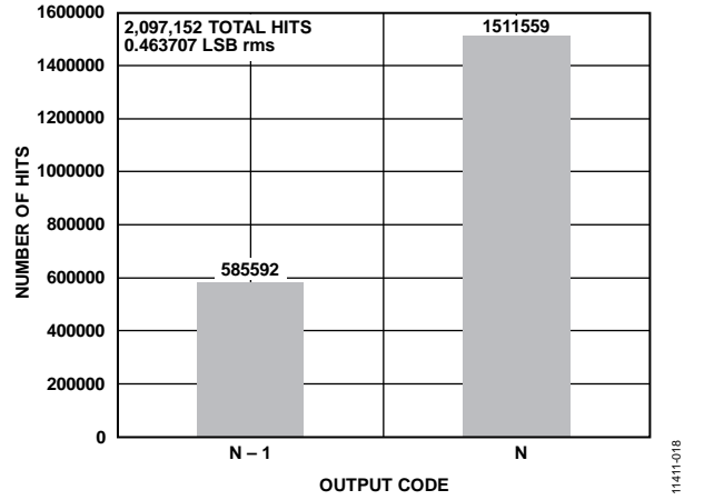
图18. 接地输入直方图
