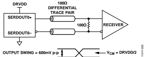
图55. 直流耦合数字输出端接示例
