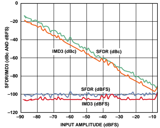
图13. 双音SFDR/IMD3与输入幅度( A_{IN} )的关系 ( f_{IN1} = 89.12 MHz, f_{IN2} = 92.12 MHz)
