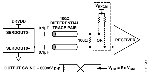
图54. 交流耦合数字输出端接示例
