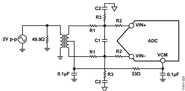
图31. 差分变压器耦合配置
