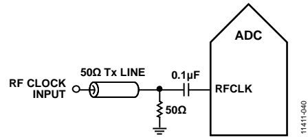
图40. 典型RF时钟输入电路
