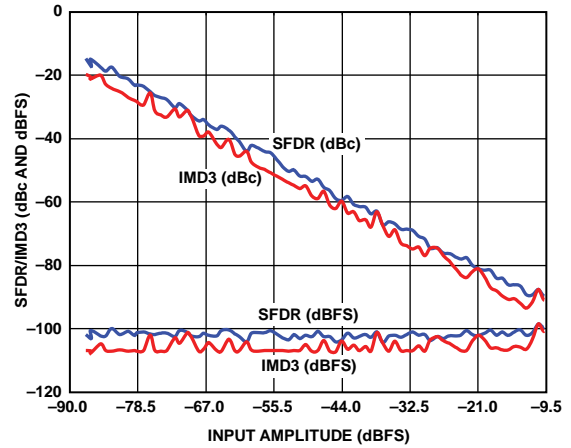
图14. 双音SFDR/IMD3与输入幅度( A_{IN} )的关系 ( f_{IN1} = 184.12 MHz, f_{IN2} = 187.12 MHz)
