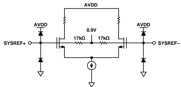
图26. 等效SYSREF±输入电路
