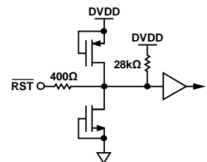
图27. 等效RST输入电路
