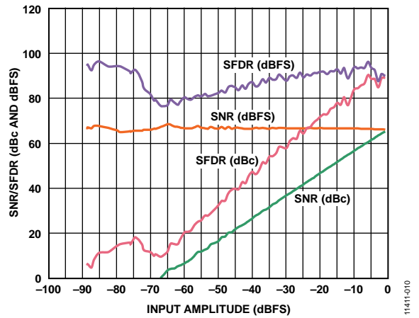
图10. 单音SNR/SFDR与输入幅度( A_{IN} )的关系( f_{IN} = 185.1\text{ MHz} )
