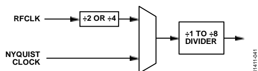
图42. AD6677时钟分频器电路
