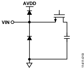
图19. 等效模拟输入电路
