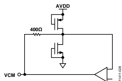
图28. 等效VCM电路
