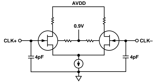
图34. 等效奈奎斯特时钟输入电路
