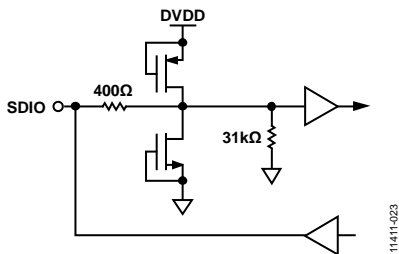
图23. 等效SDIO电路
