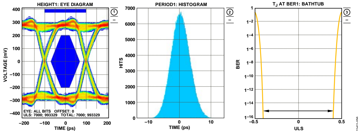
图56. AD6677数字输出数据眼图、直方图和浴盆图(5 Gbps时外部端接电阻为100 \Omega )
