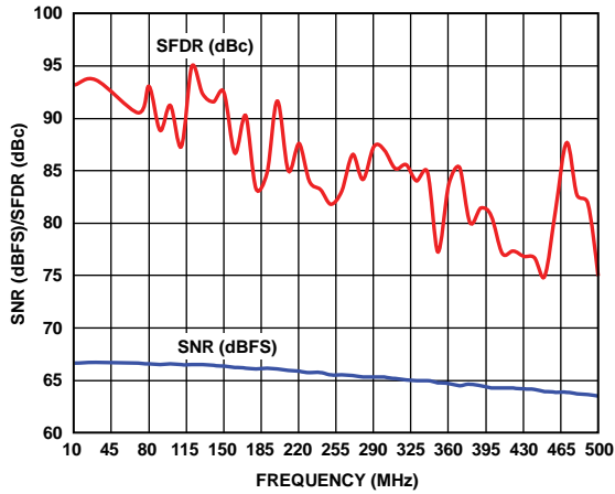
图11. 单音SNR/SFDR与输入频率( f_{IN} )的关系
