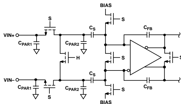
图29. 开关电容输入
