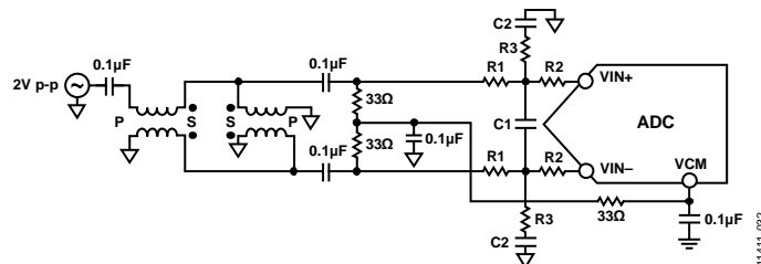
图32. 差分双巴伦输入配置
