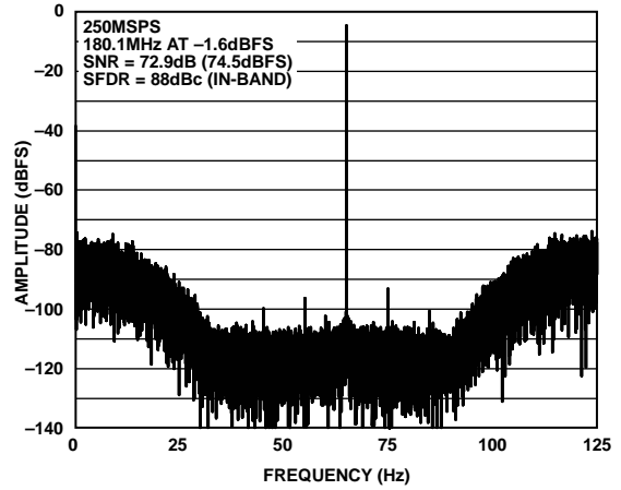
图46. 22%带宽模式，调谐字 = 28( f_s/4 调谐)
