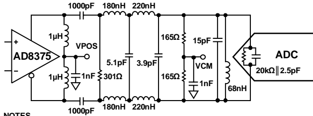
图33. 利用AD8375进行差分输入配置
