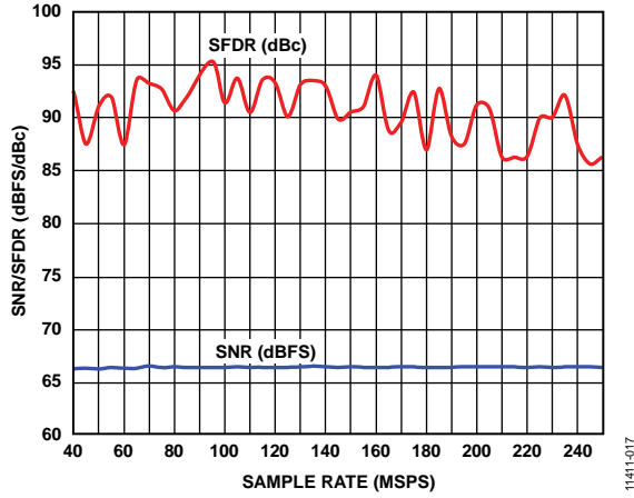
图17. 单音SNR/SFDR与采样速率( f_s )的关系( f_{IN} = 90.1 MHz)
