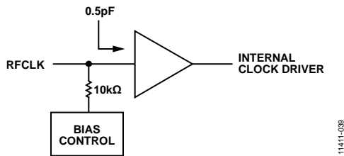
图39. 等效RF时钟输入电路
