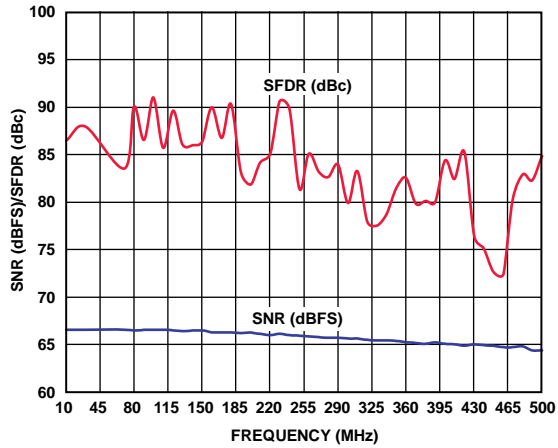
图12. 单音SNR/SFDR与输入频率( f_{IN} )的关系(RFCLK = 1.0 GHz, 4分频(地址0x09 = 0x21))
