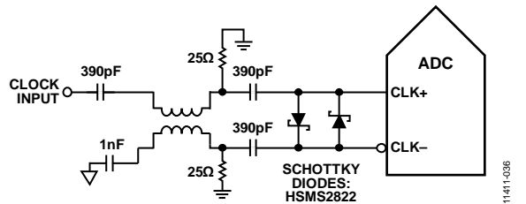
图36. 巴伦耦合差分时钟(频率可达625 MHz)
