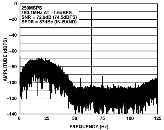
图47. 22%带宽模式，调谐字 = 41
