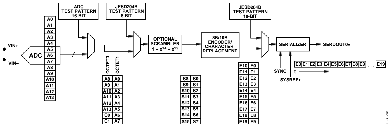
图52. JESD204B通道的数字处理
