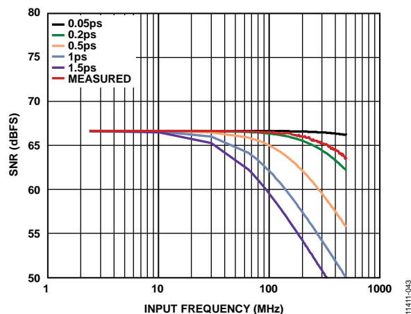
图43. 信噪比与输入频率和抖动的关系
