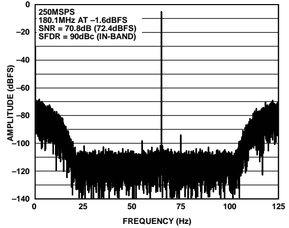
图49. 33%带宽模式, 调谐字 = 17( f_1/4 调谐)
