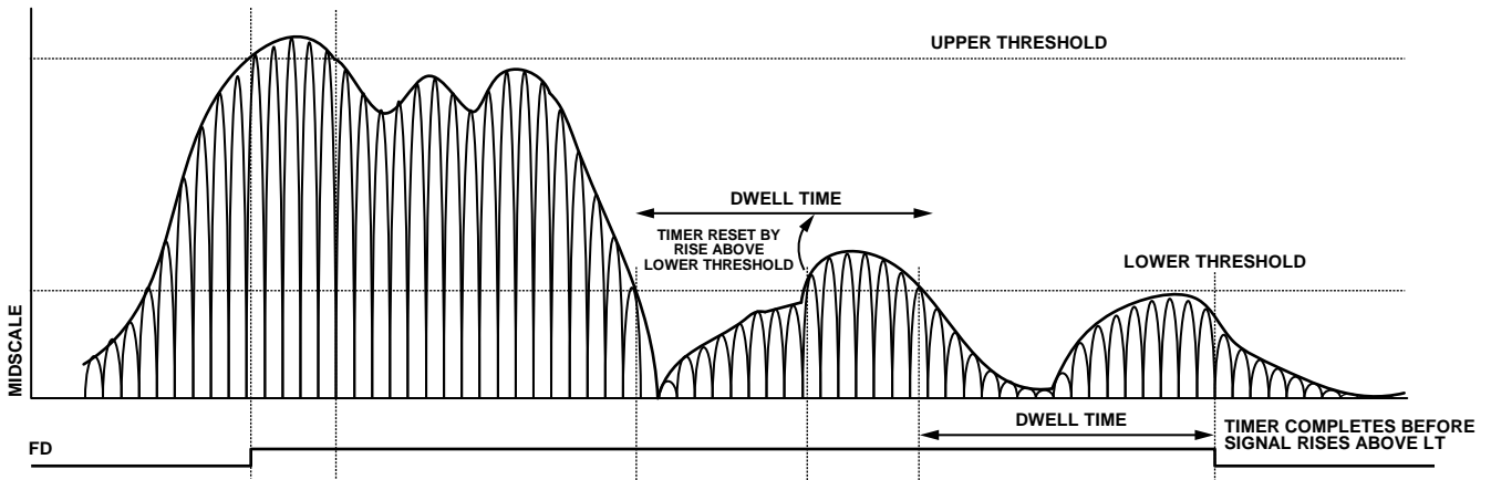
图57. FD信号的阈值设置
