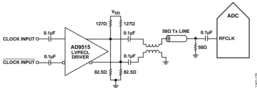
图41. 差分PECL RF时钟输入电路
