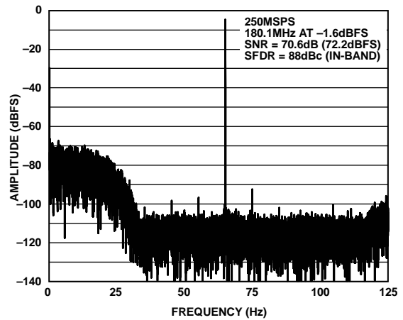
图50. 33%带宽模式, 调谐字 = 27
