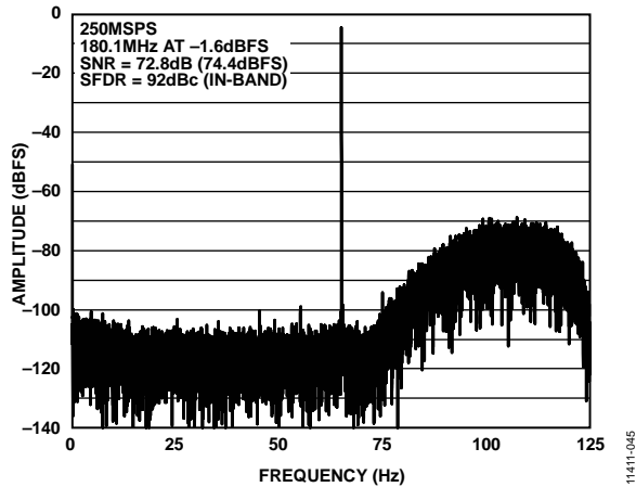
图45. 22%带宽模式，调谐字 = 13
