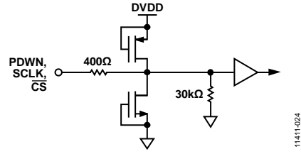
图24. 等效PDWN、SCLK或CS输入电路
