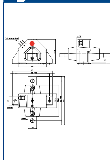
LA 255-T
