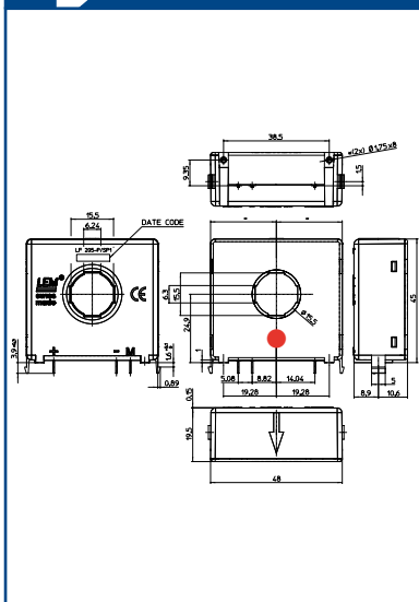
LF 205-P/SP1
