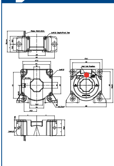
LF 305-S
