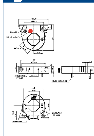
LF 306-S
