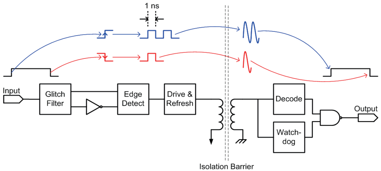
图 2. 一种数据传输方法是将边沿编码为单脉冲或双脉冲
