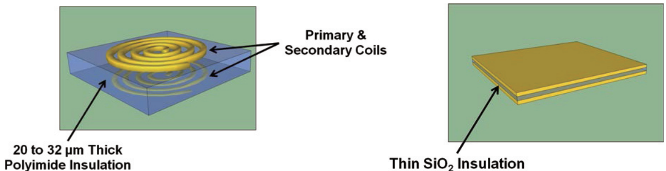
图 1. (a) 带厚聚酰亚胺绝缘层的变压器，电流脉冲产生磁场，在另一个线圈中感生电流； (b) 带薄 SiO 2 绝缘层的电容，利用低电流电场将数据耦合到隔离栅的另一端。
