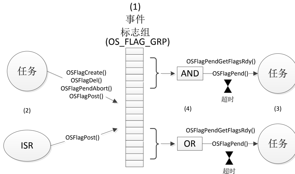
图 11.1.1 事件标志组
