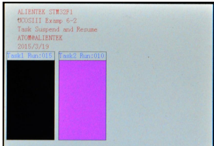
图 6.2.2 任务 2 恢复
