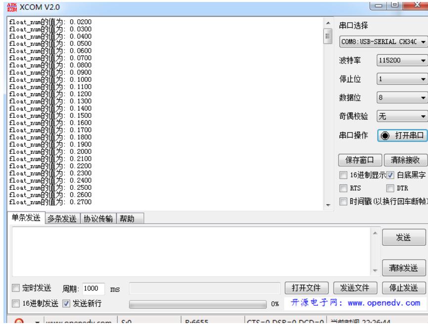
图 1.4.1 串口输出
