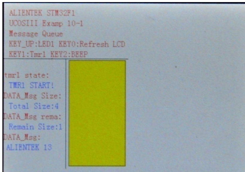
图 10.3.3 开启定时器 1
