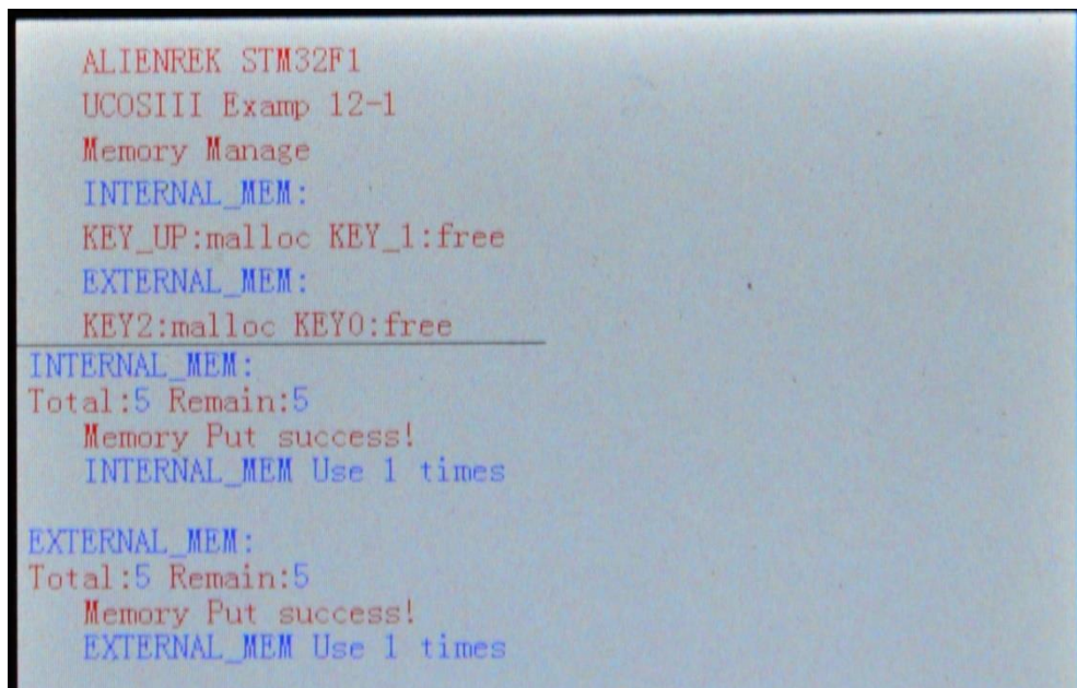
图 12.4.4 释放内存
